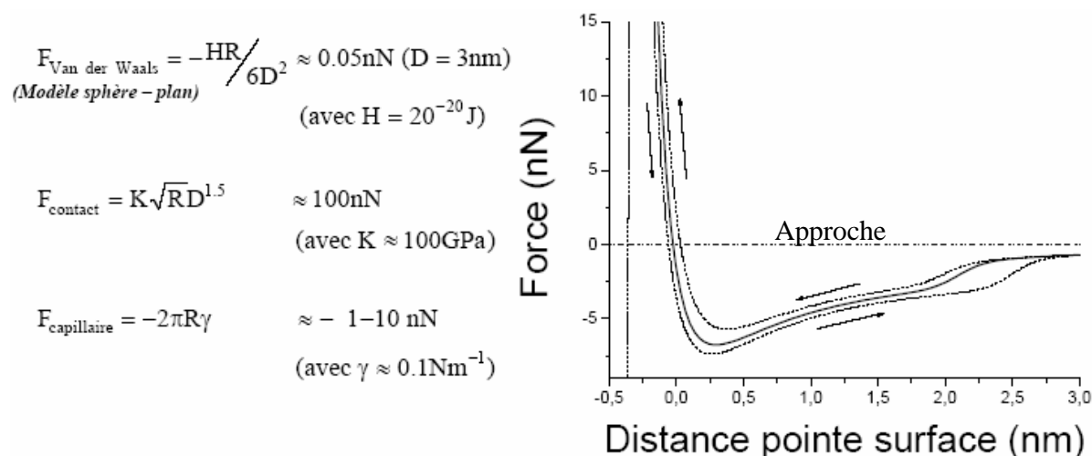
Figure B.4 : Interaction pointe-surface donnée par le potentiel de Lennard-Jones
