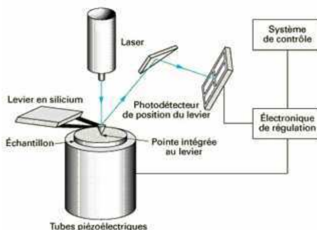
Figure B.3: Principe générale d'un microscope à force atomique standard
