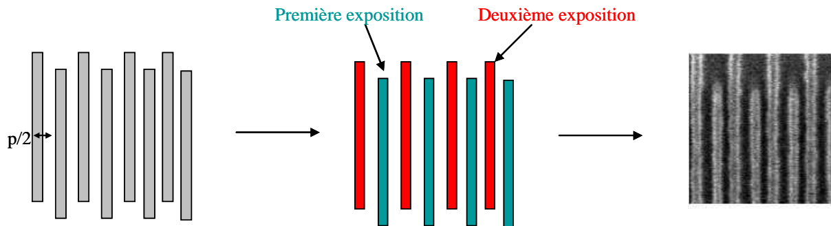
Figure 1.11 : Décomposition d'un réseau dense en étape d'exposition
