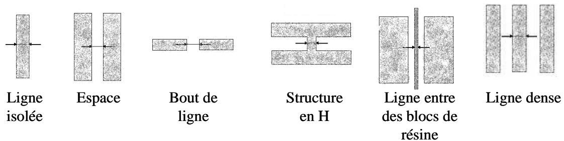
Figure 3.7: Types de structures utilisées
