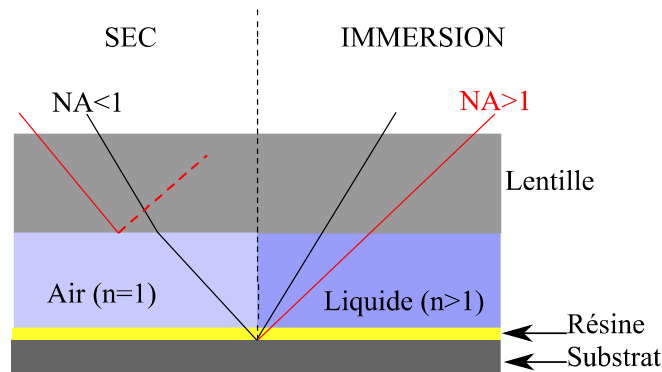
Figure 1.9 : Comparaison entre un système de lithographie « sec » et un système à immersion
