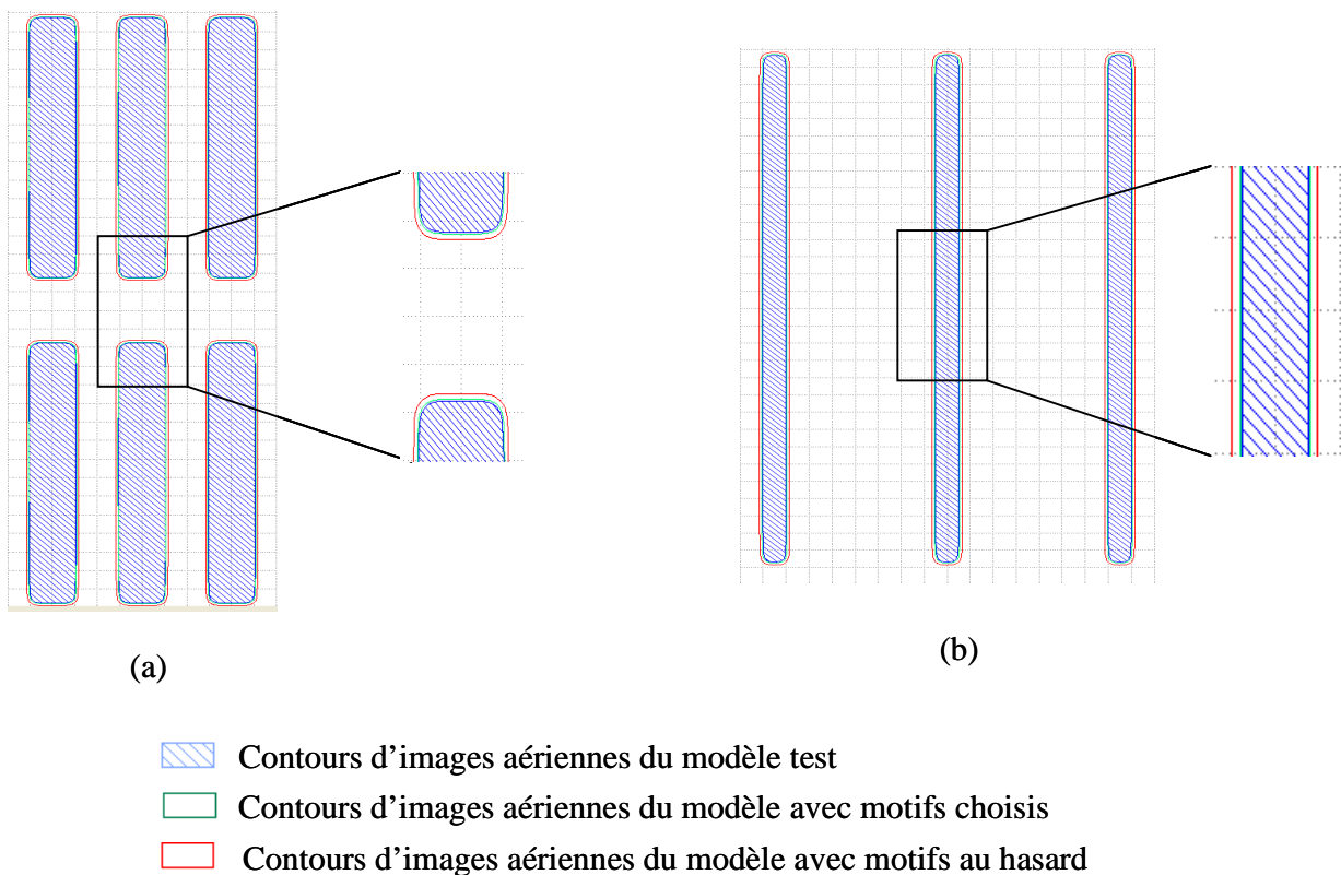
Figure 5.5 : Comparaison à condition nominale des contours des trois modèles créés avec tous les motifs, les motifs choisis et les motifs tiré au hasard, pour un motif de type ligne(a) et un motif bout de ligne(b)
