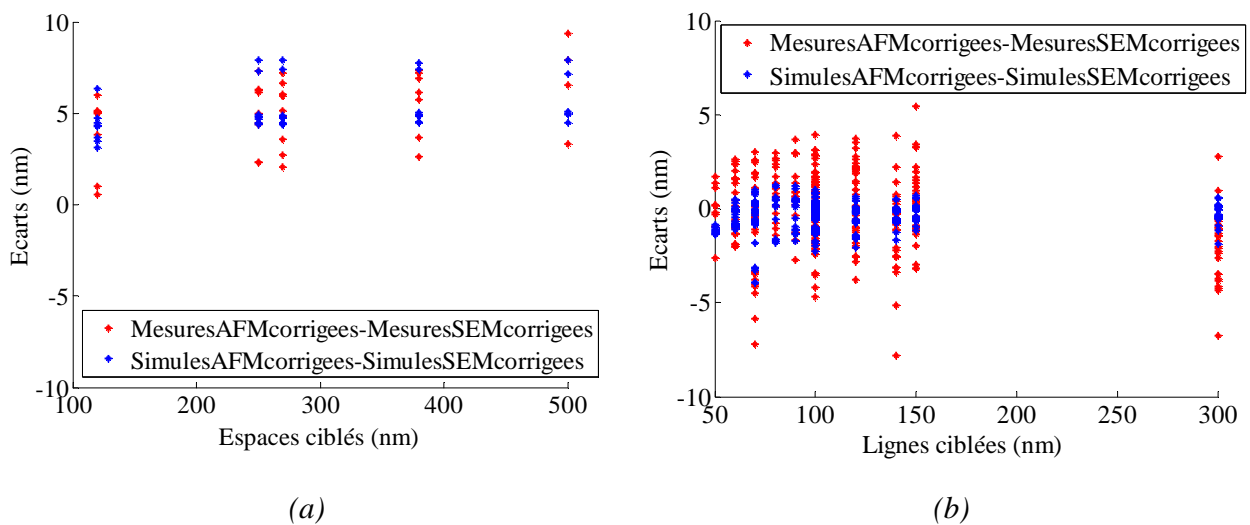
Figure 4.21 : Comparaison entre les écarts de mesures et résultats du modèle de référence par rapport au modèles calibré avec les mesures brutes provenant de la métrologie SEM, dans le cas des mesures lignes (a) et dans le cas des espaces isolés (b)
