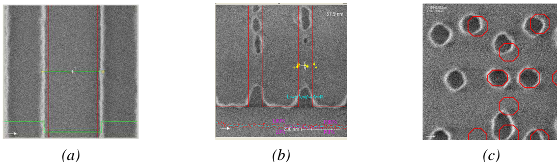
Figure 3.1 : Exemple de mauvaises mesures trouvées dans un ensemble de calibrage de modèle OPC
