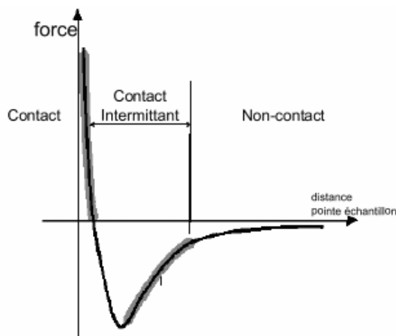
Figure B.5: Domaine d'interaction des différents modes de fonctionnement de l'AFM à l'aide d'un potentiel de Lennard-Jones
