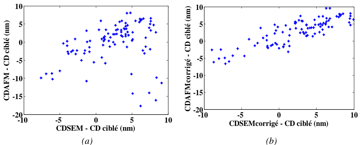
Figure 4.17 : Graphe de corrélation des écarts de mesures AFM et SEM par rapport à la mesure ciblée pour les motifs lignes denses brutes (a) et après correction (b)
