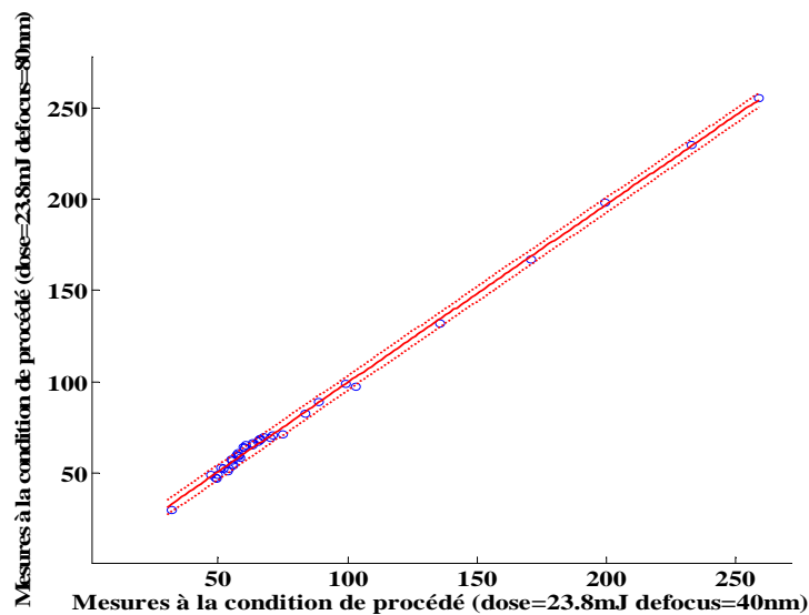
Figure 3.11 : Droite de régression et intervalle de confiance des dimensions critiques des motifs mesurées entre deux conditions de procédé
