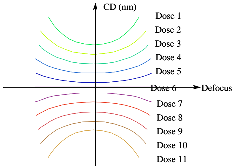
Figure 1.7 : Allure d'une courbe de Bossung
