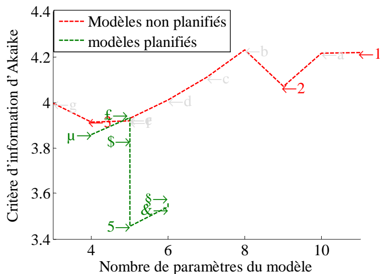
Figure 6.8: Comparaison du résultat du critère d'information d'Akaike entre les modèles créés avec des paramètres choisis au hasard sur la courbe rouge et ceux créés avec les paramètres influents du modèle donné par le plan d'expérience
