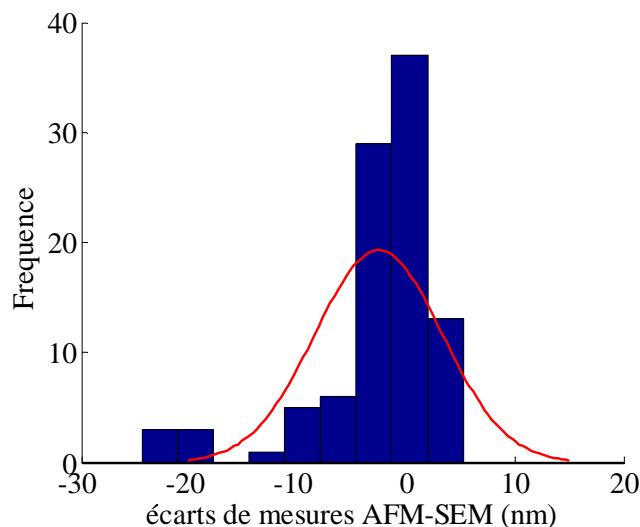
Figure 4.9 : Histogramme des écarts les mesures faites avec les métrologies AFM et SEM dans le cas des motifs « ligne dense »
