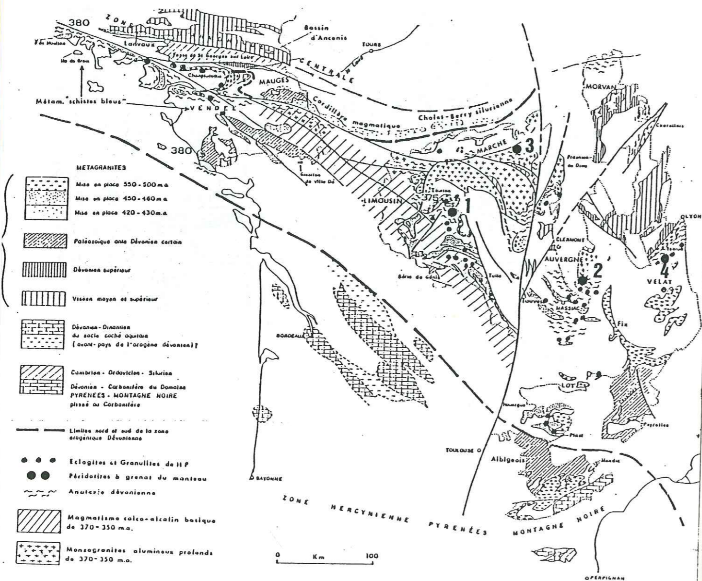
Fig. 9 - Localisation des péridotites à grenat mantelliques dans le Massif Central Français [d'après AUTRAN & COGNE, 1980]: 1 - Le massif de l'Artige, 2 - Le massif des Courtilles (rajouté), 3 - Le massif d'Auges et 4 - Les Monts du Lyonnais.
