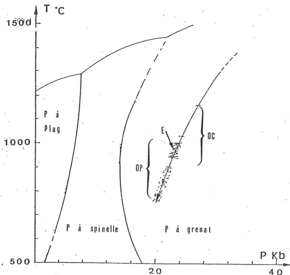
Fig. 142 - Trajectoires PT hypothétiques calculées pour les lherzolites à spinelle et grenat de l'Artige. (OP et OC): Champs des températures des porphyroclastes d'opx et de cpx; (E) Exsolution de cpx (ou de grenat ?) dans les porphyroclastes d'opx et (R) Zone de réajustement.
