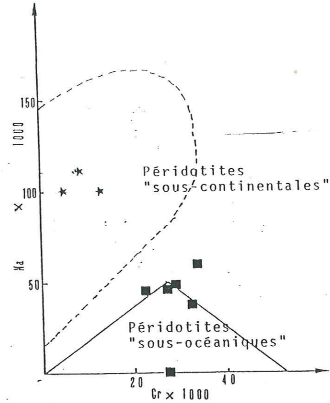
Fig. 85 - Différenciation des cpx des péridotites "sous-continentales" et des péridotites "sous-océaniques" d'après leur rapport Na/Cr selon KORNPROBST et al. [1981], appliquée aux cpx analysés ici.
