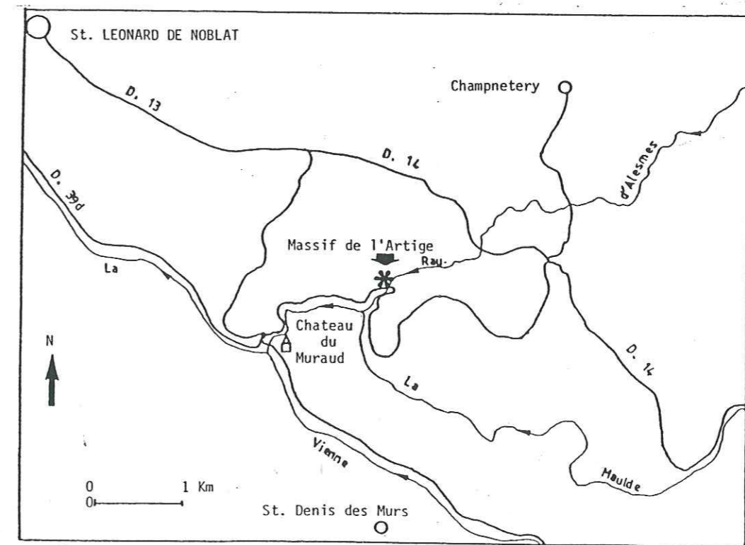
Fig. 20 - Localisation du massif ultrabasique de l'Artige, Haut-Limousin.
