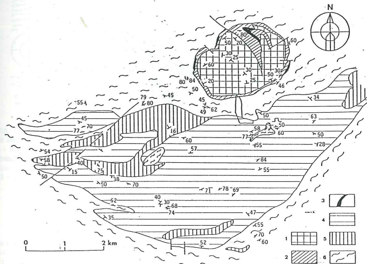
Fig. 5 - Carte géologique simplifiée du massif granitique de Bory [d'après MISAR et al., 1984]: 1 - Serpentinites; 2 - Amphibolites; 3 - Diallagites; 4 - Granulites contenant des inclusions de péridotites à grenat; 5 - Gneiss à biotite et sillimanite et 6 - Gneiss à cordiérite et migmatites.
