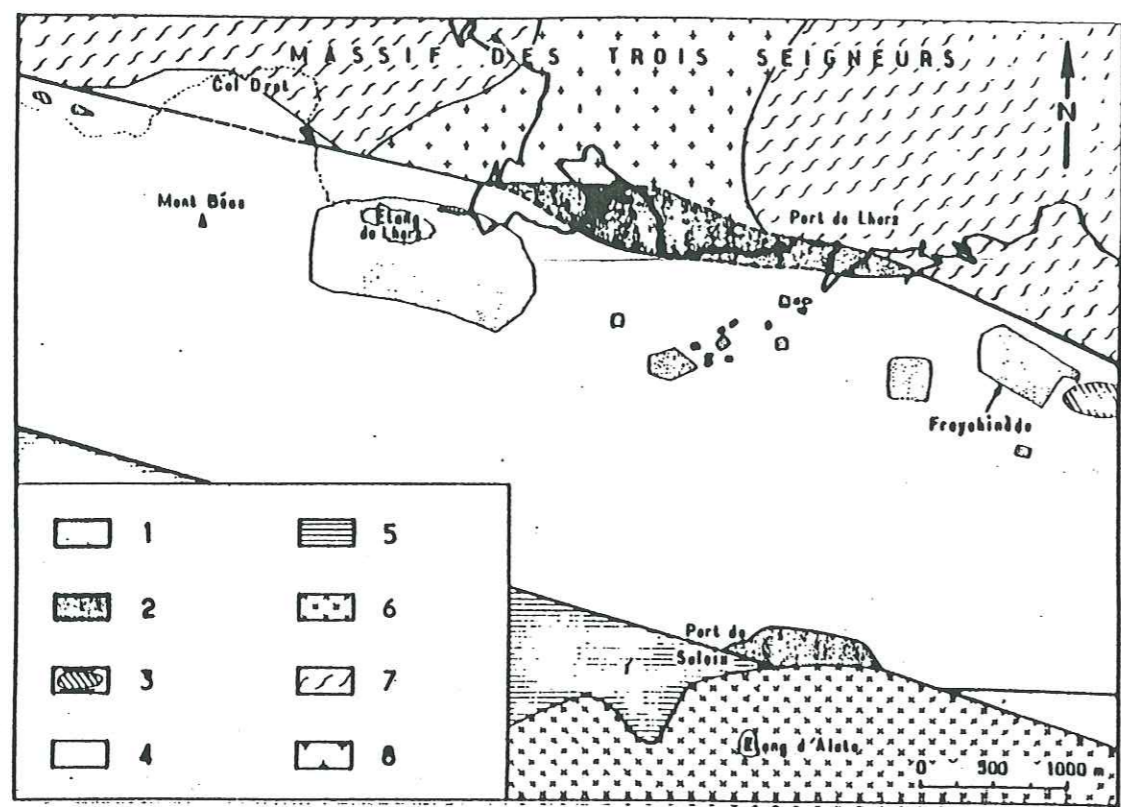
Fig. 13 - Situation des écaïlles lherzolitiques [d'après AZAMBRE & RAVIER, 1978]: 1 - Lherzolites; 2 - Formations granulitiques; 3 - Ophites; 4 - Terrains mésozoïques; 5 - Formations paléozoïques; 6 - Granites de Bassiès; 7 - Micaschistes et gneiss; 8 - Granodiorite [dans FABRIES & CONQUERE, 1984].
