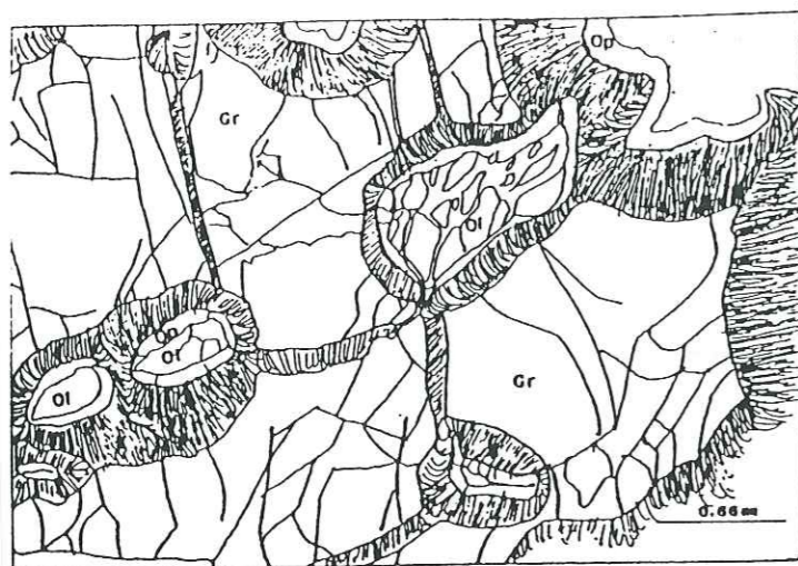
Fig. 31 - Porphyroclastes de grenat à inclusions d'olivine. La kélyphite se développe autour du grenat, dans les fractures et au contact des inclusions. Elle réagit avec l'olivine en donnant une auréole d'opx (Lame SCBF-10-10)
