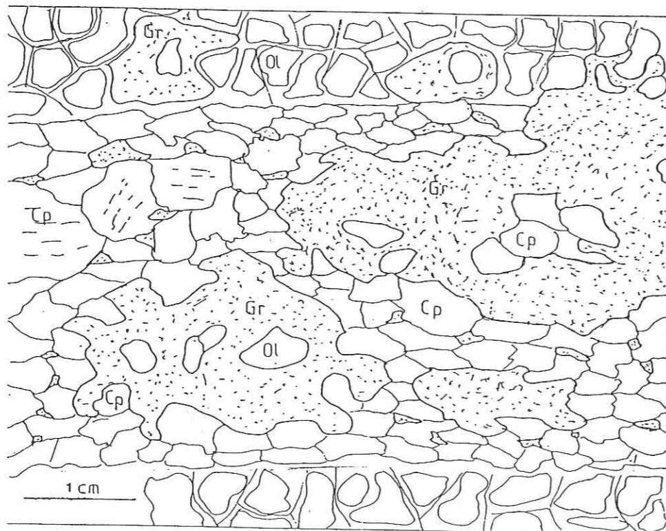
Fig. 40 - Texture d'un ruban de clinopyroxénolite à grenat associé aux métadunites à grenat et spinelle du Bois des Feuilles.
