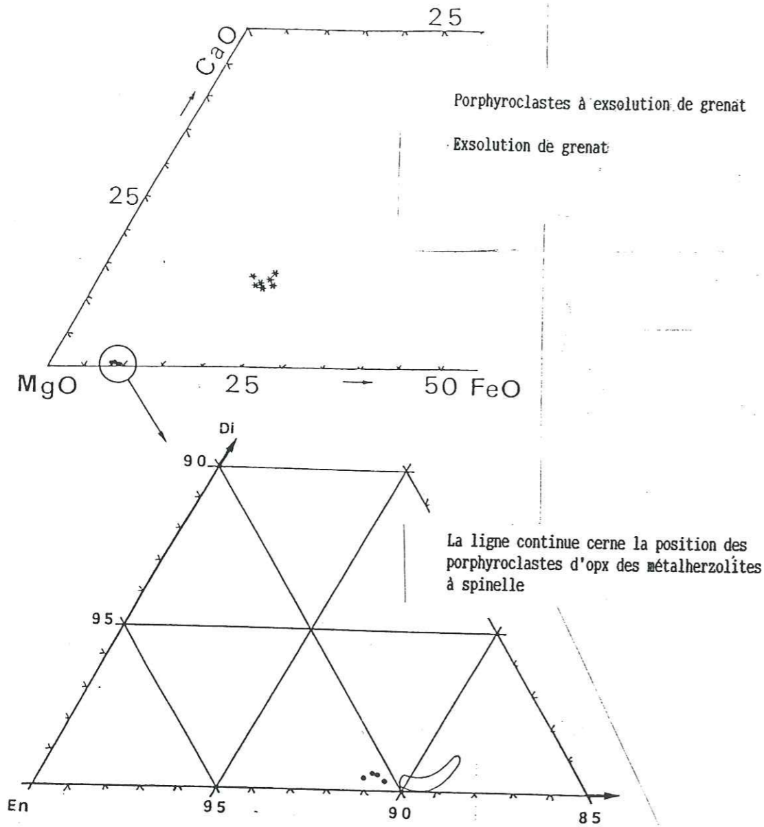
Fig. 77 - Position des porphyroclastes d'opx à exsolutions de grenat analysés dans le diagramme de Hess.
