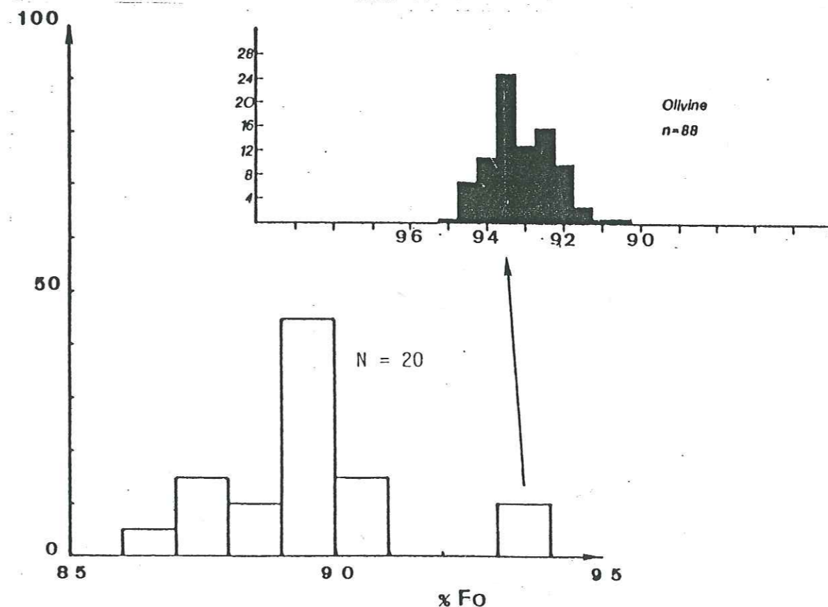
Fig. 90 - Pourcentage de forstérite contenu dans les deux types d'olivine analysés dans les métadunités à grenat et spinelle du Bois des Feuilles comparé avec celui des inclusions d'olivine rencontrées dans les diamants par MEYER [1982].
