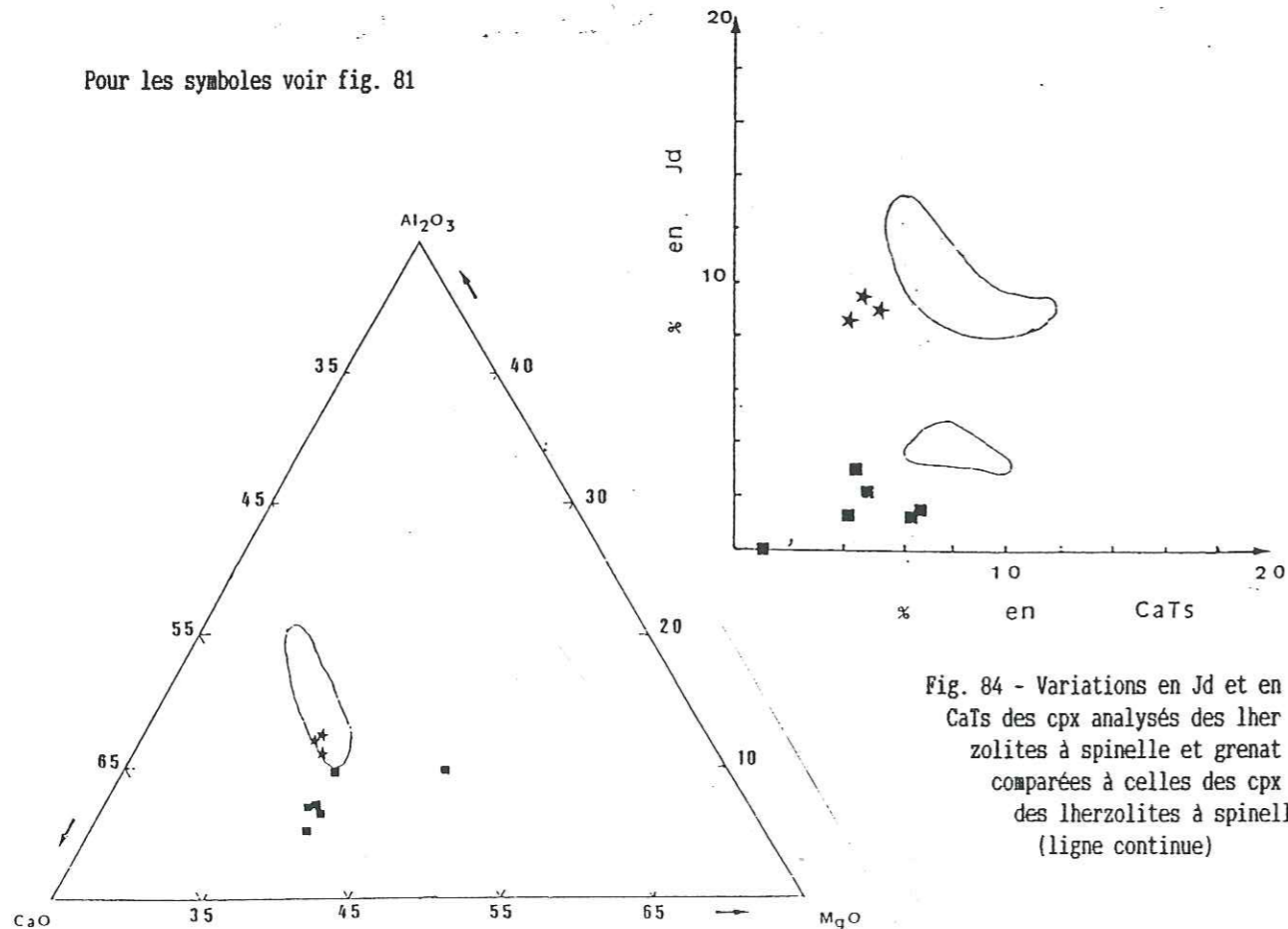
Fig. 83 - Variations en MgO, CaO et Al 2 O 3 des cpx des lherzolites à spinelle et grenat comparées à celles des cpx des lherzolites à spinelle
