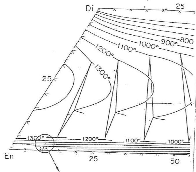
Fig. 97 - Comparaison des compositions des différents types d'opx analysés dans les métalherzolites à spinelle de Chagnon avec ceux du Bois des Feuilles (zone limitée par des tirets). Les relations de phases sont celles de LINDSLEY [1983] pour 10 Kb.
