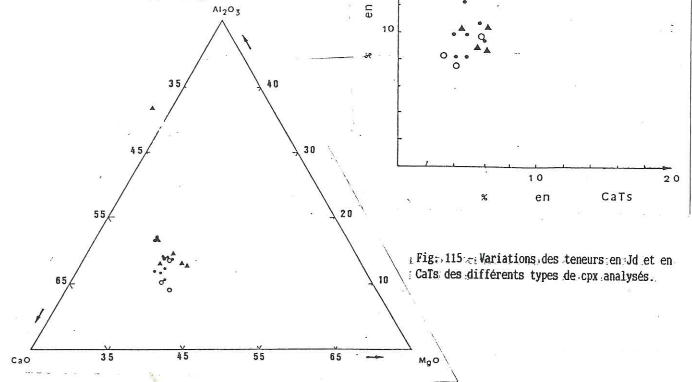
Fig. 114 - Variations en MgO, Al 2 O 3 et CaO dans les cpx analysés dans les rubans pyroxénolitiques de Chagnon.
