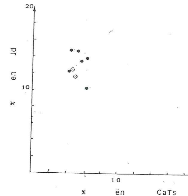
Fig. 135 - variations des teneurs en Jd. et en CaTs des cristaux de cpx analysés.
