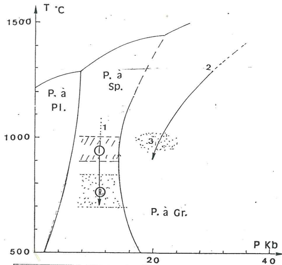
Fig. 96 - Chemins thermobarométriques hypothétiques des métaherzolites à spinelle (1), des métaherzolites à spinelle et grenat (2) et des métadunités à grenat et spinelle (3) rencontrées au Bois des Feuilles déduits de l'examen des principales phases. Pour le chemins (1) 'I' indique l'intervalle de T obtenus pour les inclusions et 'R' pour les cristaux de recuit. L'intervalle des porphyroclastes est intermédiaire. [Diagramme de phases de GASPARIK, 1984].
