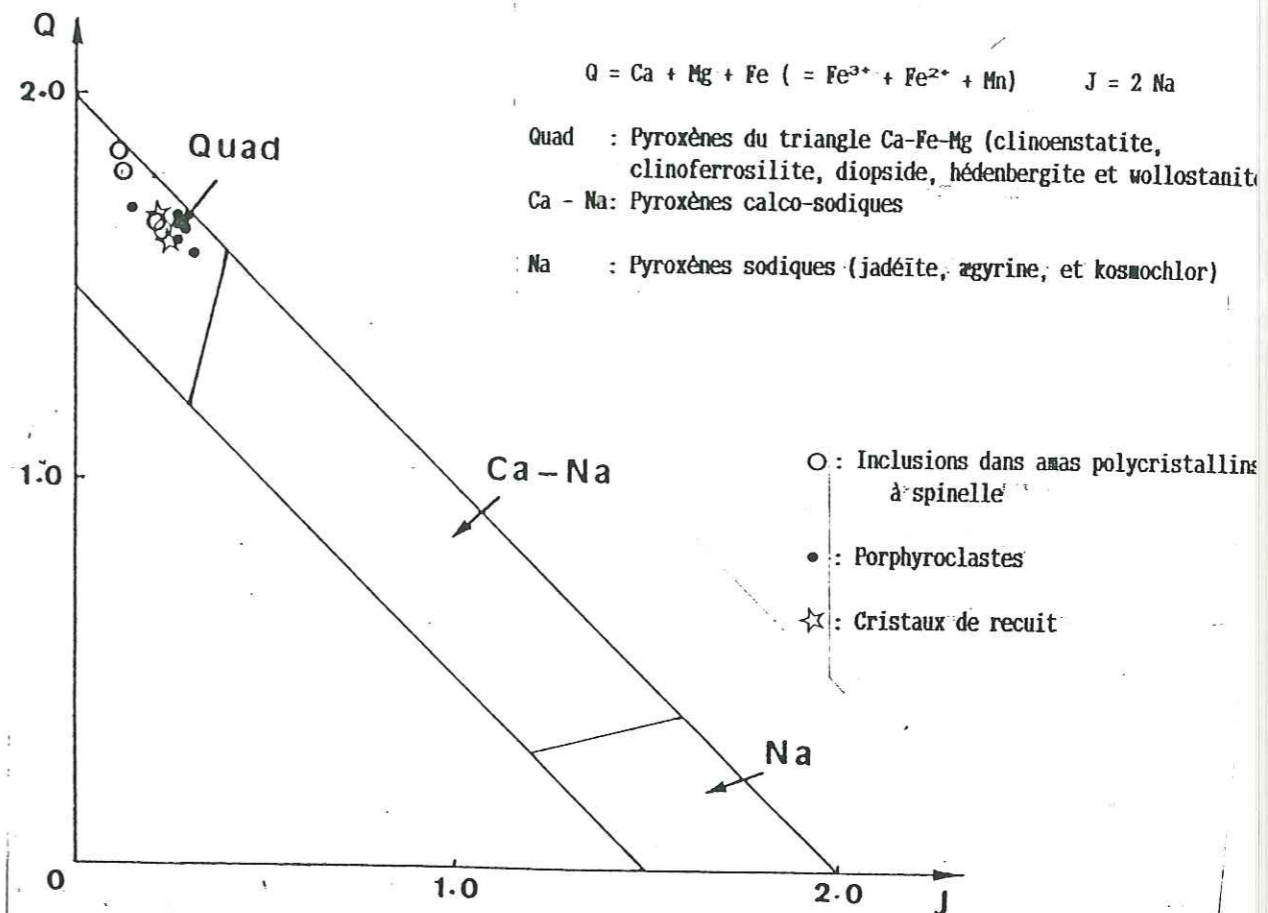
Fig. 70 - Positions des trois types de cpx analysés dans les lherzolites à spinelle du Bois des Feuilles dans le diagramme Q - J qui permet de différencier les pyroxènes à tendance sodiques et autres [MORIMOTO, 1988].
