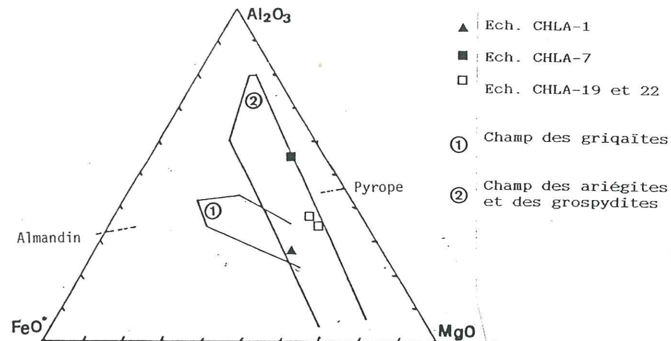
Fig. 55 - Position de quatre analyses de pyroxénolites à grenat de Chagnon dans le diagramme Al-F-M de MOUKADIRI & KORNPROBST [1984] et KORNPROBST et al. [1987]. FeO* = FeO + MgO
