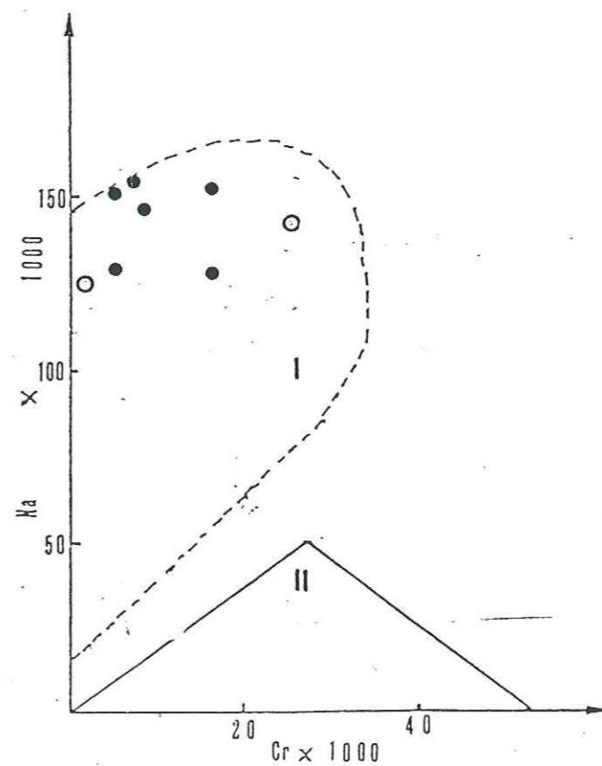
Fig. 136 - Différenciation des cpx des péridotites "sous-continentales" (I) et des péridotites "sous-océaniques" (II) d'après leurs rapports Na/Cr selon KORNPROBST et al. [1981] appliquée aux cristaux de cpx analysés
