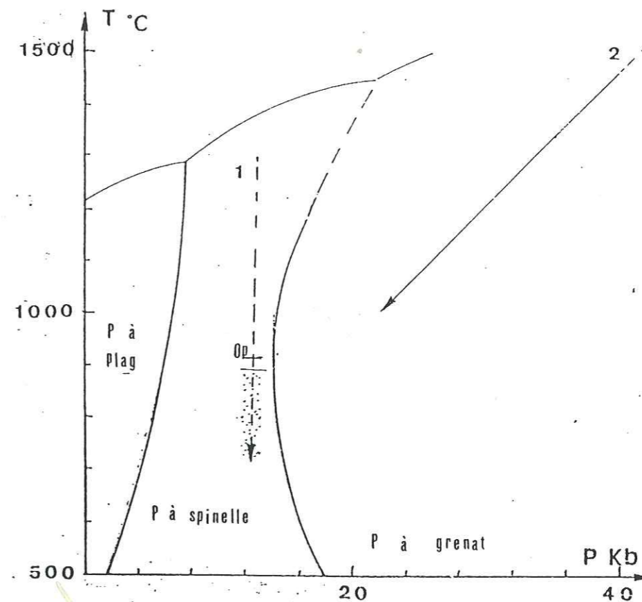
1: LHERZOLITES A SPINELLE Op: T Max. obtenue pour les porphyroclastes d'opx, d'olivine et de spinelle Zone du dernier rééquilibrage 2: CRISTAL D'OPX DE BORDURE D'UN RUBAN PYROXENOLITIQUE A GRENAT
