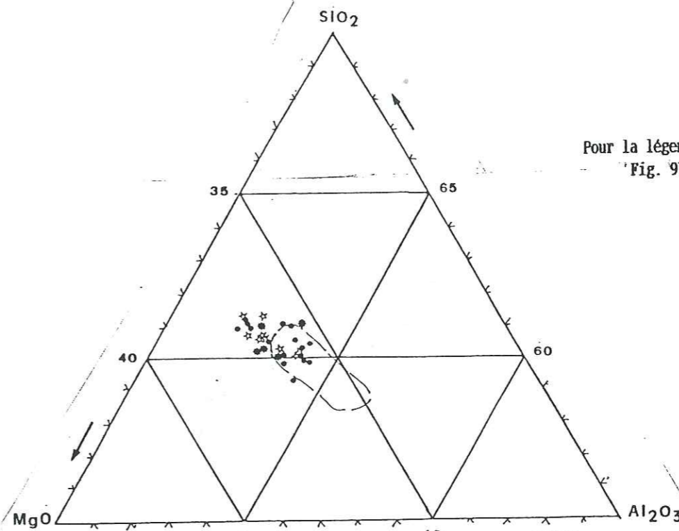
Fig. 99 - Comparaison des variations en SiO 2 , Al 2 O 3 et MgO des différents types d'opx analysés dans les métalherzolites à spinelle de Chagnon et du Bois des Feuilles (zone limitée par des tirets).
