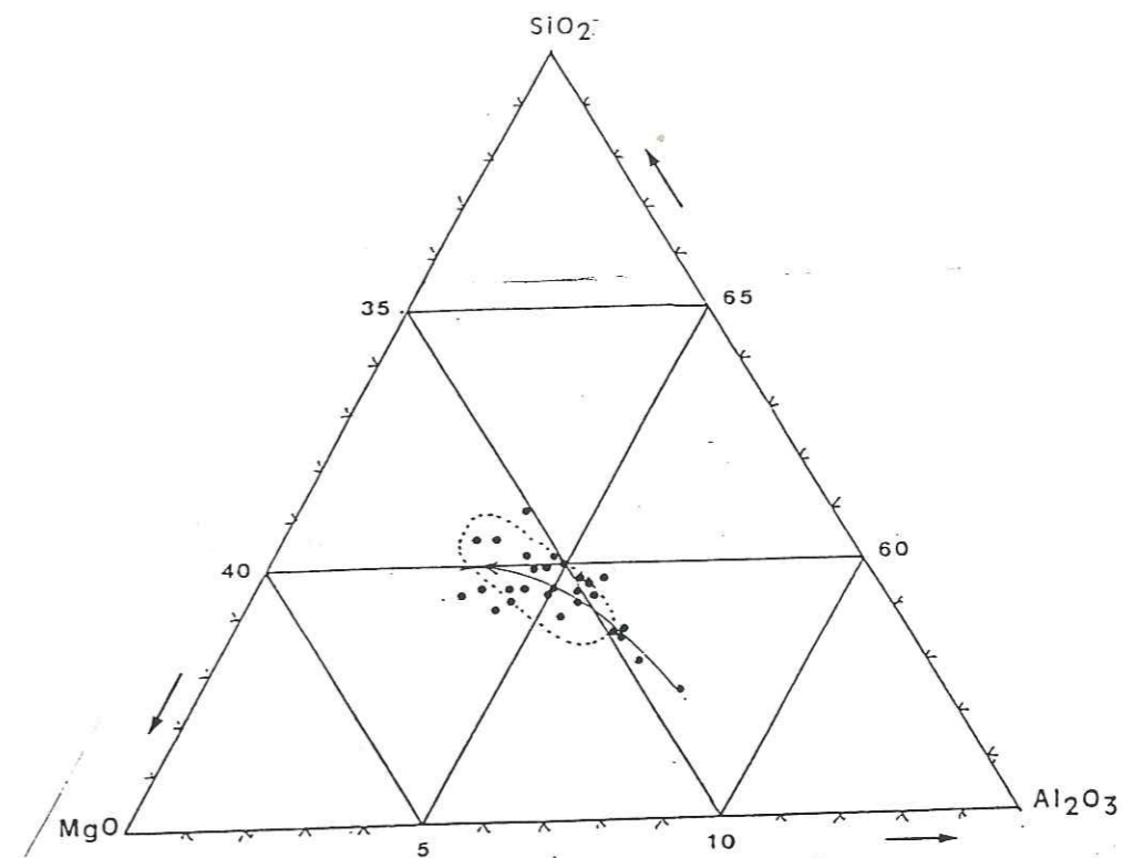
Fig. 122 - Variations en SiO 2 , Al 2 O 3 et MgO des porphyroclastes d'opx analysés à la microsonde dans les lherzolites à spinelle et grenat de l'Artige. Comparaison avec les opx des lherzolites à spinelle du Bois des Feuilles limitées par des pointillés.
