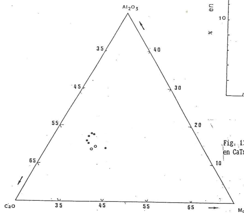
Fig. 134 - Variations en MgO, Al 2 O 3 et CaO dans les cristaux de cpx analysés dans les pyroxénolites de l'Artige.
