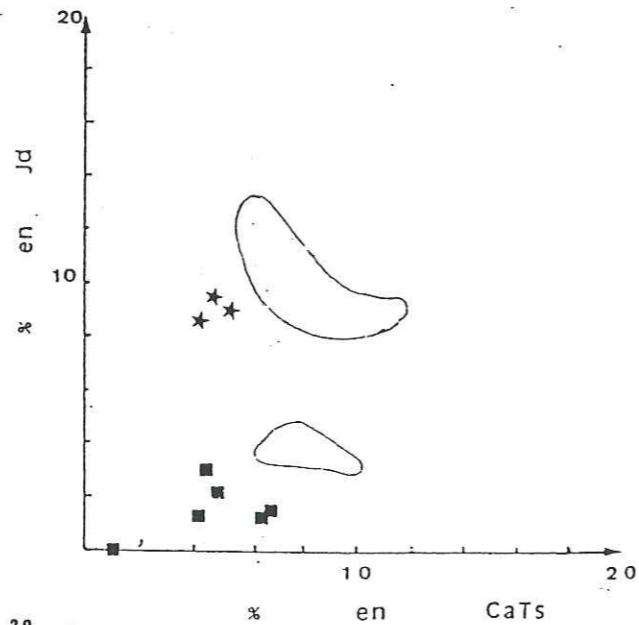
Fig. 84 - Variations en Jd et en CaTs des cpx analysés des lherzolites à spinelle et grenat comparées à celles des cpx des lherzolites à spinelle (ligne continue)
