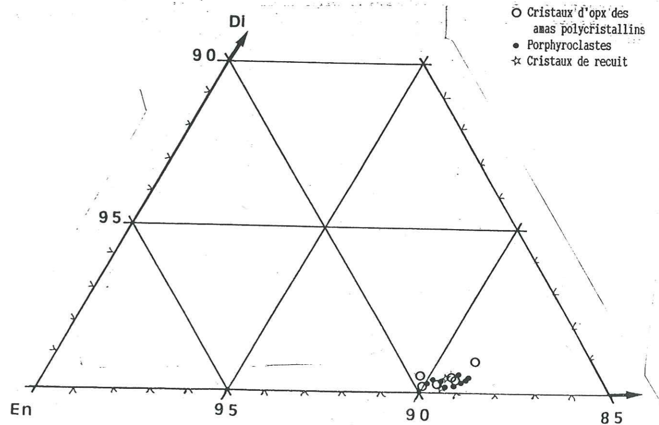
Fig. 67 - Même chose que la fig. 66 à échelle réduite.
