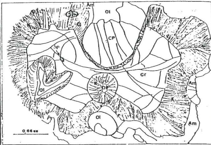
Fig. 32 - Même chose que la fig. 29, avec des inclusions de spinelle et de cpx. Vers l'extérieur la kélyphite recrystallise en amphiboles.
