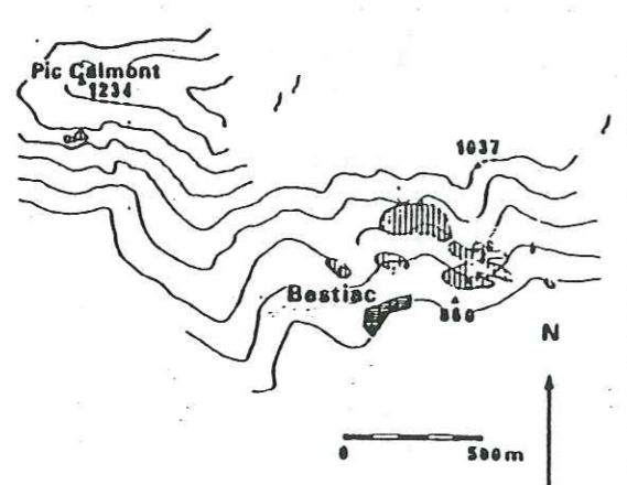
Fig. 13 - Situation des écaïlles lherzolitiques [d'après AZAMBRE & RAVIER, 1978]: 1 - Lherzolites; 2 - Formations granulitiques; 3 - Ophites; 4 - Terrains mésozoïques; 5 - Formations paléozoïques; 6 - Granites de Bassiès; 7 - Micaschistes et gneiss; 8 - Granodiorite [dans FABRIES & CONQUERE, 1984].
