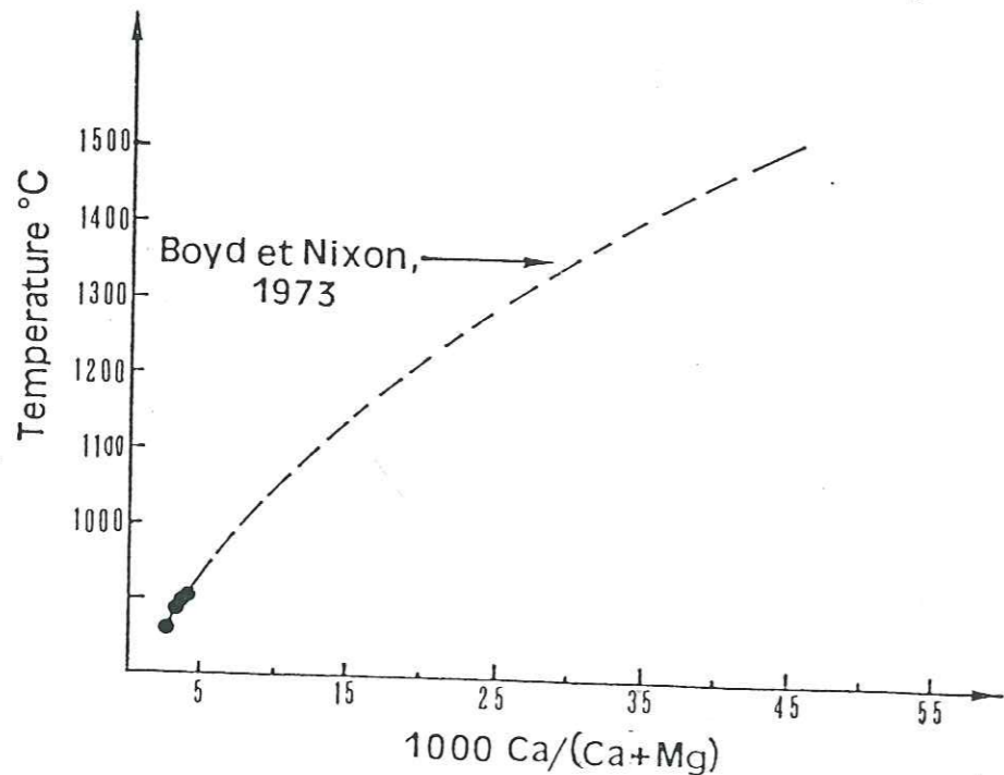
Fig. 78 - Géothermomètre de BOYD & NIXON [1973] appliqué aux porphyroclastes d'opx à exsolution de grenat analysés des métalherzolites à spinelle et grenat du Bois des Feuilles.
