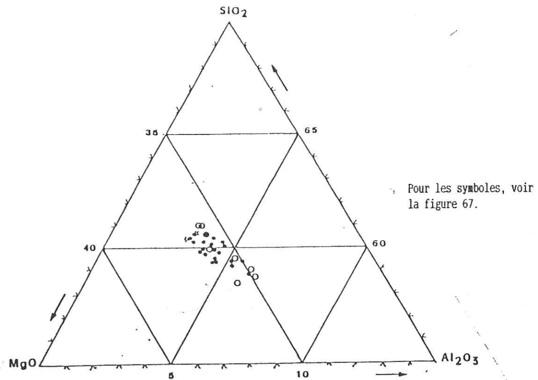
Fig. 68 - Variations des teneurs en SiO 2 , Al 2 O 3 et MgO des différents types d'opx analysés des métalherzolites à spinelle du Bois des Feuilles. Ces variations attestent une évolution entre des termes alumineux (amas polycristallins) et des termes plus siliceux et magnésiens (les cristaux de recuit).
