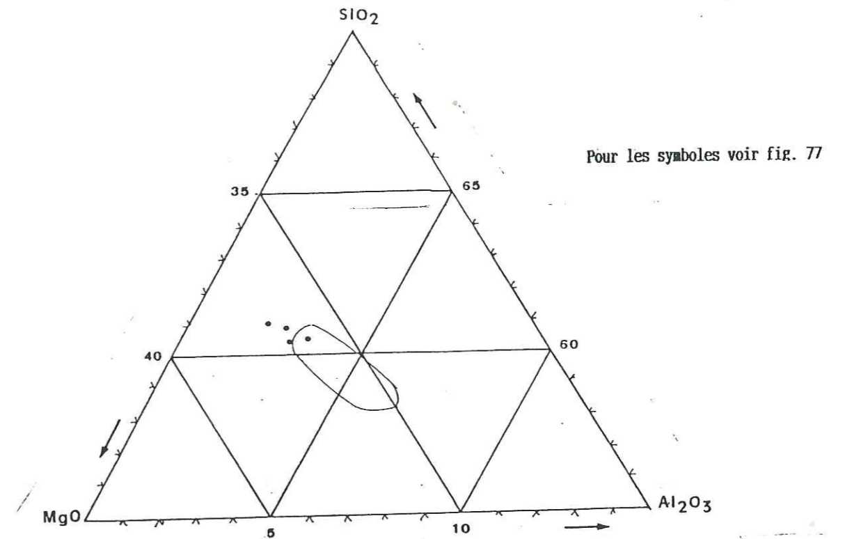
Fig. 79 - Variations des teneurs en SiO 2 , Al 2 O 3 et MgO des porphyroclastes à exsolutions de grenat comparées à celles des opx des métalherzolites à spinelle (ligne continue).
