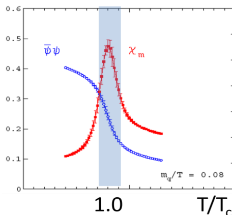
Figure 3 : Variation de la valeur moyenne des condensats de quarks en GeV en fonction de la température.
