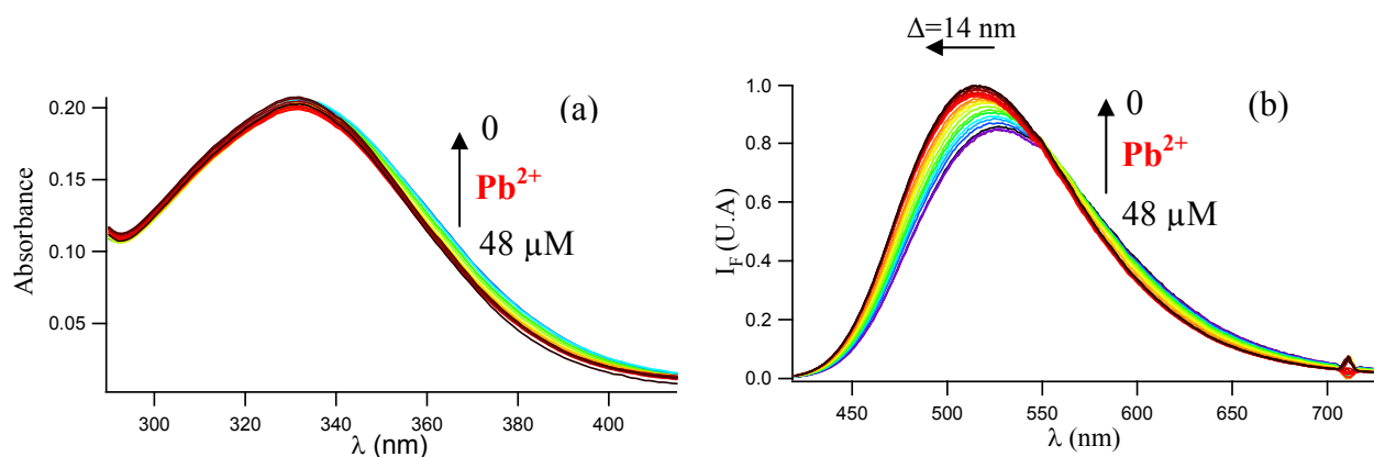
Figure IV-15 : Evolution des spectres d'absorption (figure a) et de fluorescence corrigée (figure b) ( \lambda_{\text{exc}} = 365 \text{ nm} ) du CalixDANS-3-OH, C = 1,71 \times 10^{-5} \text{ M} avec des ajouts croissants d'une solution de thiocyanate de plomb \text{pH} = 5,2 .
