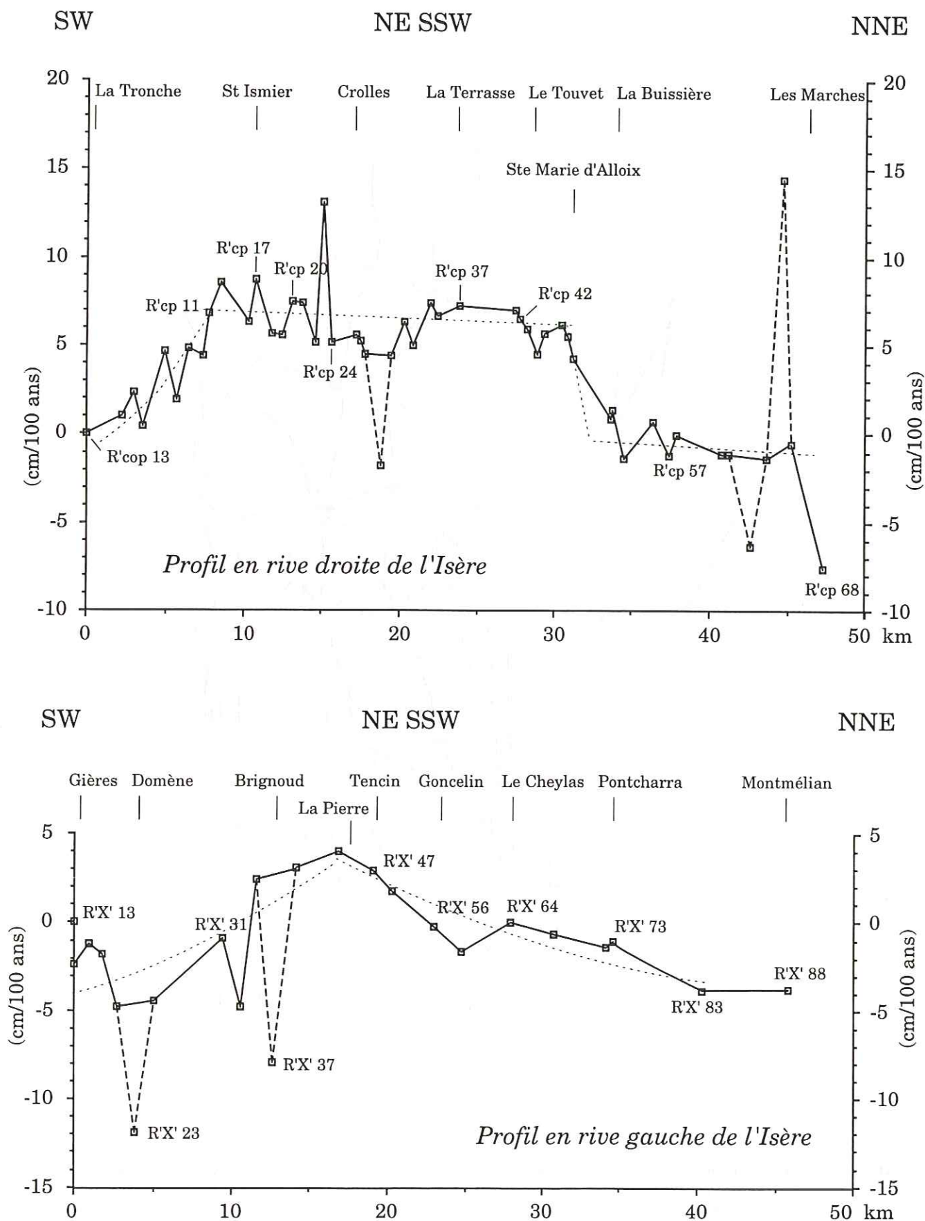
Fig. II-43. Comparaisons des nivellements effectués en 1950 et 1993 dans le Grésivaudan de part et d'autre de l'Isère. Profil de 1 er ordre R'X' en rive gauche; profil de 4 ème ordre de la maille R'c p3 en rive droite.
