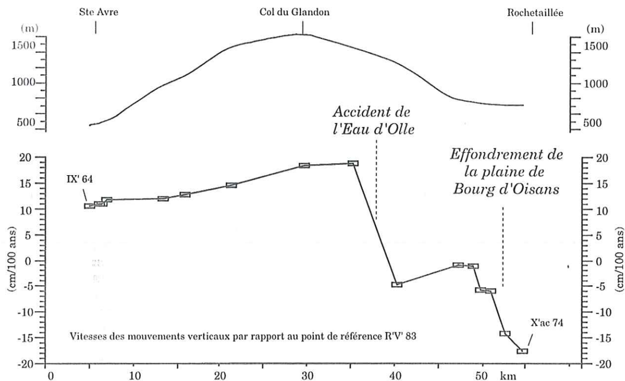
Fig. II-31. Comparaison de nivellements réalisés en 1903 et 1980, et topographie le long du profil de troisième ordre X' à km. (Extrémités du profil fixées par les valeurs calculées par la compensation de point de référence R'V' 83).
