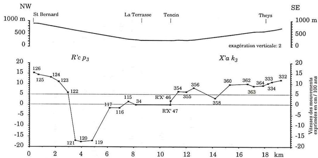
Fig. II-45. Profils de comparaison de nivellements en travers du Grésivaudan. Mesures effectuées en 1950 et 1993 sur des profils de 4 ème ordre dans les mailles X'a k_3 et R'c p_3 .
