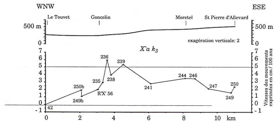
Fig. II-45. Profils de comparaison de nivellements en travers du Grésivaudan. Mesures effectuées en 1950 et 1993 sur des profils de 4 ème ordre dans les mailles X'a k_3 et R'c p_3 .
