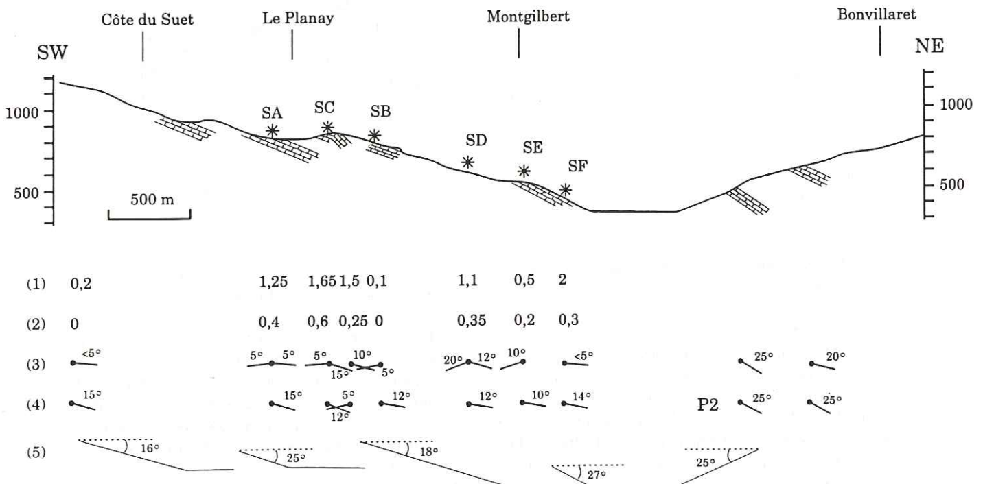
Fig. I-48. Étude morphostructurale de la colline de Montgilbert. (1): densité de fractures (par m); (2): ouverture des fractures (en cm/m); (3): plongement des pôles de fractures N120; (4): axes des plis; (5): pente topographique.
