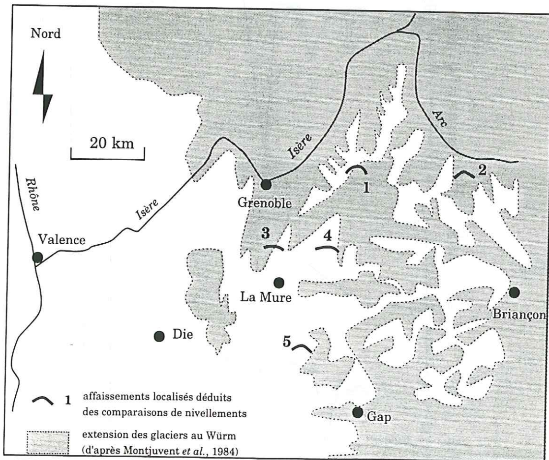
Fig. II-34. Localisation des principaux affaissements de la partie sud-est de la région étudiée et extension des glaciers au Würm.
