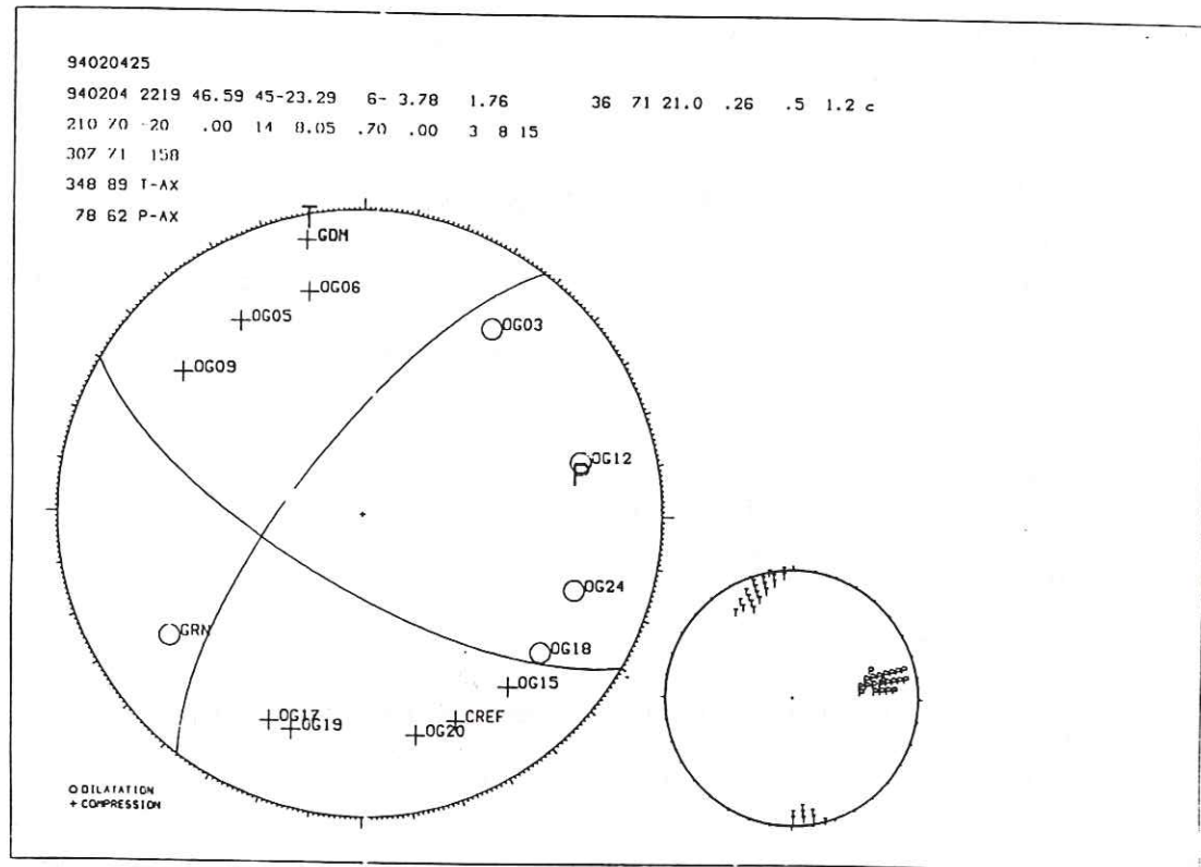
Fig. I-62. Mécanisme au foyer d'Allevard du 04/02/94 (d'après Thouvenot, 1994, communication personnelle). Magnitude: 2.1; profondeur: 1.76 km.
