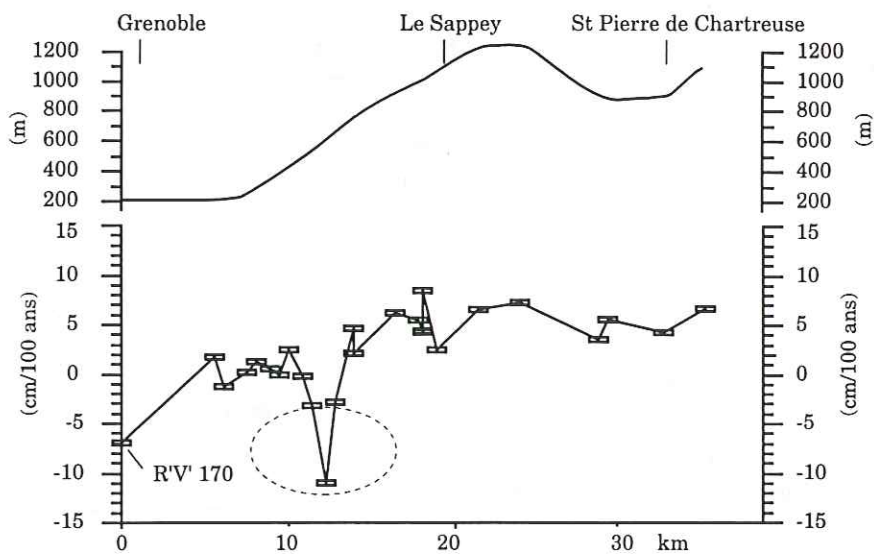
Fig. II-35. Mouvements de terrain mis en évidence par les comparaisons de nivellements.
