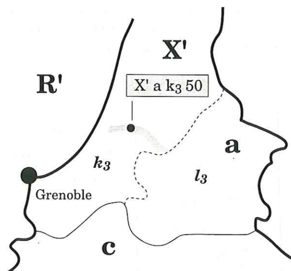
Fig. II-5. Désignation des repères de nivellement des 4 ordres de réseaux français.
