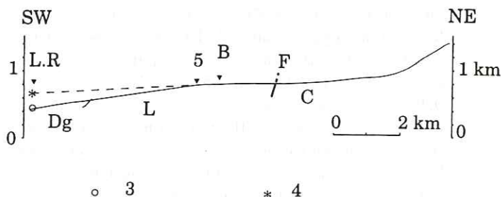
Fig. I-56. Marqueurs des mouvements verticaux sur les profils en long du Bréda, du Bens et du haut Gelon (exagération verticale: 2). 1: cours actuel; 2: paléo-cours; 3: niveau de base actuel; 4: ancien niveau de base; 5: rupture de pente correspondant à la limite supérieure atteinte par l'érosion régressive; 6: roll-over marqué dans la morphologie de la paléo-vallée en rive droite du Bréda; A: Allevard; Ar: Arvillard; B: Bourget en Huile; C: socle cristallin de Belledonne; D: Détrier; Dg: marno-calcaires du Dogger; F: faille (d'après la carte géologique au 1/50 000); L: Lias indifférencié; Lc: Lias calcaire; Ls: Lias schisteux; P: Pontcharra; R: La Rochette.
