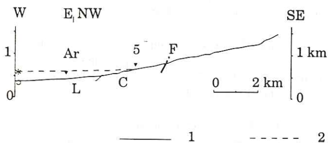
Fig. I-56. Marqueurs des mouvements verticaux sur les profils en long du Bréda, du Bens et du haut Gelon (exagération verticale: 2). 1: cours actuel; 2: paléo-cours; 3: niveau de base actuel; 4: ancien niveau de base; 5: rupture de pente correspondant à la limite supérieure atteinte par l'érosion régressive; 6: roll-over marqué dans la morphologie de la paléo-vallée en rive droite du Bréda; A: Allevard; Ar: Arvillard; B: Bourget en Huile; C: socle cristallin de Belledonne; D: Détrier; Dg: marno-calcaires du Dogger; F: faille (d'après la carte géologique au 1/50 000); L: Lias indifférencié; Lc: Lias calcaire; Ls: Lias schisteux; P: Pontcharra; R: La Rochette.
