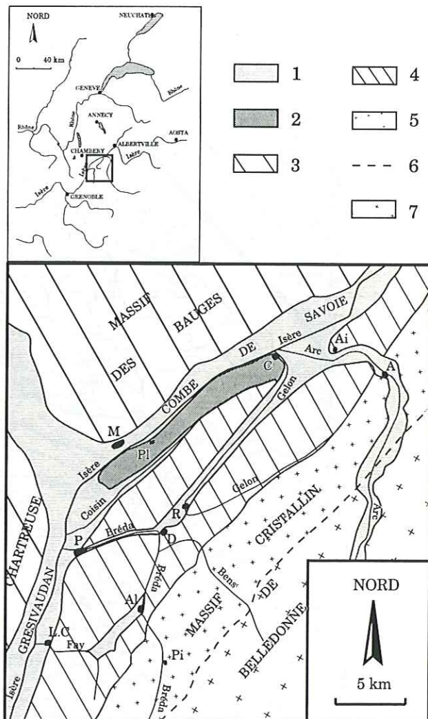
Fig. I-54. Cadre géographique et géologique de la zone étudiée.
