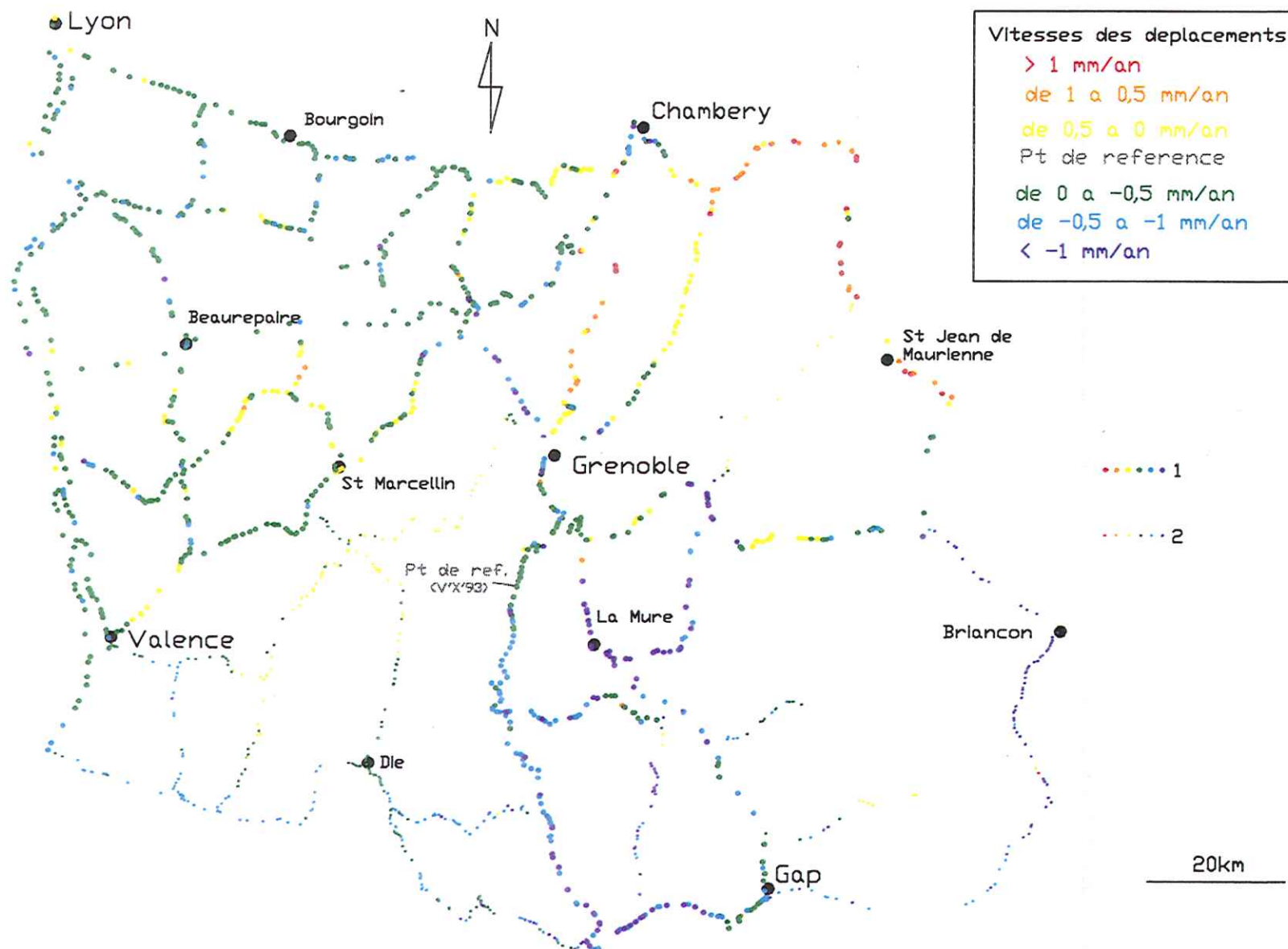
Fig.II-23. Vitesses des déplacements verticaux calculées à partir de données de différentes qualités. La qualité est traduite par le diamètre des points: 1: bonne qualité (malle à bonne fermeture); 2: qualité moindre due à
