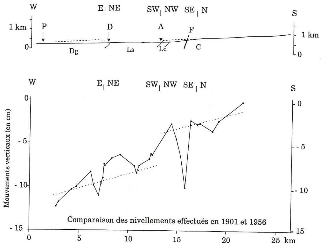
Fig. I-61. Mise en évidence de mouvements verticaux actuels (sur 55 ans) au droit du profil en long du Bréda, par comparaison des nivellements effectués en 1901 et 1956. A: Allevard; C: socle cristallin de Belledonne; D: Détrier; Dg: marmo-calcaires du Dogger; F: faille (d'après la carte géologique au 1/50000); Lc: Lias calcaire; Ls: Lias schisteux; P: Pontcharra.
