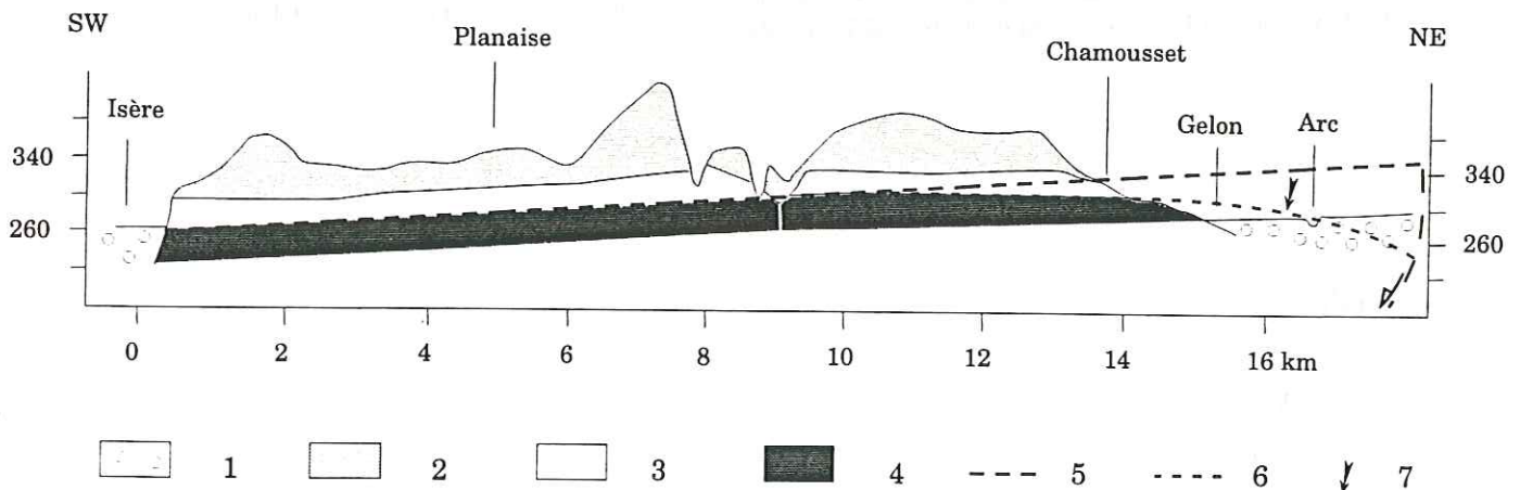
Fig. I-57. Basculement vers le NE des dépôts fluviolacustres du stade inter-glaciaire Riss-Würm (d'après Nicoud, 1983; réinterprété). 1: alluvions actuelles; 2: moraine würmienne; 3: sables fluviolacustres; 4: argiles lacustres; 5: pente initiale de la limite sables/argiles; 6: pente de la limite sables/argiles après basculement; 7: basculement de la limite ayant valeur de roll-over pour une faille NW-SE.
