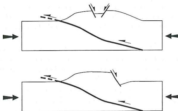
Fig. III-5. Modèles d'extension superficielle en régime compressif. L'extension est principalement une réponse gravitaire à la surrection.
