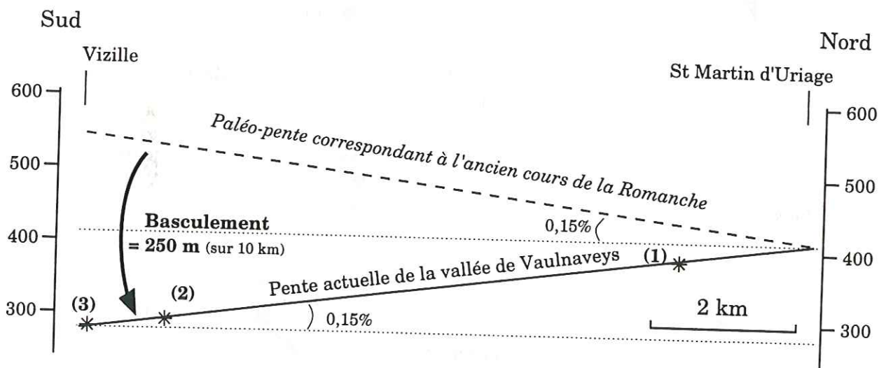
Fig. I-69. Quantification du basculement vers le Sud de la vallée de Vaulnaveys au cours des derniers 65 000 ans. Exagération verticale 10. (1), (2), (3): situation actuelle des affleurements de galets fluviaux témoignant du paléo-cours de la Romanche (cf Fig. I-68).
