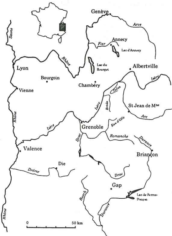
Fig. I-4. Réseau hydrographique simplifié des Alpes nord-occidentales.
