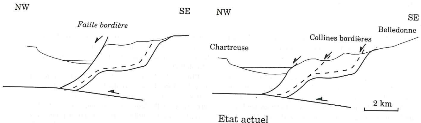
Fig. I-40. Modèle de basculement des failles bordières orientales du Grésivaudan lié au glissement des Collines bordières.
