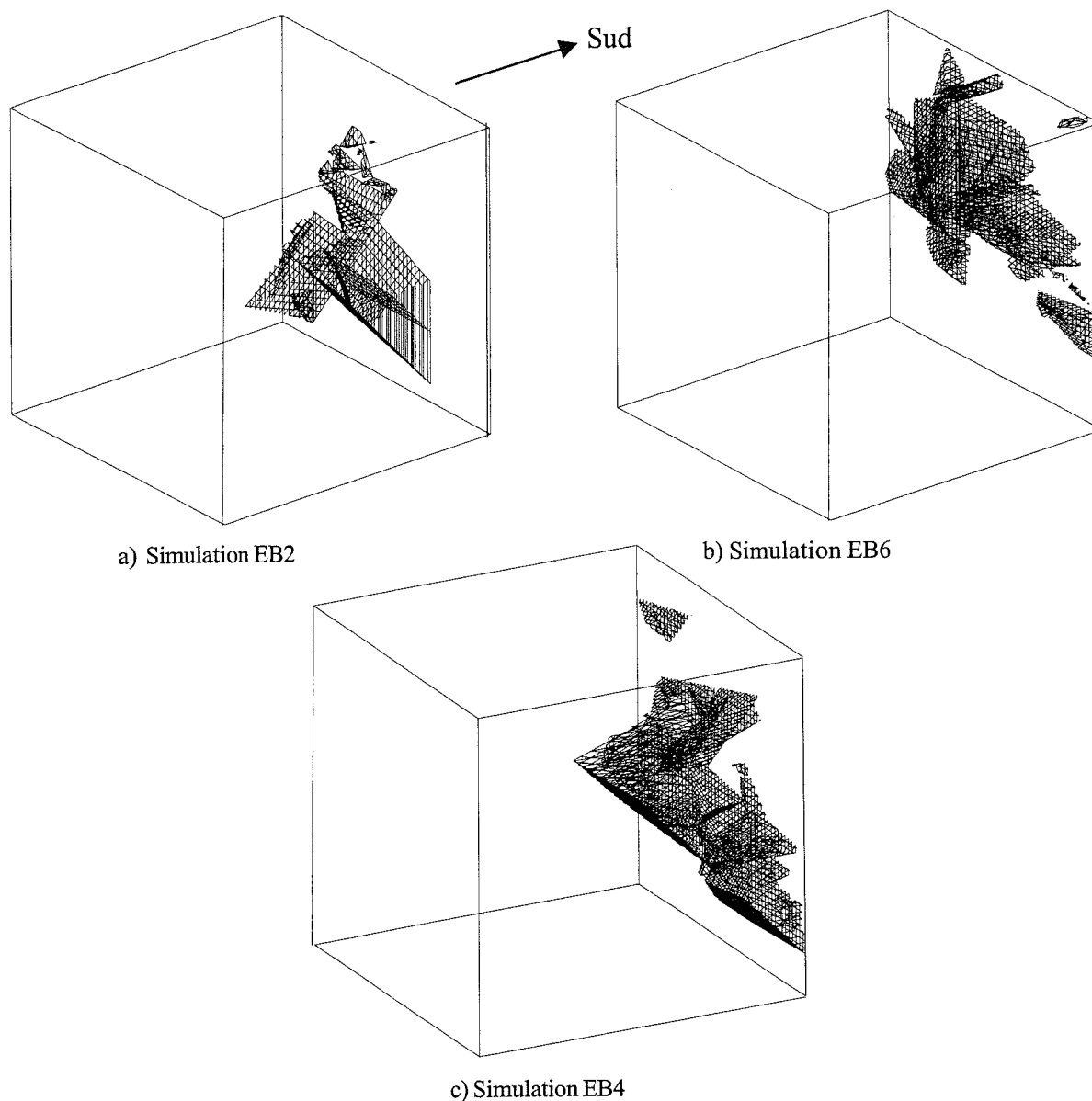
FIG. 198. – Trois exemples d'éboulements sur des volumes cubiques affectés par une fracturation homogène de type « A ». Fractures non recoupantes. a) : Simulation EB2 : 2001 blocs (2000 fractures non recoupantes) – 45 blocs évacués. b) : Simulation EB6 : 5001 blocs (5000 fractures non recoupantes) – 168 blocs évacués. c) : Simulation EB4 : 10001 blocs (10000 fractures non recoupantes) – 80 blocs évacués. La face supérieure et la face de l'éboulement (sud) sont à l'air libre. Les volumes évacués à terme sont représentés en 3D.
