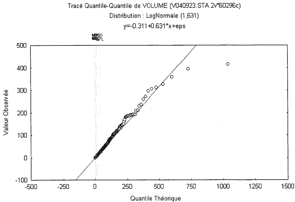
FIG. 85.- Diagramme des quantiles de la distribution des volumes des blocs, pour un ajustement sur une loi lognormale. Scénario D, p=0,8 , 24 salves (60296 blocs).
