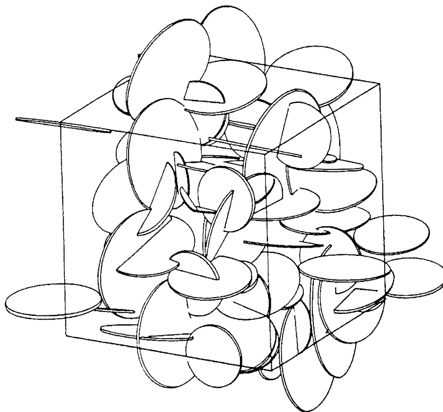
Fig. 9.- Génération stochastique d'un réseau tridimensionnel de fractures représentées par des disques (d'après Billaux [1990]).
