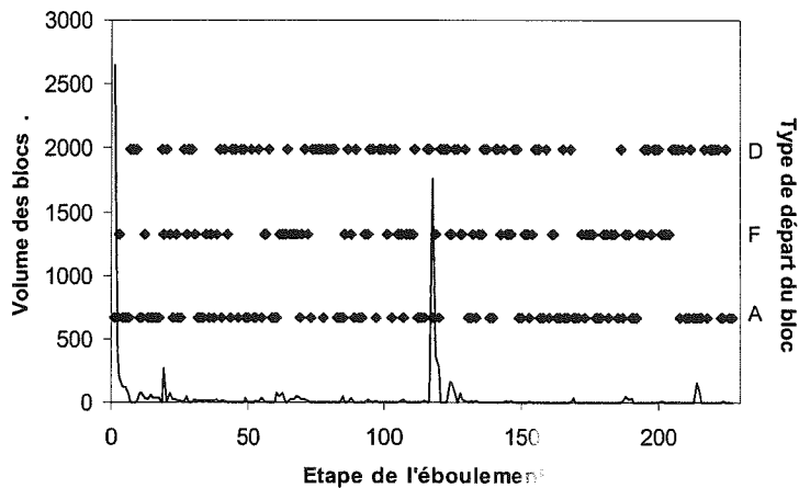
Fig. 194.- Diagramme séquentiel d'un éboulement simulé dans une configuration d'escarpement de stabilité minimale (extrait représentatif). Les volumes des blocs évacués sont figurés par la courbe. Pour chaque événement, le type de déstabilisation est figuré par un point (D = décollement, F = glissement sur une face, A = glissement sur une arête).
