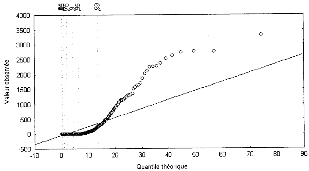
Fig. 83.- Diagramme des quantiles de la distribution des volumes des blocs, pour un ajustement sur une loi lognormale. Scénario C, p=0,6 , 20 salves (11452 blocs).
