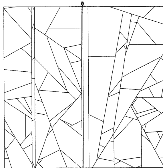
FIG. 143.- Deux exemples de l'effet de la « contrainte de segment vide ». Simulations dans un cube de 50 m d'arête traversé verticalement par le puits EPS1, pour z entre -1900 m et -1850 m. Les simulations comportent 500 fractures périphériques non recoupantes, et aucune fracture imposée. En haut, simulation de type A (bloc aléatoire) ; en bas simulation de type B (position aléatoire du germe). La zone du puits est cloisonnée précocement par des fractures subverticales. Du fait du processus de tirage aléatoire des coordonnées du germe, le « couloir » ainsi formé autour du puits est plus étroit dans le cas B, à nombre de fractures égal.
