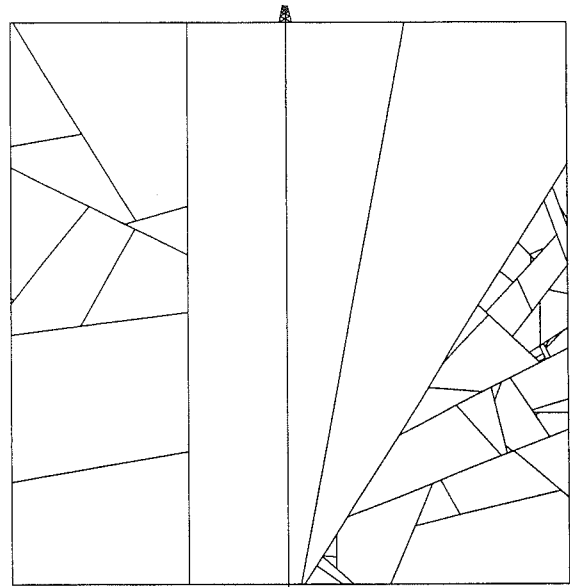
FIG. 142.- Illustration de la contrainte imposée lors du tirage du plan d'une fracture locale dans le but de couper le bloc B. Etant donné le germe g, le tirage des plans P_A , P_B et P_C n'est pas satisfaisant car ces plans coupent le puits. Le plan P_D , lui, peut être retenu.
