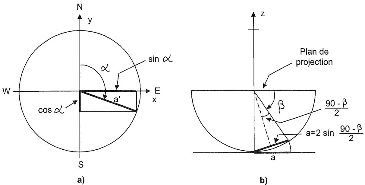
FIG. 47.- Principe de la projection de Schmidt. a) Vue en plan, b) Vue en coupe verticale. En b), on a : a = 2 \sin \frac{(90 - \beta)}{2} . Le module de projection a' = k.a est à ramener sur un cercle de diamètre unité. On écrit cette condition pour b=0 : a' = 1 = k.a = k.2 \sin(45^\circ) , ce qui donne k = \frac{\sqrt{2}}{2} , d'où finalement a' = \sqrt{2} \sin \frac{(90 - \beta)}{2} .
