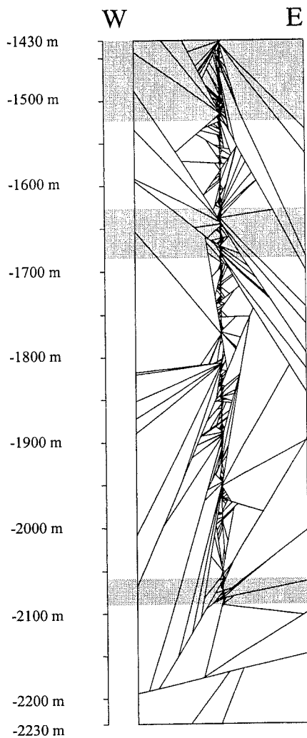
FIG. 158.— Simulation réalisée dans un volume de 200 m (X) x 200 m (Y) x 800 m (Z) autour du puits EPS1 (profondeurs Z comprises entre -1430 m et -2230 m), prenant en compte les seules fractures du puits (aucune fracture périphérique). Le tirage des fractures est pondéré par l'épaisseur. L'épaisseur des 12 zones hydrothermalisées (30 cm à 24 m) est donnée par la figure 156. L'épaisseur des 2944 autres fractures relevées sur carottes dans le puits, entre -1430 m et -2091 m a été fixée arbitrairement à 3 mm. Les trois zones grisées correspondent aux zones où la densité est maximale sur l'intervalle carotté (fig. 132).
