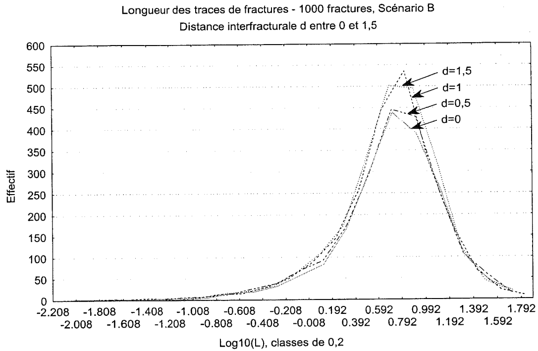
FIG. 106.- Processus B. Effet de la variation de la distance interfracturale \Delta_F sur la distribution des longueurs de traces. 1000 fractures.
