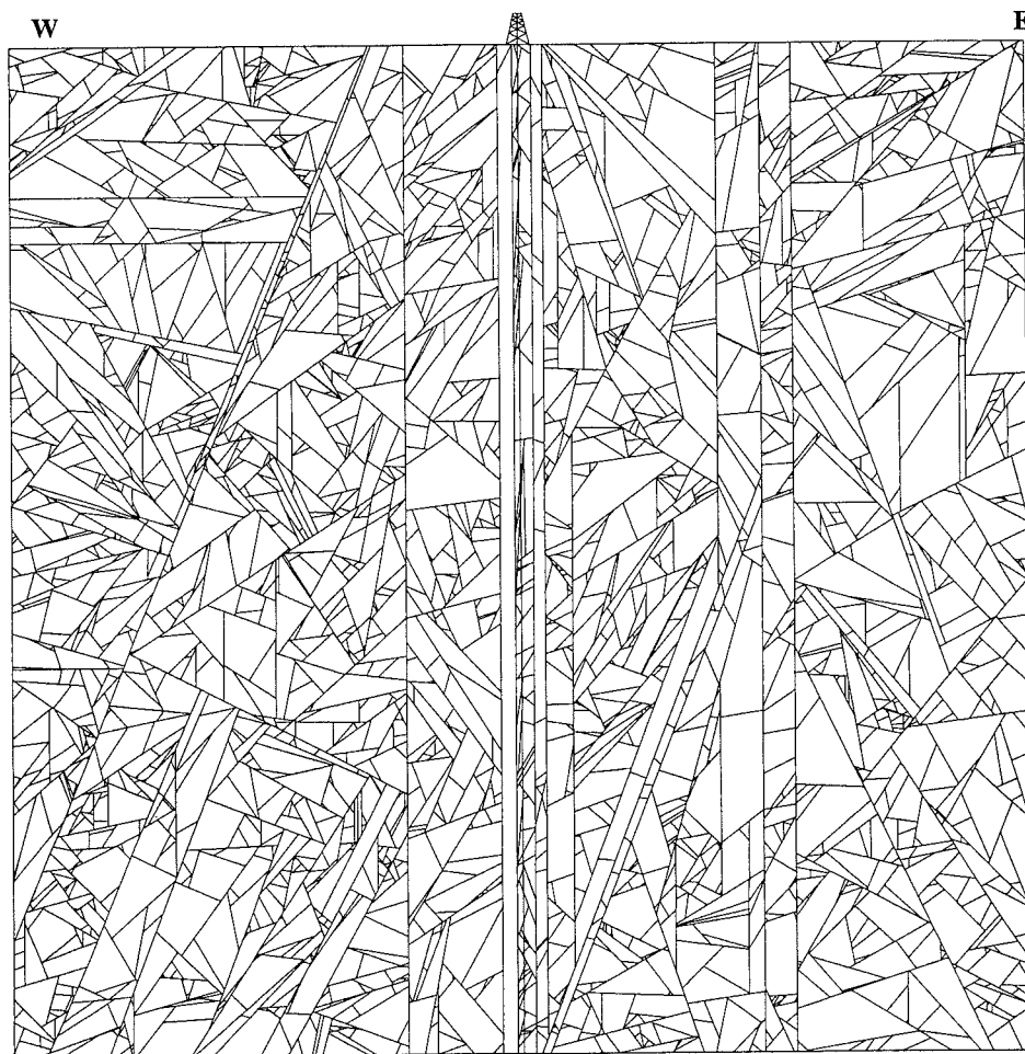
FIG. 144. – Simulation de 70 000 fractures dans un volume de 50x50x50 m, autour du puits EPS1 pour des profondeurs entre -1850 et -1900 m. Coupe verticale W-E passant par le puits. Les 146 fractures relevées visuellement sur carottes dans le puits sont représentées. Scénario « Fractures imposées finales » : Une phase de type B (20000 fractures), est suivie d'une phase de type A (49860 fractures périphériques, puis les 146 fractures imposées. Représentation réalisée avec AutoCAD.
