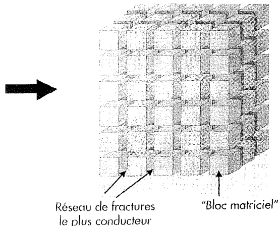
FIG. 5.- Schématisation d'un réseau de fractures par un modèle de type double porosité (D'après Warren et Root [1963] ; Massonnat [1994]).
