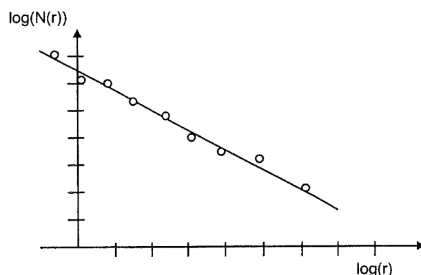
FIG.13.- Calcul empirique de la dimension de Hausdorff sur un graphe bilogarithmique. N(r) est le nombre d'objets de taille supérieure à r . La dimension de Hausdorff D_H est la pente de la droite obtenue (D'après Dubois [1995]).
