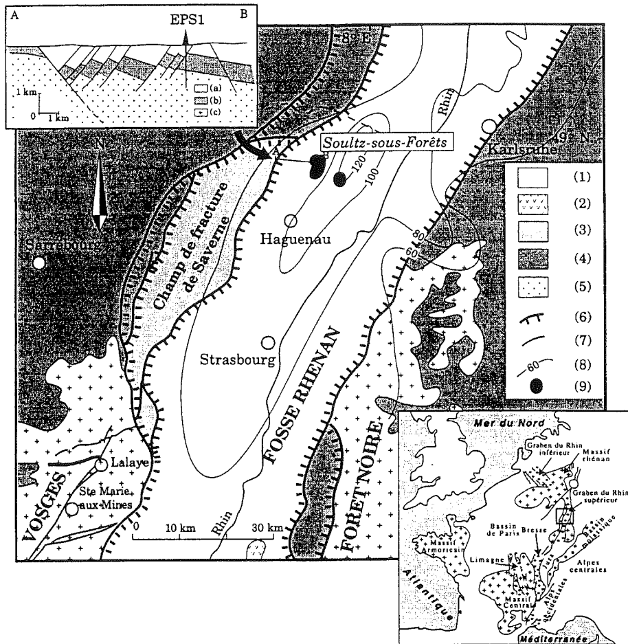
FIG. 117.- Carte géologique structurale simplifiée du fossé rhénan : (1) Remplissage sédimentaire oligo-miocène, (2) Volcanisme cénozoïque, (3) Jurassique, (4) Trias germanique, (5) Socle hercynien, (6) Failles bordières du graben, (7) failles, (8) Isogrades géothermiques (°/km) (9) Zones d'investigation géothermique (d'après Dezayes [1995]).
