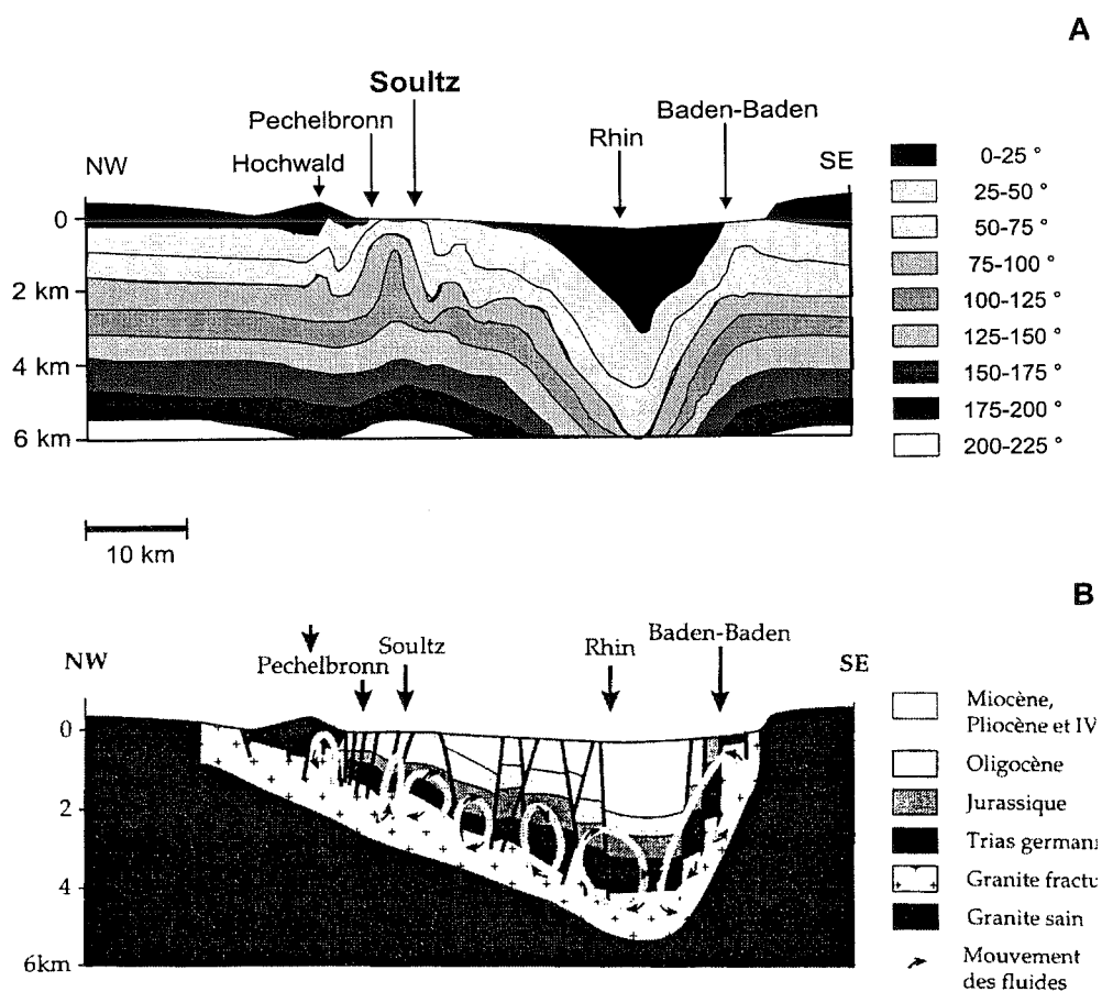
FIG. 119.- Coupe géologique passant par le forage géothermique GPK1 (d'après Cautru [1987] modifiée par Dezayas [1995]). Coupe réalisée par les données de sismique réflexion. On observe les failles normales antithétiques permettant une remontée du socle granitique jusqu'à -1400 m.
