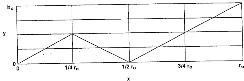
FIG. 17.- Application de la méthode de comptage de boîtes sur un fractal auto-affine. Pour déterminer sa dimension, on utilise des rectangles de largeur r_j=r_0/4 et de hauteur h_j=h_0/4 . L'objet est recouvrable par les N_j=8 rectangles grisés. Puisque N_0=1 pour la boîte de hauteur h_0 et de largeur r_0 , on obtient D=3/2 . [Turcotte, 1997]
