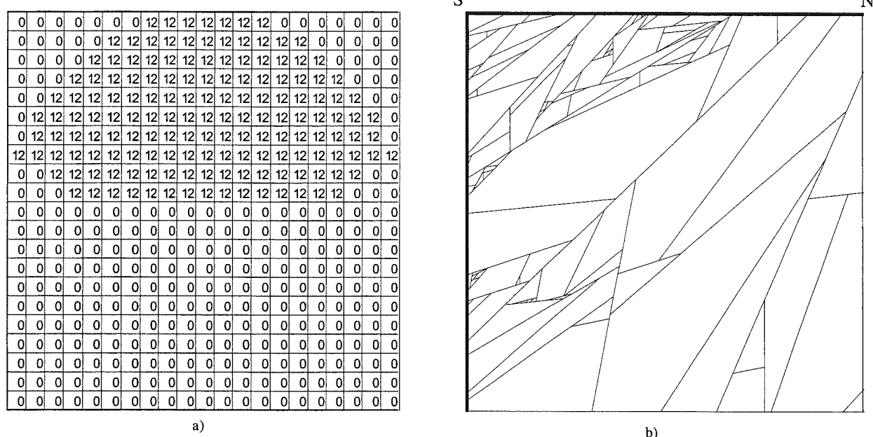
Fig. 193.– Simulation d'éboulement réalisée sur un bloc rocheux parcouru par une fracturation d'orientation E-W, d'inclinaison dominante de secteur Sud. 1848 fractures non recoupantes. a) Matrice des pôles de fractures (Schmidt hémisphère inférieure) correspondant au jeu de fractures parcourant le bloc modélisé dans la figure 195. b) Coupe verticale N-S dans le modèle. La paroi à l'air libre est représentée par le trait épais (orientation E-W).
