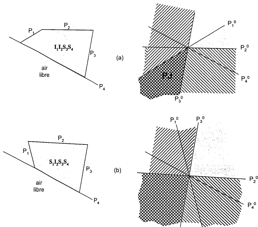
FIG. 171.— Illustration en 2D du théorème de Shi sur la « dégageabilité » du bloc. a) : Bloc libre ou dégageable. Le bloc est l'intersection des demi-espaces I_1I_2S_3S_4 . Pour obtenir sa pyramide de joints (à droite) on considère les plans formant les joints du bloc, P_1^0, P_2^0, P_3^0 , qui sont la translation à l'origine des plans P_1, P_2 et P_3 . L'intersection des demi-espaces I_1I_2S_3 donne la pyramide des joints (PJ). Celle-ci est un ensemble non vide ; d'après le théorème de Shi, le bloc est libre. On remarque que la pyramide du bloc, obtenue par intersection de PJ et du demi-espace S_4 , est vide, indiquant que le bloc est fini. b) : Bloc non libre ou coincé. Le bloc est l'intersection des demi-espaces S_1I_2S_3S_4 . De la même façon que pour (a), la pyramide des joints est formée par l'intersection des demi-espaces S_1I_2S_3 à partir des plans translétés. Dans ce cas, la pyramide des joints, comme la pyramide du bloc sont vides, confirmant qu'il s'agit d'un bloc fini, et non libre.
