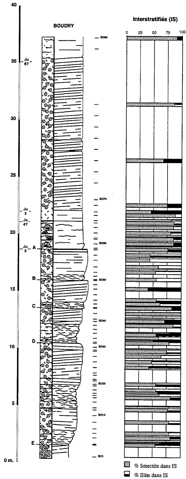
FIG. 108.— Coupe de Boudry, composition des interstratifiés (fraction <2\mu\text{m} glycolée).
