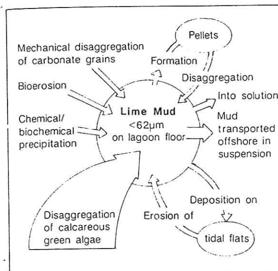
FIG. 21. – Bilan du cycle des boues carbonatées, « Bight of Abaco, Bahamas », d'après Tucker et Wright [1990].
