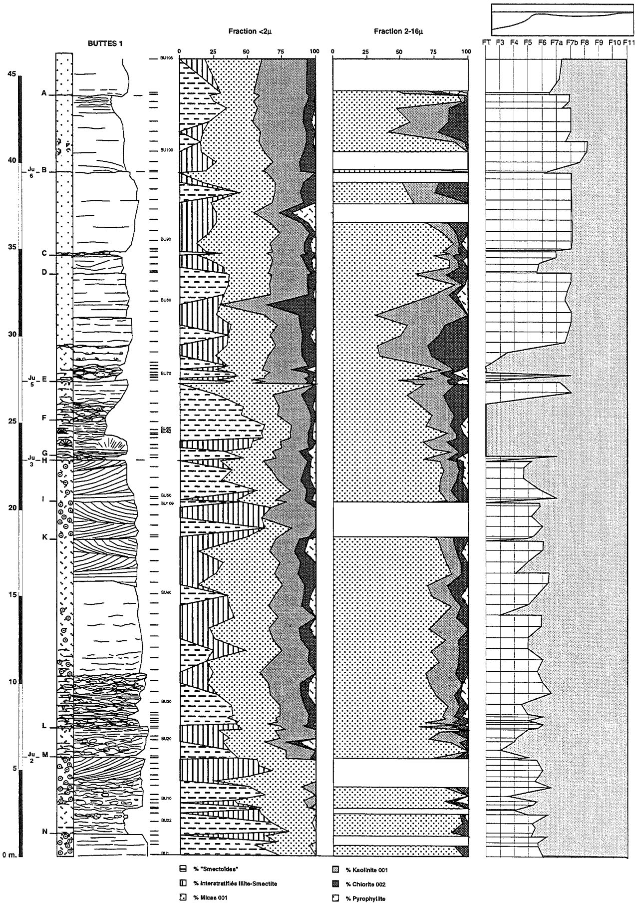
FIG. 117.- Coupe de Buttes 1, pourcentages relatifs des phyllosilicates des fractions <math><2\mu\text{m}</math> et <math>2-16\mu\text{m}</math>, comparaison avec la courbe de microfaciès.
