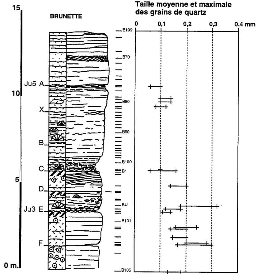
FIG. 95.- Coupe de Brunette, taille des grains de quartz.
