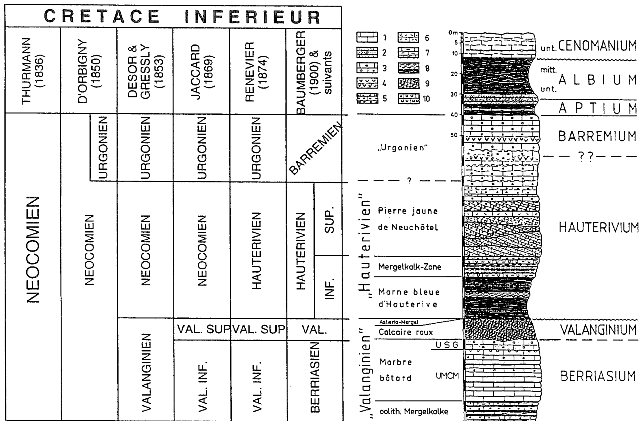
FIG. 7.— Evolution historique du Néocomien dans la région stratotypique : coupe synthétique d'après Remane [1982] et tableau d'après Adatte et Rumley [1989]. Légende : 1, calcaire micritique ; 2, calcaire sableux ; 3, calcaires à pellets (pelmicrite/pelsparite) ; 4, calcaire récifal ; 5, calcaire oolithique (oosparite) ; 6, débris de fossiles (biosparite) ; 7, Marnocalcaires ; 8, marnes à calcaires marneux ; 9, calcaire à oolithes ferrugineuses et stratification oblique ; 10, terriers ; USG, "Unité supérieure gréseuse" ; UMCM, "Unité moyenne calcaire massive".
