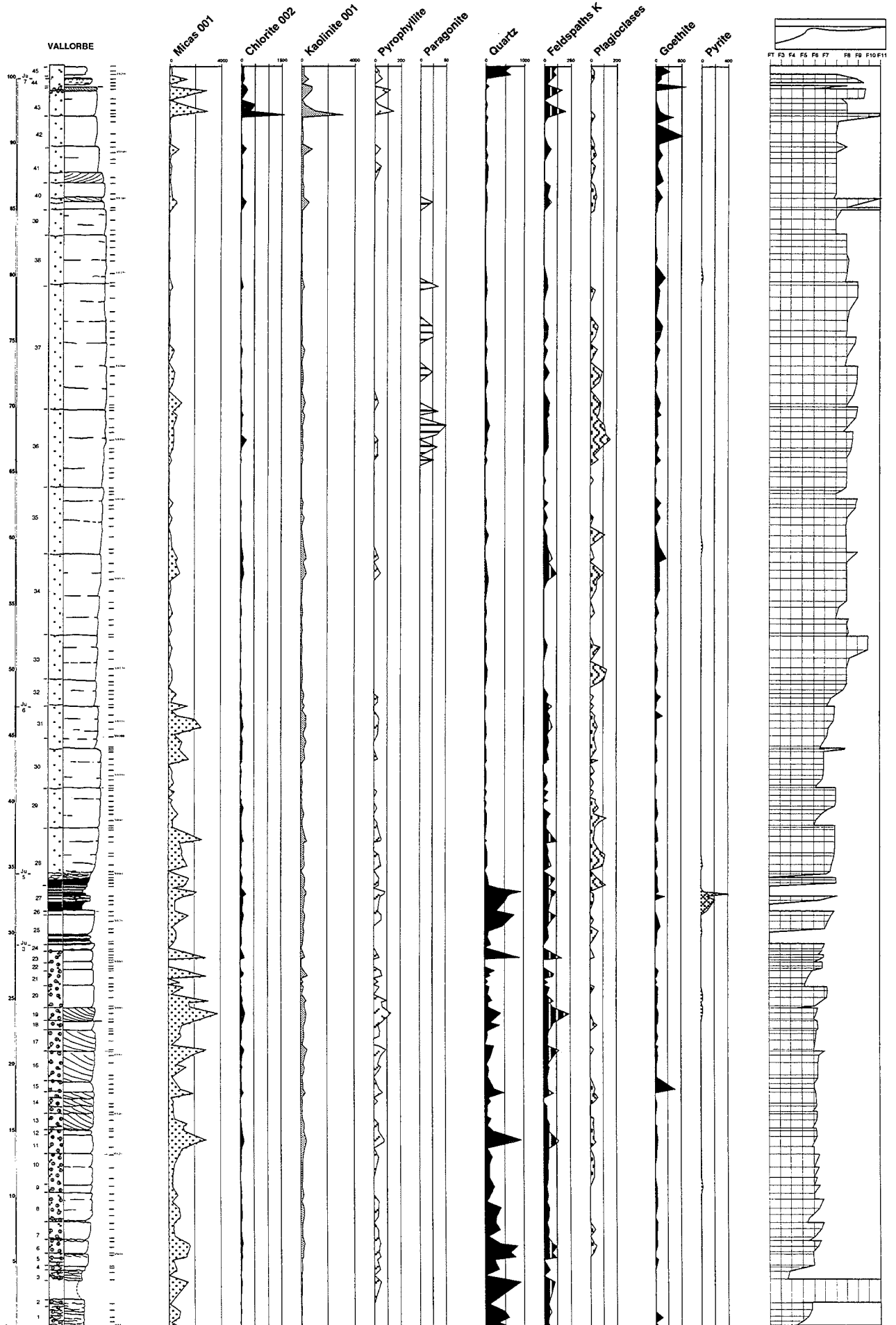
FIG. 144.- Coupe de Vallorbe, répartition des minéraux argileux, silicatés et ferrifères (fraction 2-16 µm), intensités en Coups Par Seconde (CPS). Géologie Alpine , 1995, Mémoire H.S. n° 24
