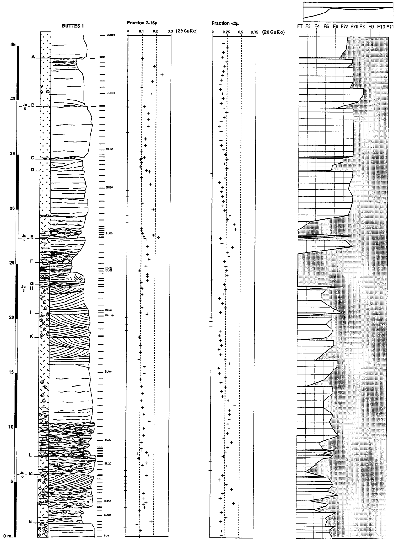
FIG. 116.- Coupe de Buttes 1, largeurs de Scherrer (fractions 2-16μm et <2μm) ; comparaison avec la courbe de microfaciès.
