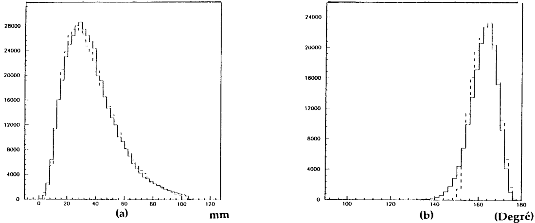
Figure 3.12: Distribution (a) en position, (b) angulaire, des fragments de fission prompte en coïncidence dans la région permise. Expérience (trait plein) et simulation (tirets).
