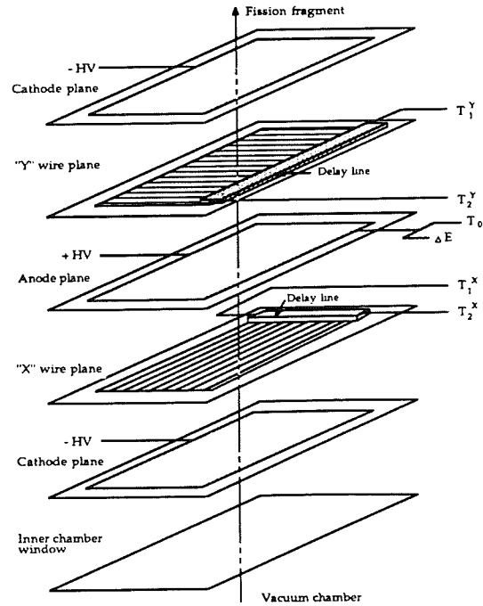
Figure 2.8: Le détecteur PPAC utilisé par l'expérience PS177 en 1988. Figure extraite de la référence [34]
