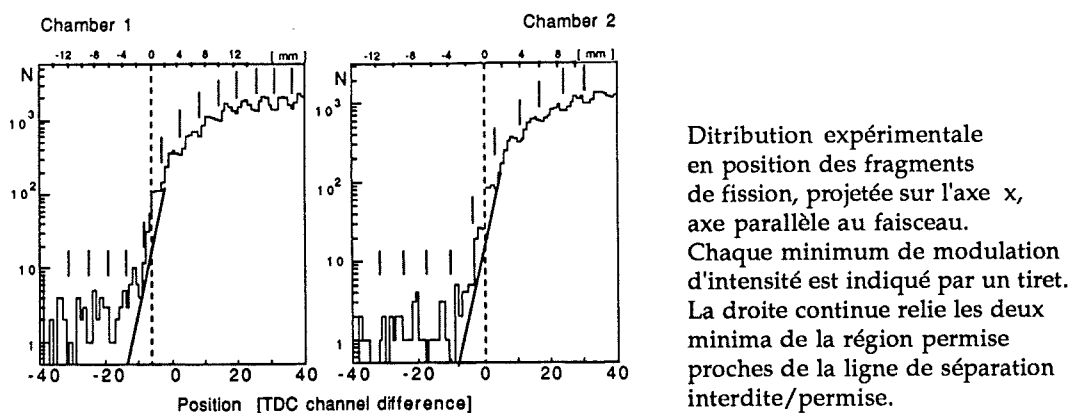
Figure 3.6: Distribution en position dans les PPACs. Méthode de détermination de la ligne de séparation entre les zones interdite et permise. Figure extraite de [34]
