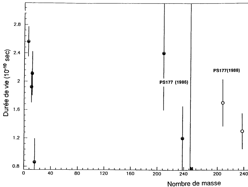
Figure 4.4: Durées de vie expérimentales
