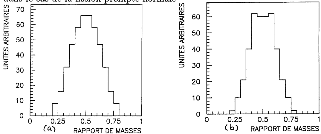
Figure 2.32: Distribution symétrisée des rapports de masses N_F en fonction de R_1 dans le cas (a) des hypernoyaux de fission prompte, (b) des hypernoyaux de fission retardée
