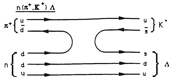
Figure 1.2: Diagramme des lignes de quarks de la réaction n(\pi^+, K^+)\Lambda
