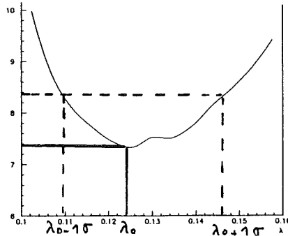
Figure 3.22: \chi_\lambda^2 en fonction de \lambda
