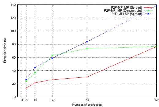
(e) sparseMatMult
