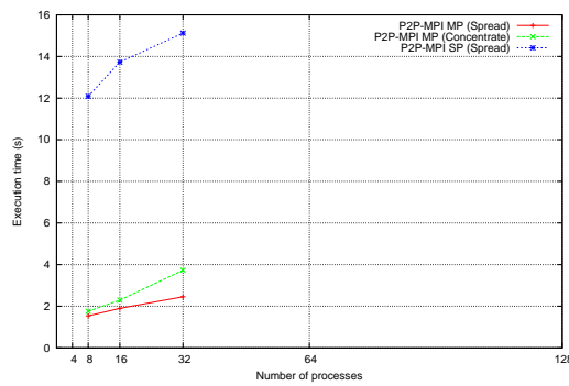
(d) sor
