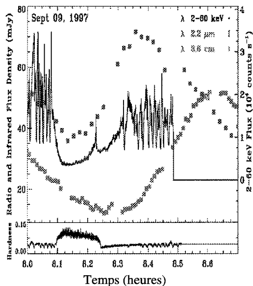
FIG. 2.16 – Courbe de lumière X, Infra-rouge, Radio, ainsi que le rapport de dureté (flux 13-60 keV / flux 2-13 keV) de GRS 1915+105, pendant le passage d'un état haut à un état bas (Mirabel et al. 1998).
