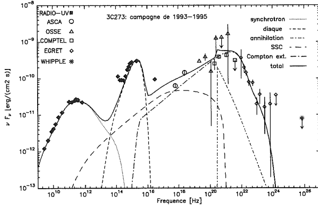
FIG. 2.7 – À gauche: spectre simulé comparé aux observations multi-longueur d'onde quasi-simultanées de 3C 273 (Von Montigny et al. 1997). À droite: paramètres utilisés pour obtenir le spectre synthétique. M est unité de 10^8 M_\odot , \dot{M} en M_\odot \cdot \text{an}^{-1} , B_0 en Gauss et z_1 en r_g .
