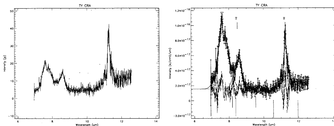
Figure V.6 – Idem que figure V.4 pour les émissions PAH à 7,7 , 8,6 et 11,3 \mu m
