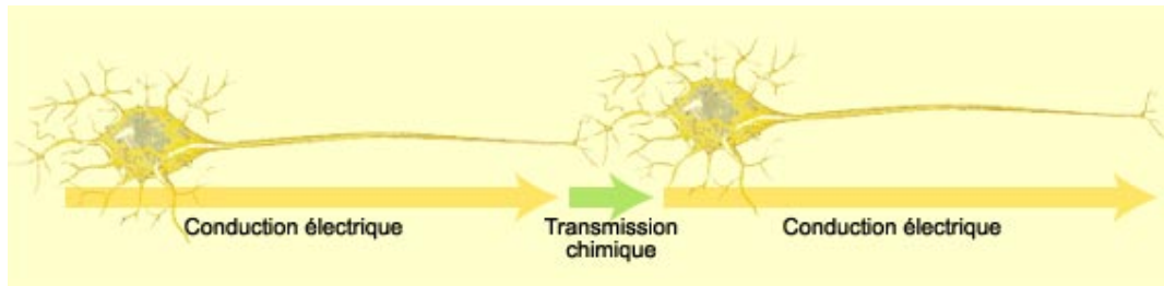
FIGURE 1.2 – La communication neuronale repose sur des conceptions électriques le long des axones, et chimiques (ou électriques) au niveau des synapses. Source des dessins : Cerveau à tous les niveaux.
