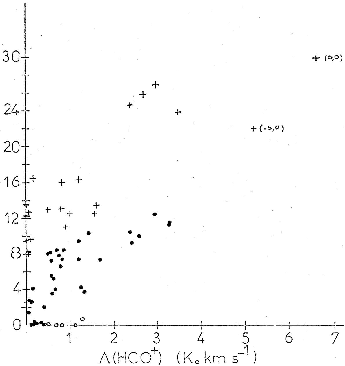
Figure D7 : Comparaison des aires de raies \text{HCO}^+ et ^{13}\text{CO} en chaque point du nuage.
