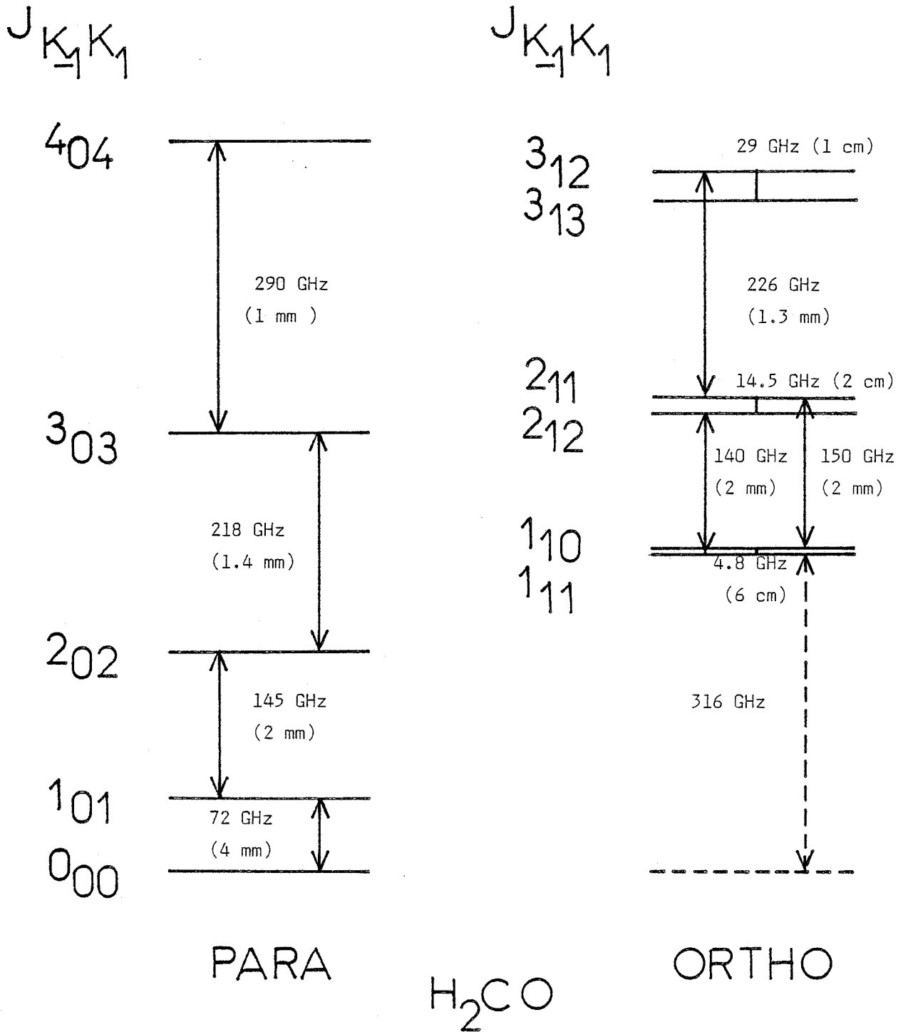
Figure B3 : Les premiers niveaux de rotation de la molécule H2CO ainsi que les fréquences et les longueurs d'onde des transitions rotationnelles observées dans les nuages moléculaires. La flèche en pointillés indique la différence d'énergie entre le fondamental de l'orthoformaldéhyde et celui du paraformaldéhyde.
