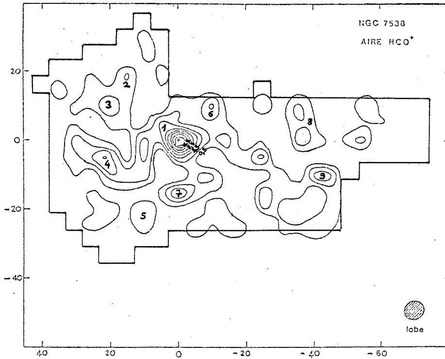
Figure D6 : Isophotes d'aire de raies \text{HCO}^+ ( J=1-0 ). L'intervalle entre 2 contours est de 2 \text{K km/s} et le contour minimal correspond à 0,5 \text{K km/s} . Les coordonnées du point (0,0) sont les mêmes que dans la figure D4. La numérotation des condensations est celle du texte.
