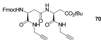
Figure 101 – Dimère 70 formant un organogel
