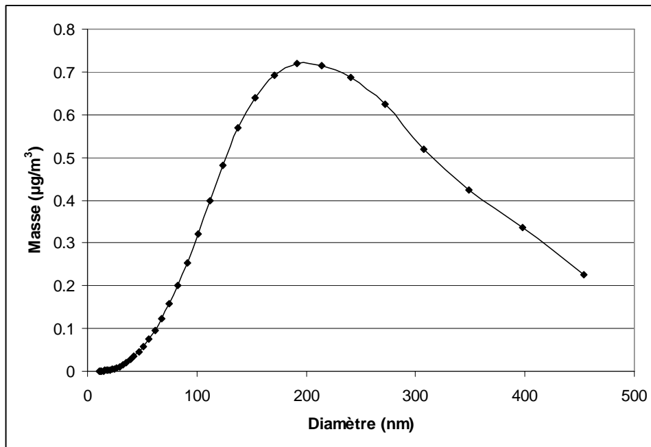
Figure 39 : Spectre moyen de la masse de l'aérosol en fonction de la granulométrie lors de la campagne de Marseille. Mise en évidence de la forte contribution des particules les plus grosses.
