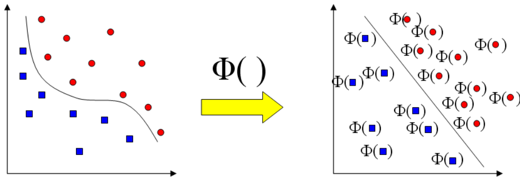
FIGURE 6.3 – Séparation de classes non linéaire
