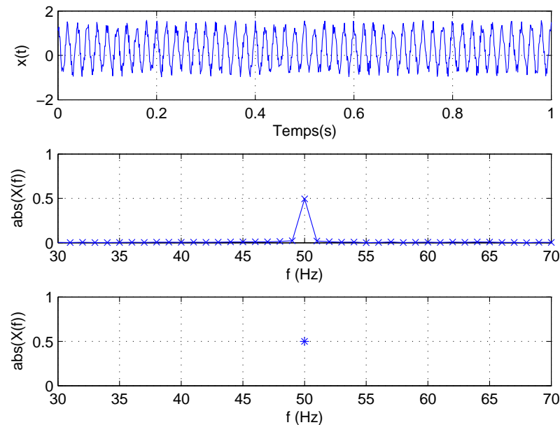
FIGURE 2.10 – Signal x(t) bruité observé sur une durée de 1s, traité avec la TF et la méthode de Matrix Pencil
