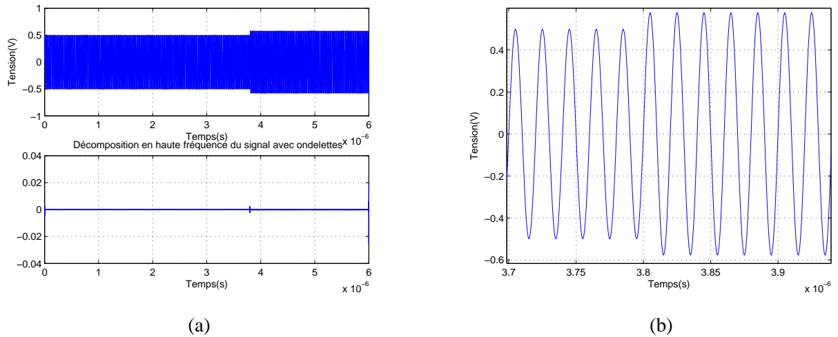
FIGURE 4.20 – (a) : Tension d'entrée et sa décomposition en ondelettes db4 niveau 1, (b) Zoom de la tension lors du changement d'état
