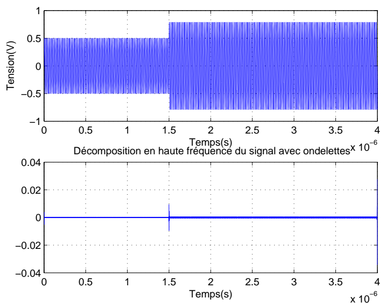
FIGURE 4.16 – Tension d'entrée et sa décomposition en ondelettes db4 niveau 1
