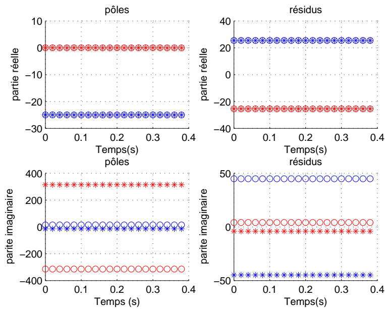
FIGURE 3.20 – Suivi temporel des pôles et résidus pour une charge RLC série R = 1\Omega , L = 20mH et C = 60mF
