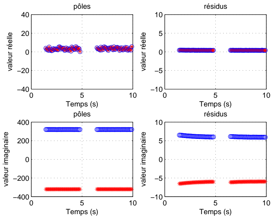
FIGURE 5.9 – Suivi temporel des pôles et des résidus normalisés du courant consommé par le radiateur
