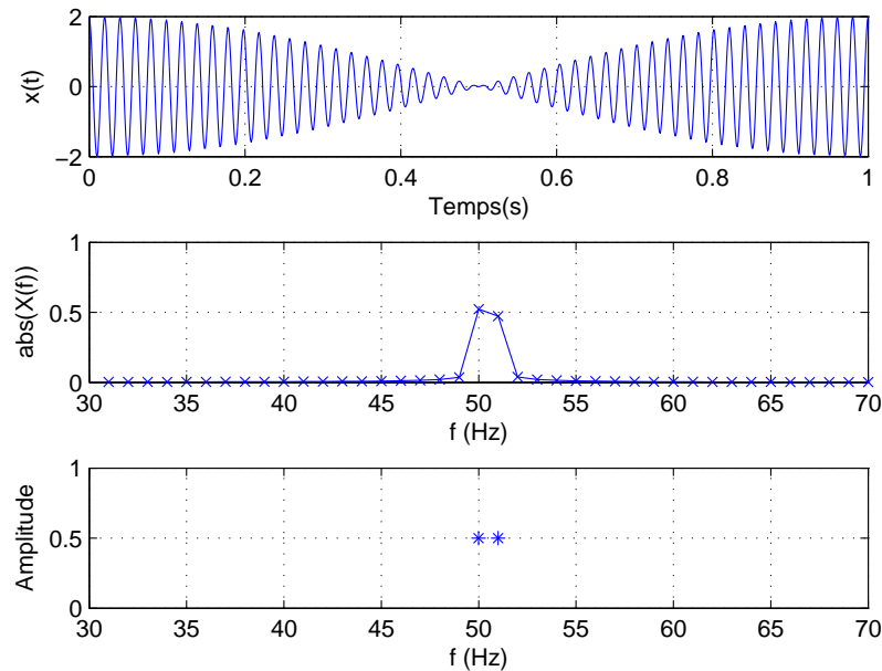
FIGURE 2.8 – Signal x(t) observé sur une durée de 1\text{s} , traité avec la TF et la méthode de Matrix Pencil
