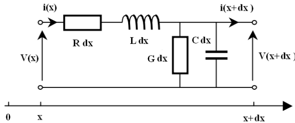
FIGURE 4.1 – Quadripôle équivalent d'une cellule de ligne à deux conducteurs
