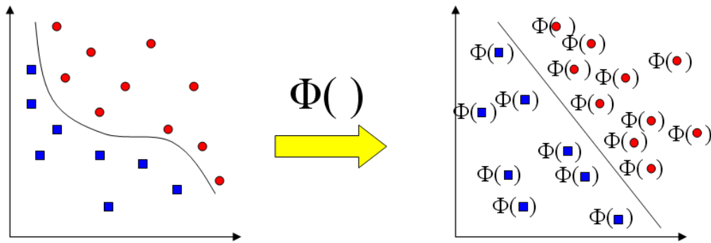
FIGURE 6.3 – Séparation de classes non linéaire
