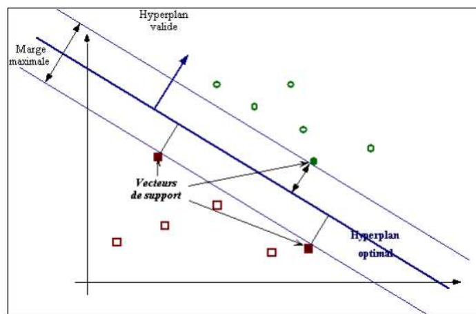
FIGURE 6.1 – Hyper plan de séparation des deux classes
