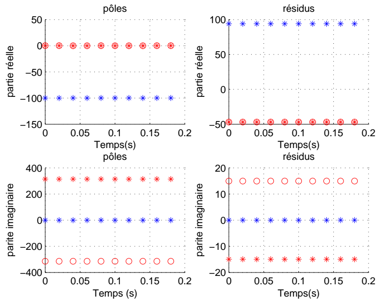
FIGURE 3.17 – Suivi temporel des pôles et résidus pour une charge RL série R = 1\Omega et L = 10mH
