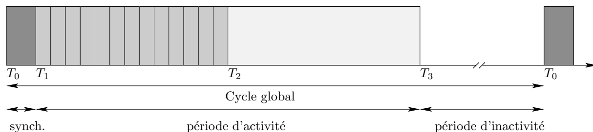
FIG. 3.2 – Le cycle global dans MaCARI.
