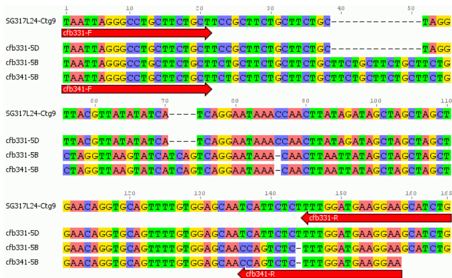
Figure 34 : Alignement entre la séquence du contig Ctg9 issu du clone BAC 317L24 et les deux loci cfb331-5D et cfb331-5B. Une identité de 100% est observée entre le Ctg9 et le locus cfb331-5D indiquant que le clone BAC 317L24 est en fait originaire du chromosome 5D. Le marqueur cfb341 spécifique uniquement du 5B a été désigné en utilisant les SNP identifiés entre les deux séquences.
