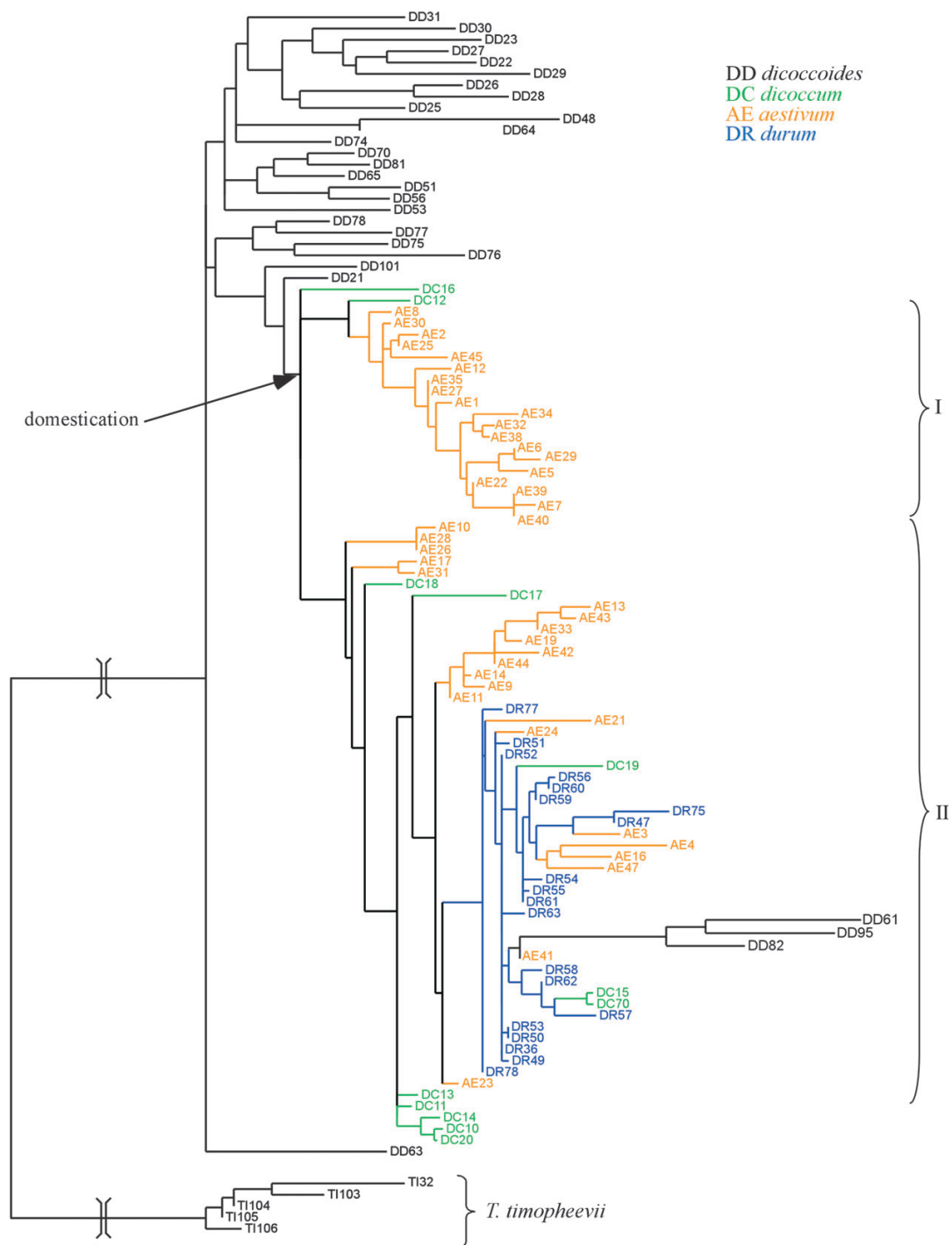
Figure 6 : Arbre phylogénétique construit par HAUDRY et al. (2007) basé sur la comparaison de 21 locus entre les formes sauvages T. turgidum ssp. dicoccoides , la forme cultivée T. turgidum ssp. dicoccum , T. turgidum ssp. durum et le blé hexaploïde T. aestivum . Un seul simple événement de domestication est observé pour le blé amidonnier tandis que les formes cultivées présentent une diversité génétique réduite.
