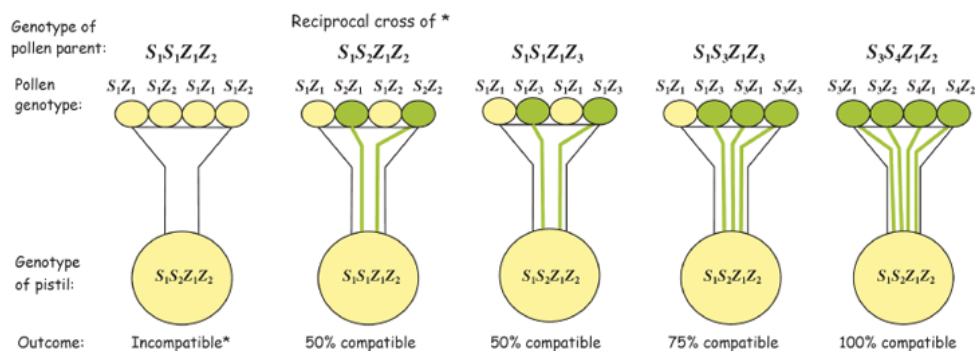
Figure 11: Contrôle génétique de l'auto-incompatibilité gamétophytique (GSI) par deux locus multi-alléliques S et Z . D'après BICHENG et al. (2008).
