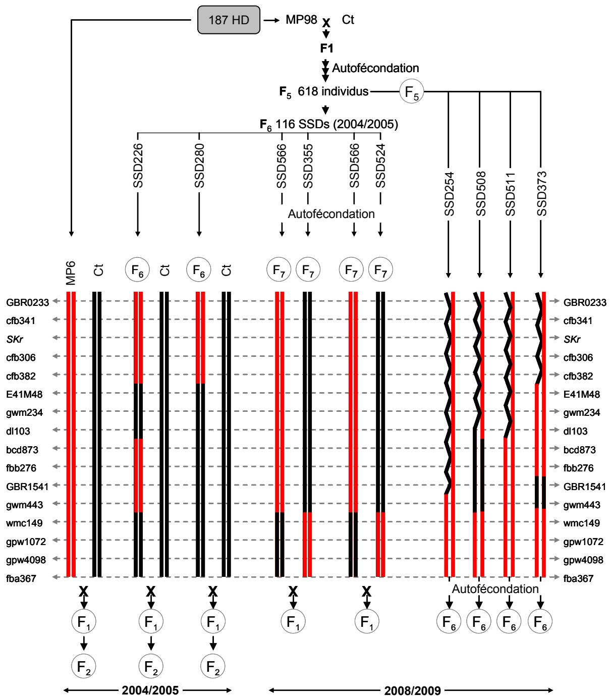
Figure 35: Schéma de production de nouvelles populations (2004/2005) et (2008/009). En noir : le fond génétique de Ct d'origine. En rouge, le fond génétique de MP98.
