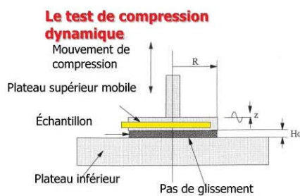
Photo : Test de compression dynamique
