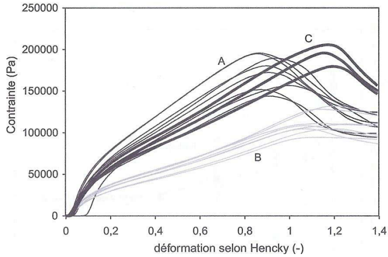
Figure n°8 : Courbe de compression uniaxiale pour 3 fromages Emmental français: une phase linéaire de déformation ( < 0,1 ), une phase d'écoulement puis une phase de rupture (Famelard et al, 2002)
