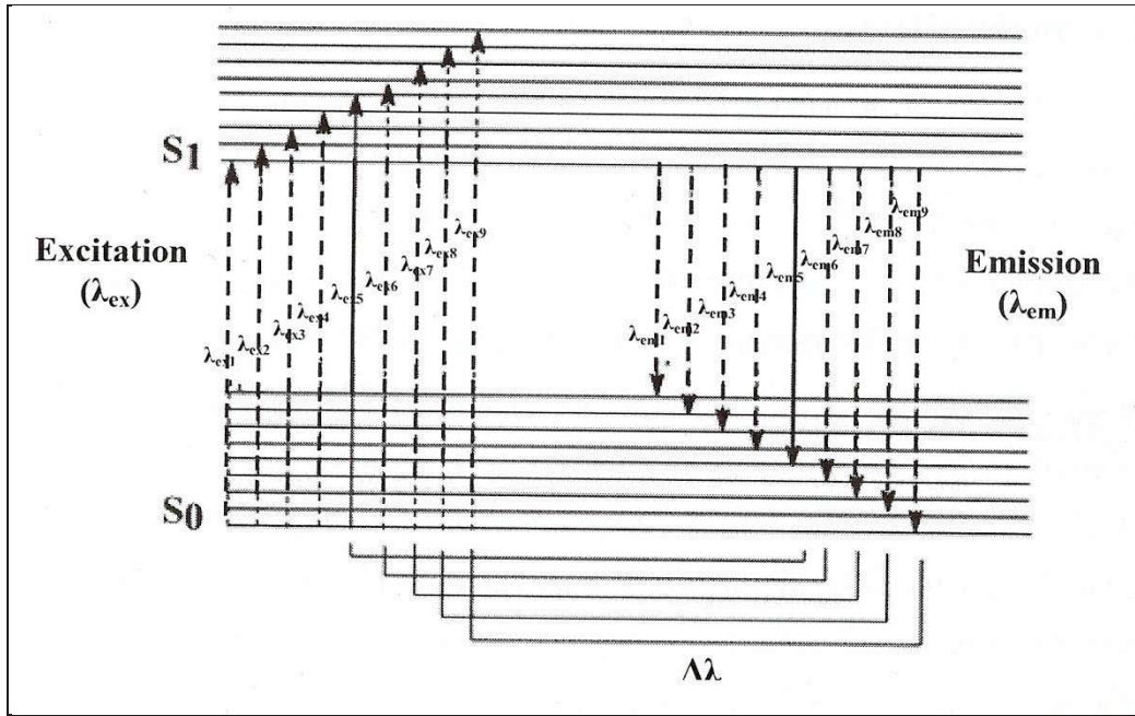
Figure n°13 : schématisation du balayage de fluorescence synchrone (Patra et Mishra, 2002) \Delta\lambda = \lambda_{\text{émi}} - \lambda_{\text{exi}}
