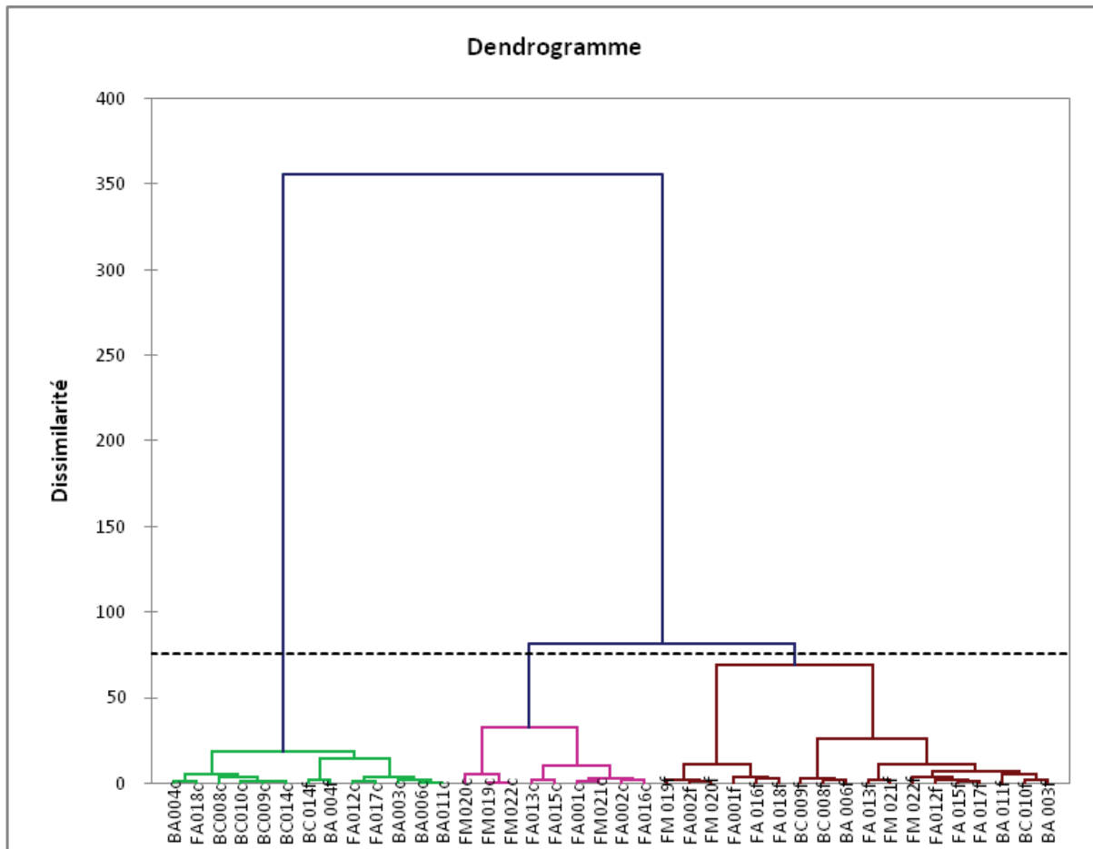
Figure n°22 : Classification hiérarchique ascendante (dissimilarité, méthode de Ward) sur les notes des 13 descripteurs pour les fromages à chaud et à froid.
