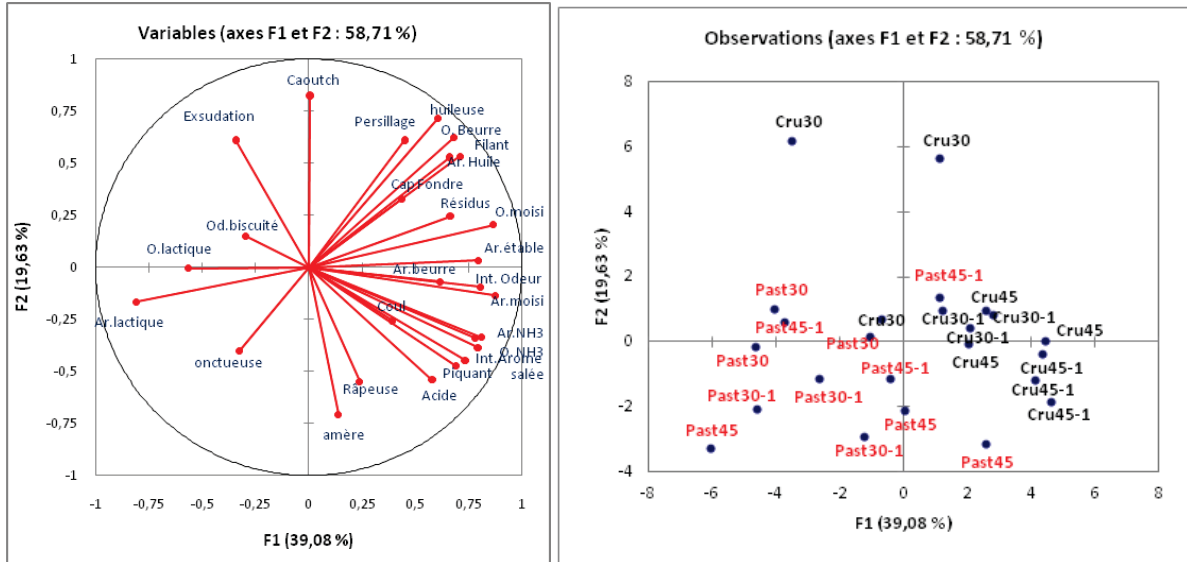
Figure n°21 : Cercle de corrélation et carte des Fourmes d'Ambert issus de l'ACP sur les plans factoriels 1-2
