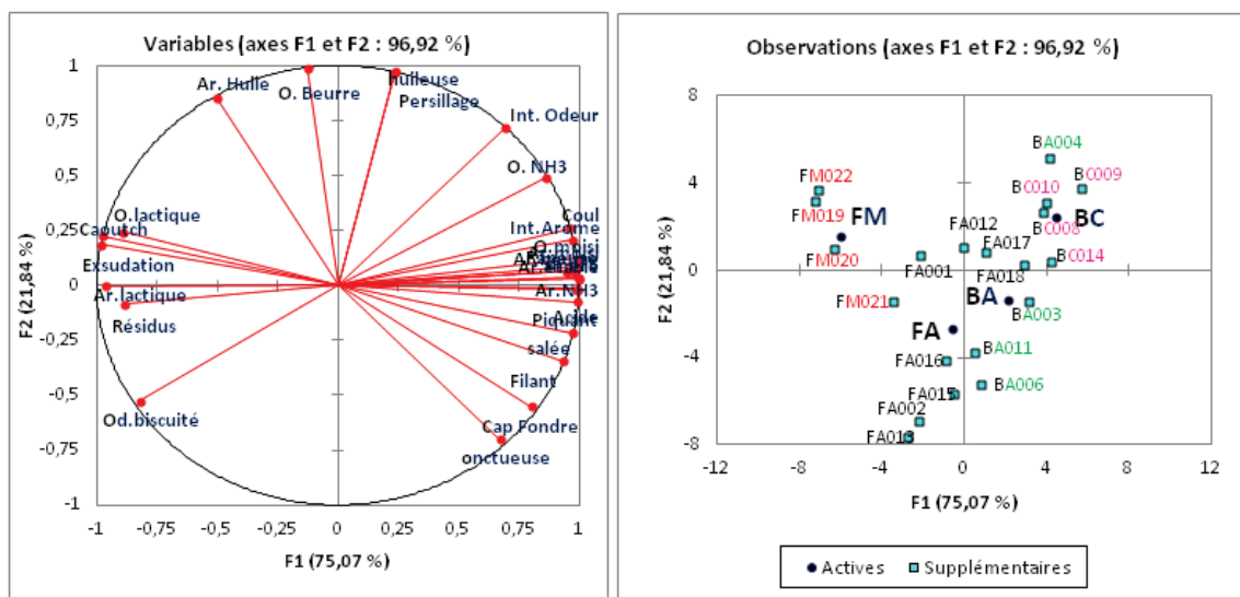
Figure n°19 : ACP représentant les descripteurs sensoriels et les 4 catégories de fromages sur les axes factoriels 1-2. Les 20 échantillons de fromages sont en observations supplémentaires.
