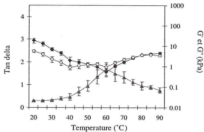
Figure n°10 : Courbe de test de cisaillement dynamique avec balayage température sur des fromages expérimentaux de type pâte pressée (n=10 Mamirolle) (triangle : \tan\delta , losange plein : G' , losange vide : G'' ) (Reparet et al 2003)
