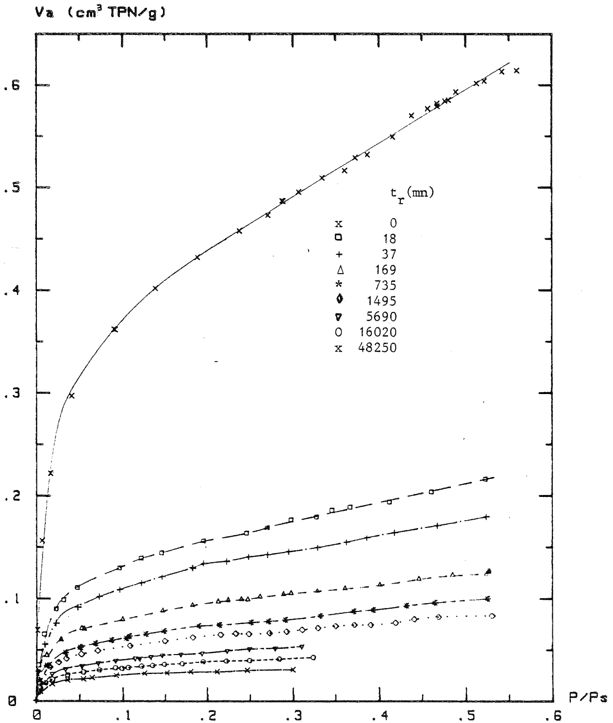
Figure 4.11 : ISOTHERME D'ADSORPTION N2 (77K) V_a=f(X) Glace Ih Broyée à 77K , Resultats successifs à 195.45K (Ech.6)
