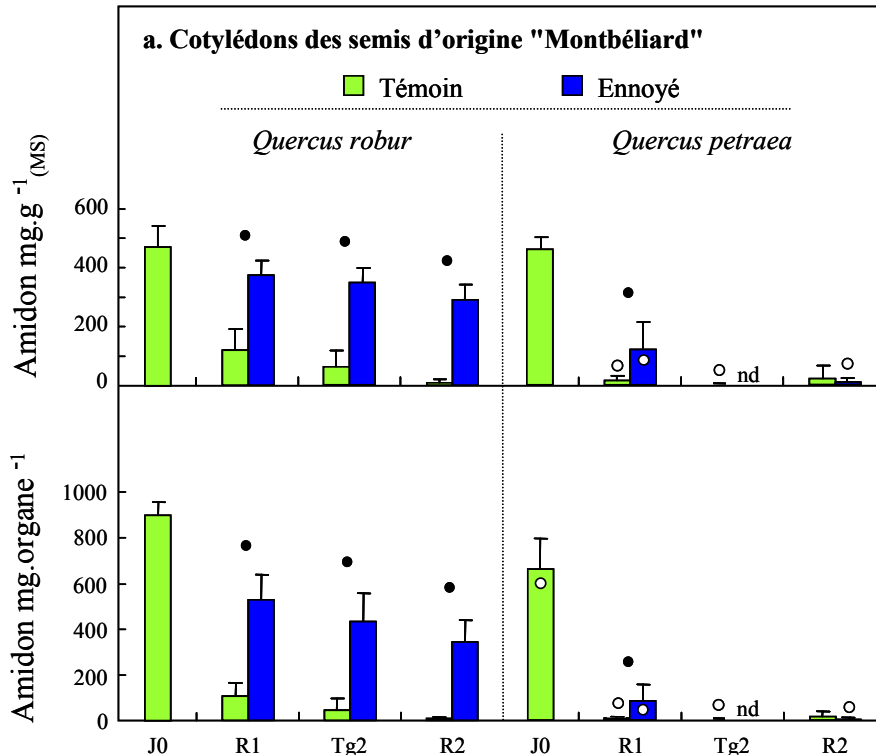
Figure 12. Variations des teneurs en amidon exprimées en équivalent glucose, en mg.g -1 de matière sèche (MS), et des quantités totales en amidon exprimées en mg.organe -1 des cotylédons (a) des semis témoins et ennoyés de Quercus robur et de Quercus petraea d'origine "Montbéliard" aux récoltes J0, R1, Tg2 et R2, et (b) des semis témoins, ennoyés et ennoyés puis drainés de Quercus robur et de Quercus petraea d'origine "ONF" aux récoltes J0, J15, R1, R1 D+10 et R2. Le drainage des semis ennoyés est effectué à la récolte R1. Les semis ennoyés de Q. petraea d'origine "Montbéliard" (a) n'ont pas développé de deuxième étage. A la récolte R2 ces semis sont toujours au stade de repos apparent du premier étage foliaire. Les mesures sur les semis d'origine "ONF" (b) ont été effectuées sur les mêmes semis que ceux utilisés dans les Figure 13 et Figure 16.
