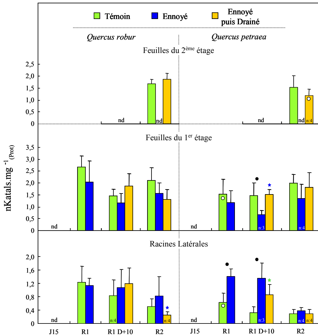
Figure 18. Activité de la glutamine synthétase, en nKatsals (nmoles de produit ( \gamma -GH) formées par secondes) par mg de protéines (nKatsals.mg -1 Prot), dans les feuilles du 1 er et du 2 ème étage et dans les racines latérales des semis témoins, ennoyés et ennoyés puis drainés de Quercus robur et de Quercus petraea d'origine "ONF" aux récoltes J15, R1, R1 D+10 et R2. Le drainage des semis ennoyés est effectué à la récolte R1.
