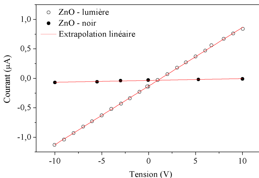
FIGURE 3.20 – Évolution de la courbe courant tension pour un film mince de ZnO , en fonction de la lumière incidente
