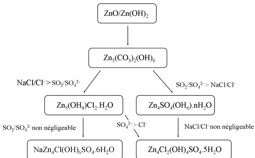
FIGURE 1.3 – Évolution des produits de corrosion du zinc en fonction des polluants présents [45]
