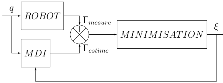
FIG. 1.22 – Identification dynamique
