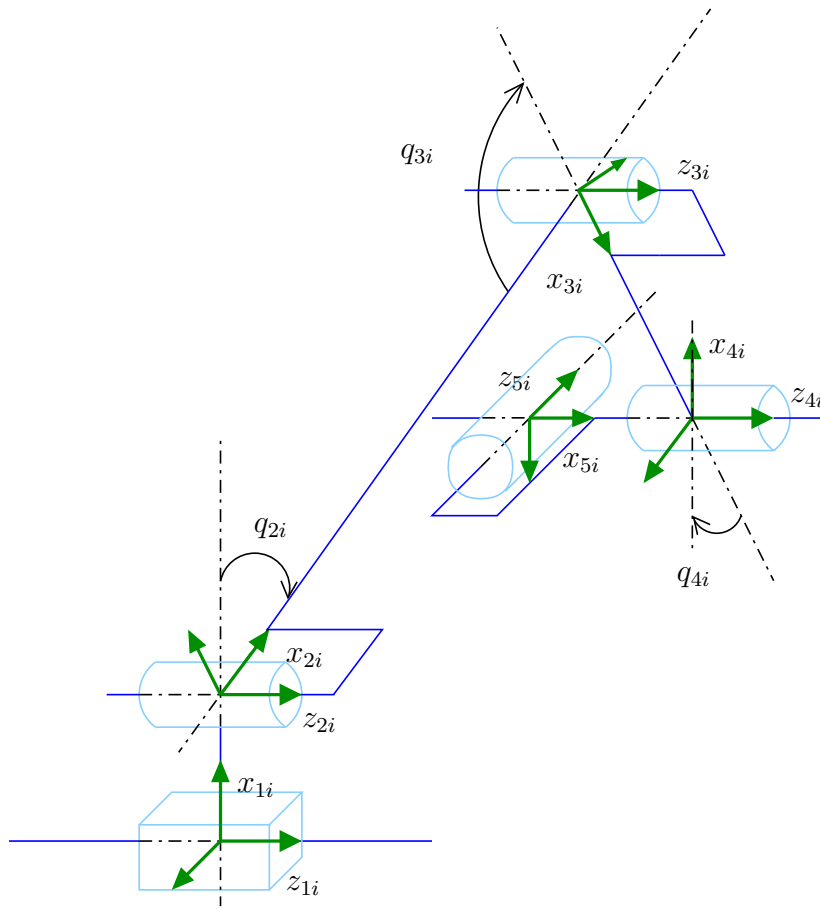
FIG. 3.4 – Schéma cinématique d'une jambe
