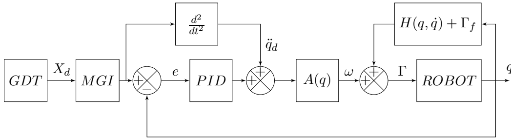
FIG. 1.14 – Commande en couple calculé dans l'espace articulaire
