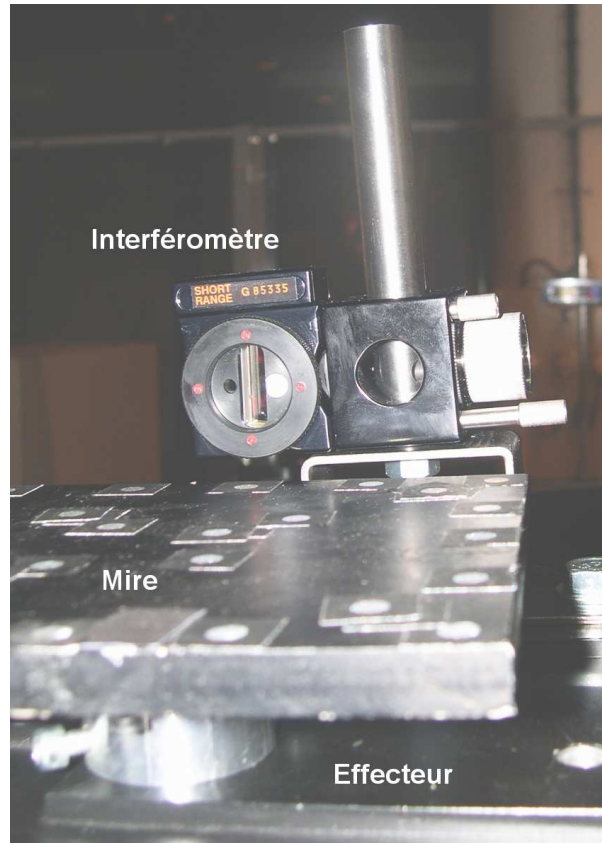
(a) Mire et interféromètre montés sur l'effecteur
