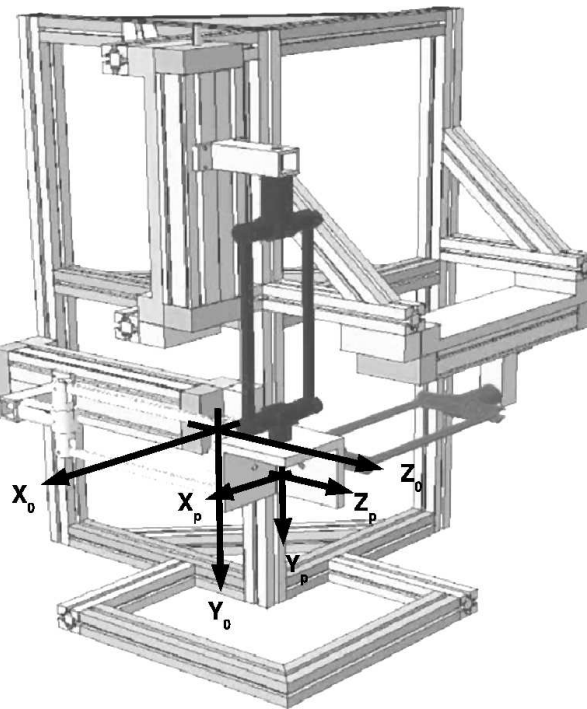
FIG. 3.8 – Schéma de l'Orthoglide [WC00]
