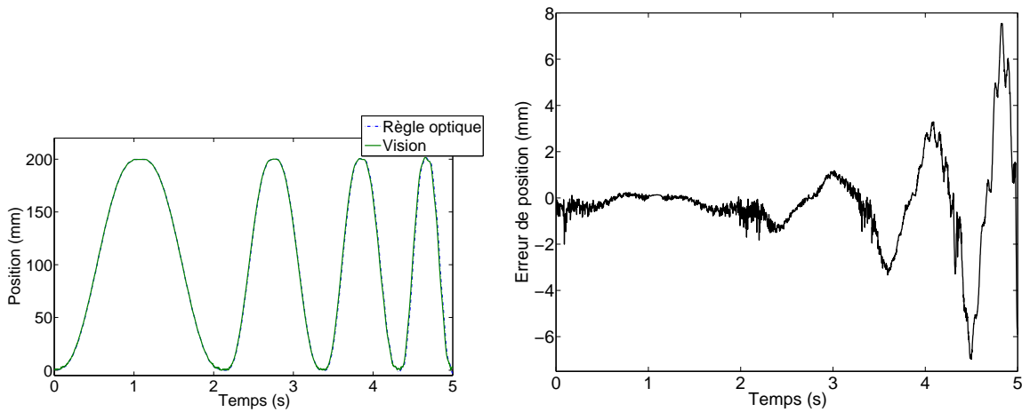
FIG. 3.31 – Comparaison entre la mesure visuelle à 500\text{Hz} et une règle linéaire optique à 1\mu\text{m} pour des accélérations allant de 1\text{ m.s}^{-2} à 10\text{ m.s}^{-2}
