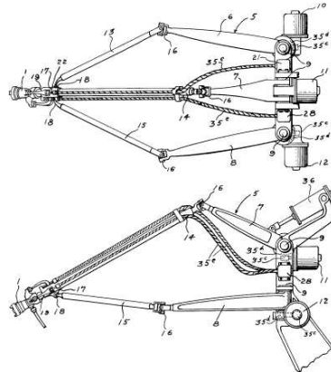
FIG. 1.2 – La machine à peindre de Pollard à 5 degrés de liberté [Pol42]
