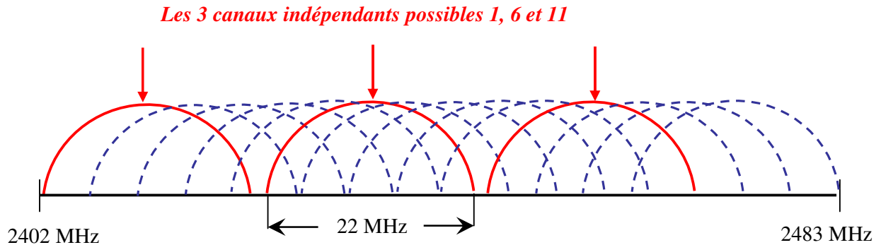
Figure 3.7. Recouvrement des canaux dans la bande ISM 2.4 GHz.
