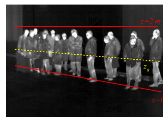
FIG. 3 – Le quai est modélisé par un plan 3-D du point de vue du capteur. La région d'intérêt est située entre les deux lignes z = 0 et z = 2\text{ m} . La ligne en pointillés représente le seuil de hauteur z_0 utilisé pour détecter les personnes à terre.
