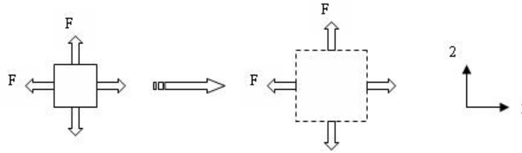
FIG. 2.3 – Traction équibiaxiale
