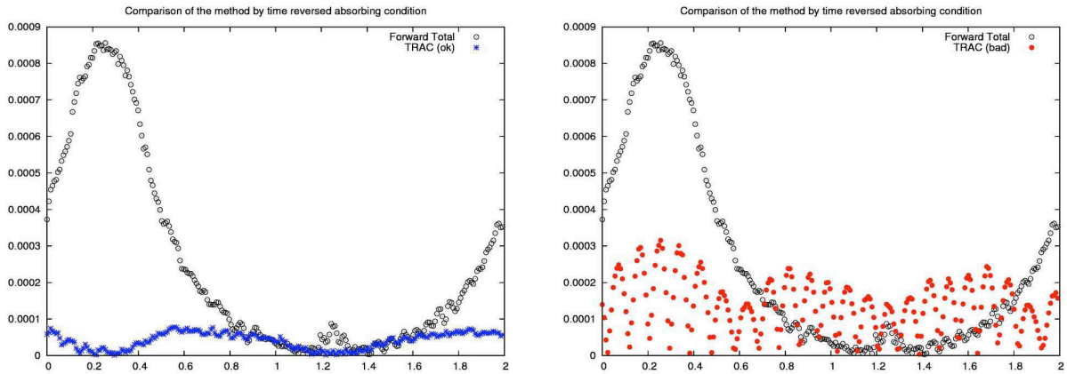
(c) Illustration du critère J_{ABC} : comparaison de \text{TRAC}(\hat{v}_R^T - \overline{\hat{u}^T}) (astérisque à gauche si D \subset B , point épais à droite si D \not\subset B ) et de \text{TRAC}(\overline{\hat{u}^T}) (cercle) le long de la frontière artificielle \Gamma_{J_{ABC}} .
