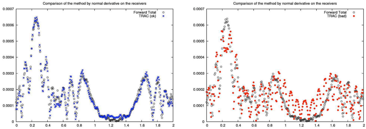
(b) Illustration du critère J_{DN} : comparaison des dérivées normales \partial \hat{v}_R^T / \partial n (astérisque à gauche si D \subset B , point épais à droite si D \not\subset B ) et \partial \overline{\hat{u}^T} / \partial n (cercle) le long de la ligne d'émetteurs-récepteurs.
