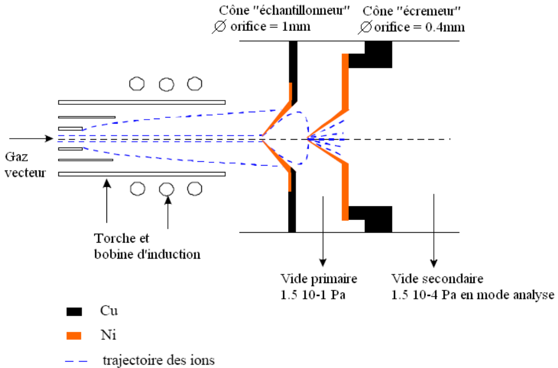
Figure II.12: Schéma de l'interface torche/quadripôle dans le cas de l'ICP-MS ThermoElemental X Series
