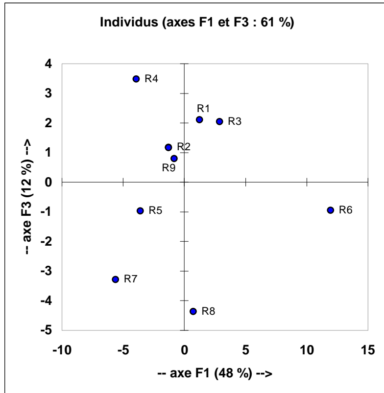
Figure III.8 : Répartition des observations dans le plan factoriel formé par les CP 1 et 3.
