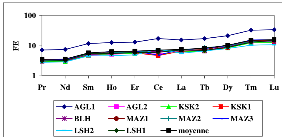
Figure III. 28 : Facteur d'enrichissement individuel et moyen dans la phase colloïdale de la rivière Bouregreg (cas des terres rares).
