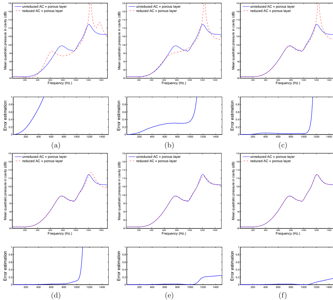
Figure A.20: Convergence - superposition des modes sélectionnés, \chi_{\max} = 0.4 : (a) Mode 1, (b) Modes 1, 2, 21; (c) Modes 1, 2, 21, 15; (d) Modes 1, 2, 21, 15, 4; (e) Modes 1, 2, 21, 15, 4, 12, 26; (f) Modes 1, 2, 21, 15, 4, 12, 26, 16
