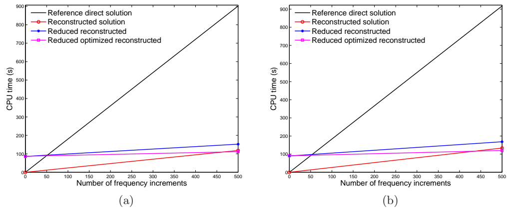
Figure A.22: Comparaison des temps de calcul avec reconstruction par approximants de Padé, problèmes non réduit, réduit, et réduit optimisé: (a) L = 3 , M = 4 ; (b) L = 5 , M = 6 .
