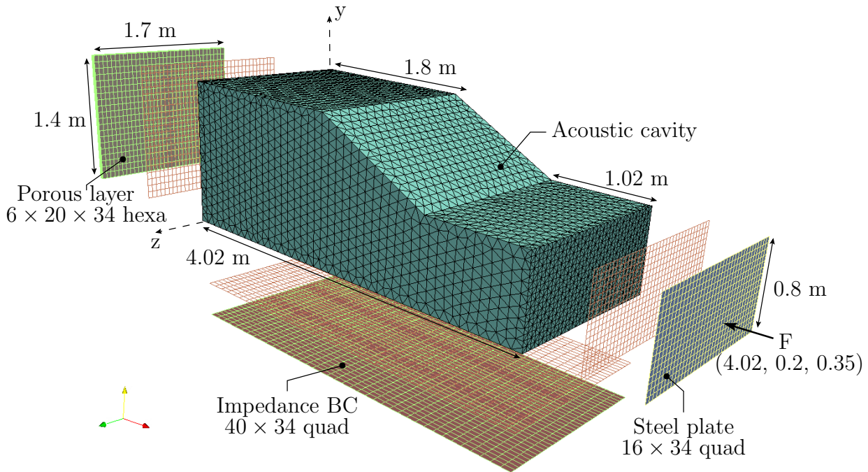
Figure A.23: Géométrie et maillage du modèle éléments finis.
