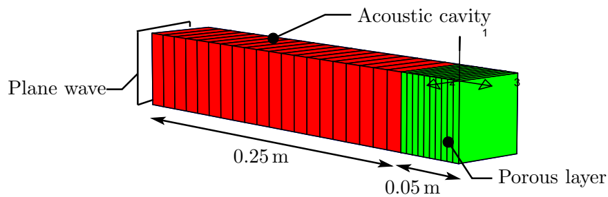
Figure A.9: Maillage et dimensions pour le problème 1D.
