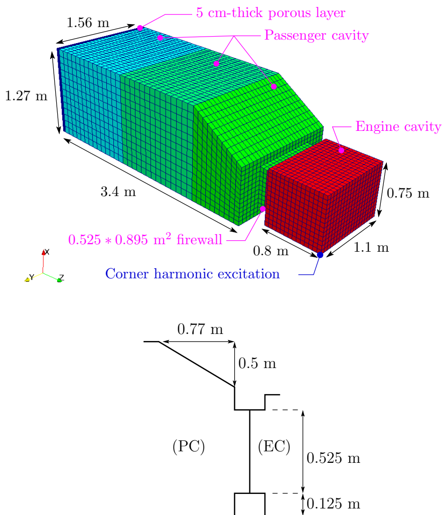
Figure A.4: Modèle EF Concrete car et dimensions extérieures.
