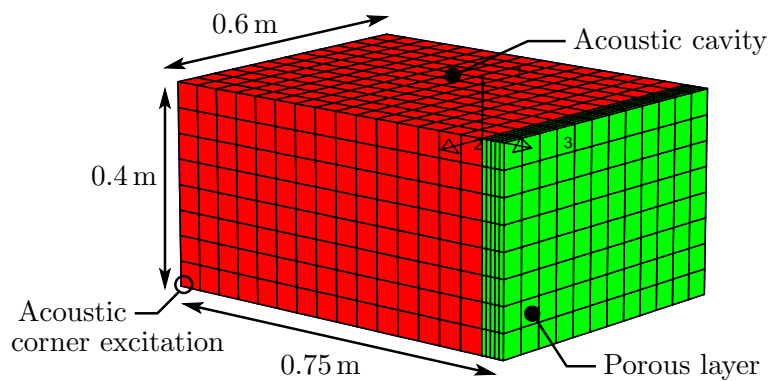
Figure A.12: Maillage et dimensions de la cavité 3D.
