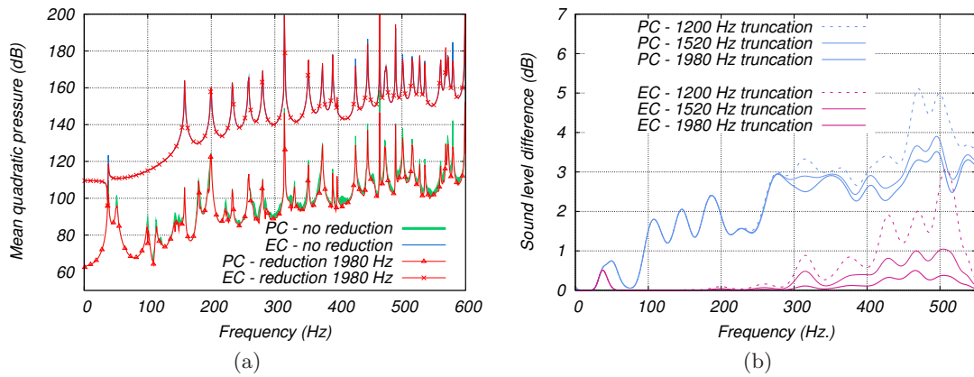
Figure A.6: Résultats avec troncature jusqu'à 1980 Hz: (a) FRF, pression quadratique moyenne; (b) différence (dB) à la solution du problème non réduit.
