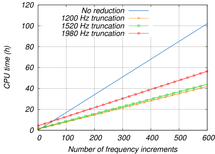
Figure A.7: Comparaison du temps de calcul, CPU.
