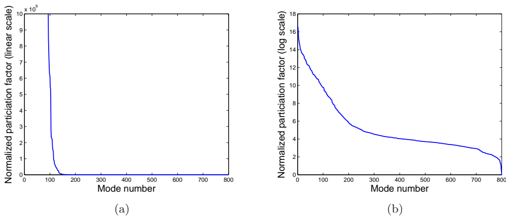
Figure A.16: Exemple de facteurs de participation modale normalisés: (a) échelle linéaire (b) échelle logarithmique.
