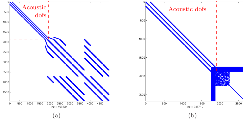
Figure A.14: Remplissage du système matriciel (a) non-réduit, (b) avec domaine poroélastique réduit.
