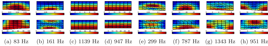
Figure A.19: Déformée des modes poreux 2D sélectionnés 1, 2, 21, 15, 4, 12, 26, 16: phases solide (haut) et fluide (bas). Maillage en configuration déformée et champ de déplacement.
