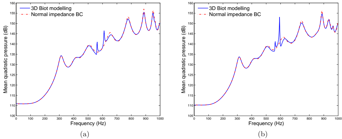
Figure A.2: Pression quadratique moyenne dans la cavité, modèle de Biot 3D ou par impédance localisée, Lz_p = 0.05 m: (a) (Lx_a, Ly_a, Lz_a) = (0.28, 0.4, 0.5) m; (b) (Lx_a, Ly_a, Lz_a) = (0.3, 0.4, 0.5) m.
