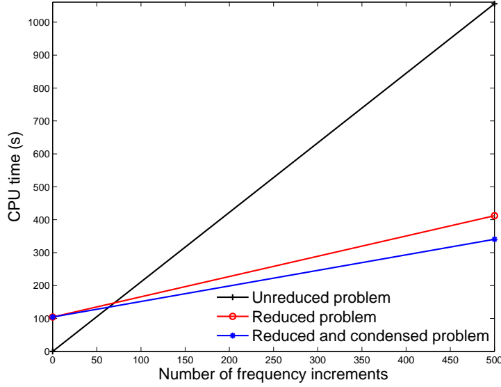
Figure A.15: Comparaison du temps de calcul, CPU, de fonctions de réponse en fréquence.
