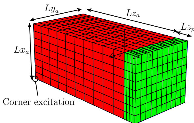
Figure A.1: Géométrie utilisée pour la comparaison entre modélisation 3D ou par impédance localisée pour un matériau poreux.
