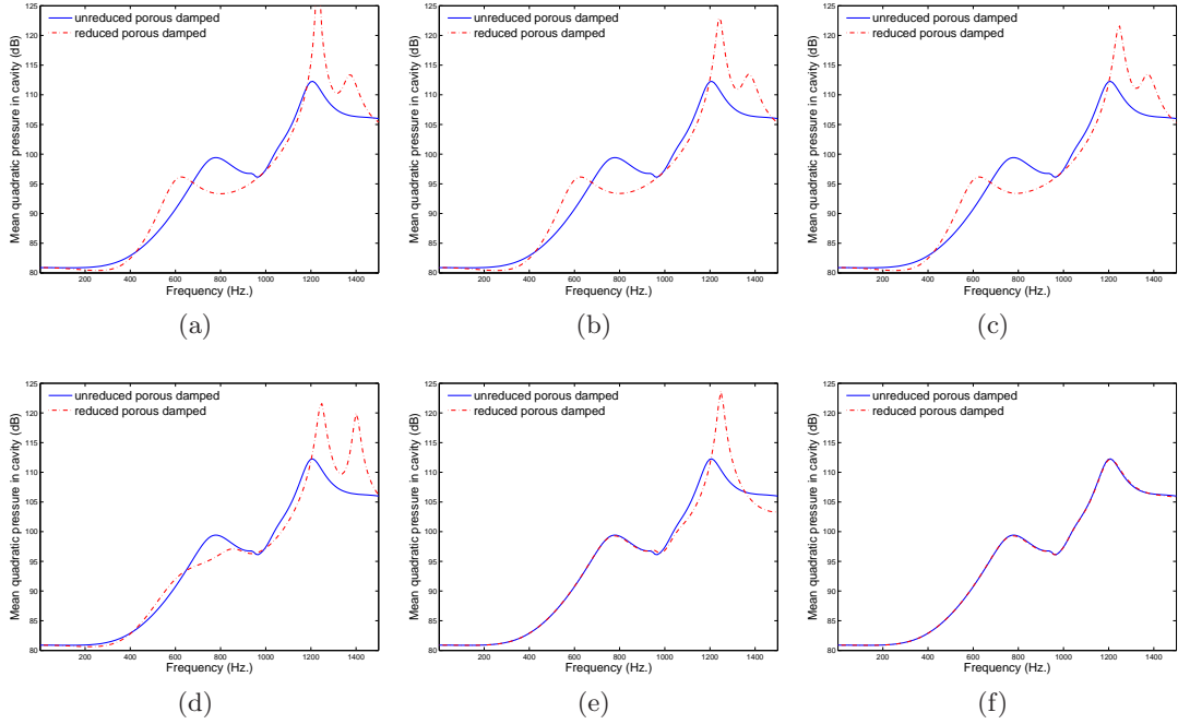
Figure A.18: Convergence - superposition des modes manuellement sélectionnés: (a) Mode 1, (b) Modes 1, 2; (c) Modes 1, 2, 4, 12; (d) Modes 1, 2, 4, 12, 15; (e) Modes 1, 2, 4, 12, 15, 16, 21; (f) Modes 1, 2, 4, 12, 15, 16, 21, 26
