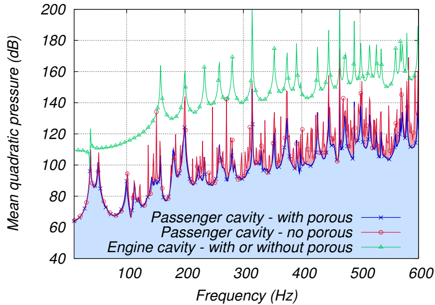
Figure A.5: FRF de référence avec et sans traitement poreux.
