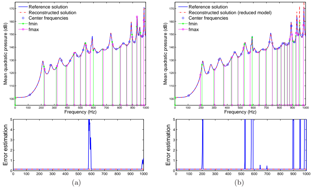
Figure A.21: Procédure de reconstruction adaptative de la réponse du problème 3D, avec L = 5 , M = 6 : (a) problème non réduit; (b) problème réduit.
