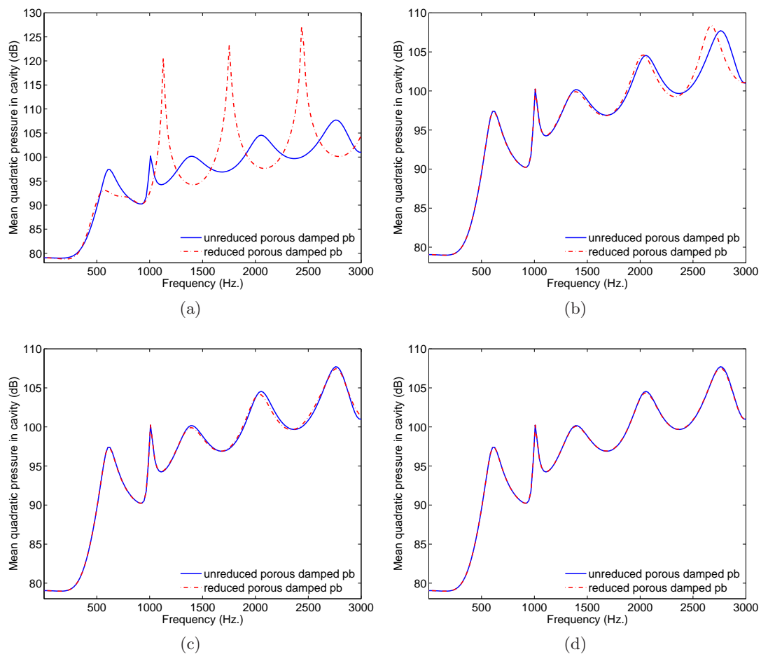
Figure A.10: FRF, pression quadratique moyenne: Convergence du modèle réduit vers la solution de référence: (a) 1 mode, (b) 2 modes, (c) 3 modes, (d) 4 modes.
