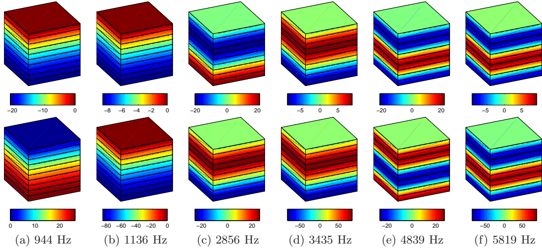
Figure A.11: Six premiers modes de la couche poreuse 1D: (a) – (f), phases solide (haut) et fluide (bas). Maillage et champ de déplacement.
