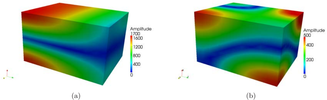
Figure A.3: Amplitude du champ de pression acoustique, (Lx_a, Ly_a, Lz_a) = (0.3, 0.4, 0.5) m, Lz_p = 0.05 m, à 593 Hz: (a) Modèle de Biot 3D pour le matériau poreux; (b) Condition limite d'impédance localisée.
