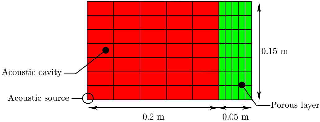
Figure A.17: Maillage et dimensions - problème 2D.
