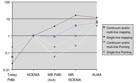
FIG. 1 – Vitesses relatives de différents instruments dont les caractéristiques sont définies dans le tableau ci-dessous, où D est le diamètre des antennes, N_{\text{ant}} le nombre d'antennes, N_{\text{bas}} le nombre de lignes de base, N_{\text{pix}} le nombre de pixels et B la bande passante totale disponible. La vitesse relative est définie comme l'inverse du temps qu'il faut pour atteindre la même sensibilité par point observé du ciel : en mode pointé, elle est proportionnelle à B N_{\text{bas}} D^4 ; en mode d'imagerie grand champ, elle est proportionnelle à B N_{\text{pix}} N_{\text{bas}} D^2 . Les vitesses ont été normalisées par les performances de NOEMA.
