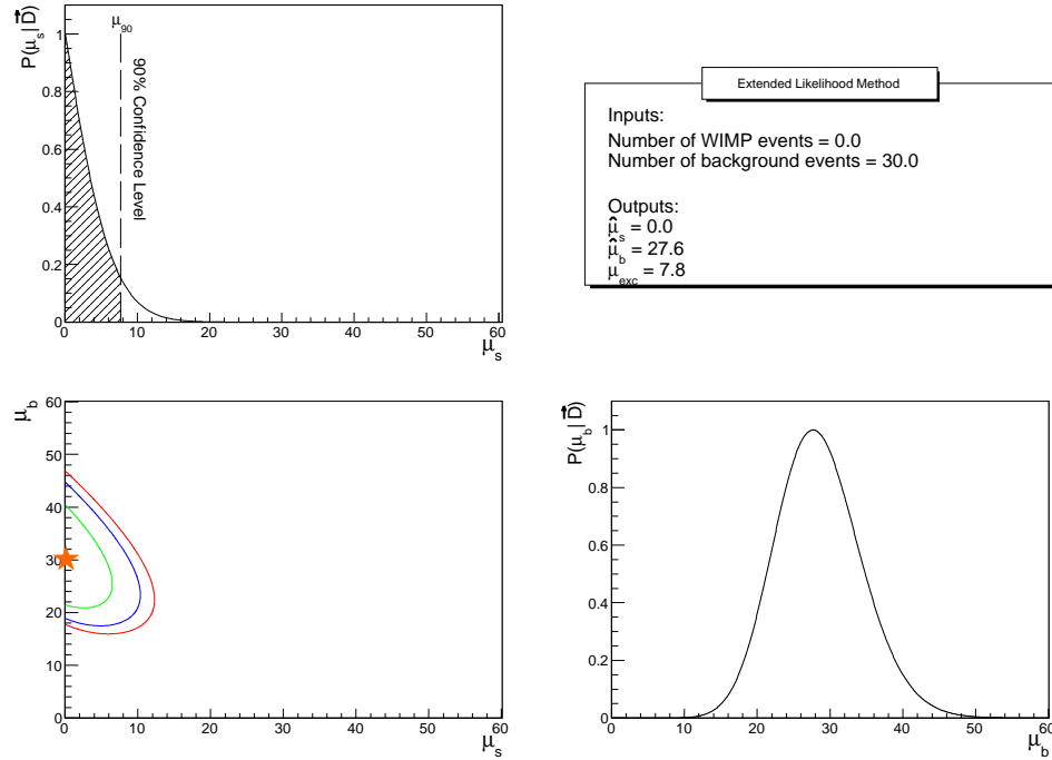
FIGURE 4.2 – Représentation de \mathcal{L}(\mu_s, \mu_b) dans le cas où \mu_s = 0 et \mu_b = 30 . En bas à gauche : représentation à deux dimensions de la fonction de vraisemblance dans le plan (\mu_s, \mu_b) avec les contours de confiance à 68%, 90% and 95%. L'étoile orange représente les valeurs d'entrée des paramètres \mu_s et \mu_b . Les panneaux en haut à gauche et en bas à droite représentent les distributions marginalisées P(\mu_s|\vec{D}) et P(\mu_b|\vec{D}) respectivement. La limite \mu_{90} correspond à la borne supérieure du niveau de confiance à 90% sur le nombre d'événements WIMP exclus. On trouve dans ce cas que \mu_{exc} = 7,8 à 90% de confiance. Figure extraite de [165].
