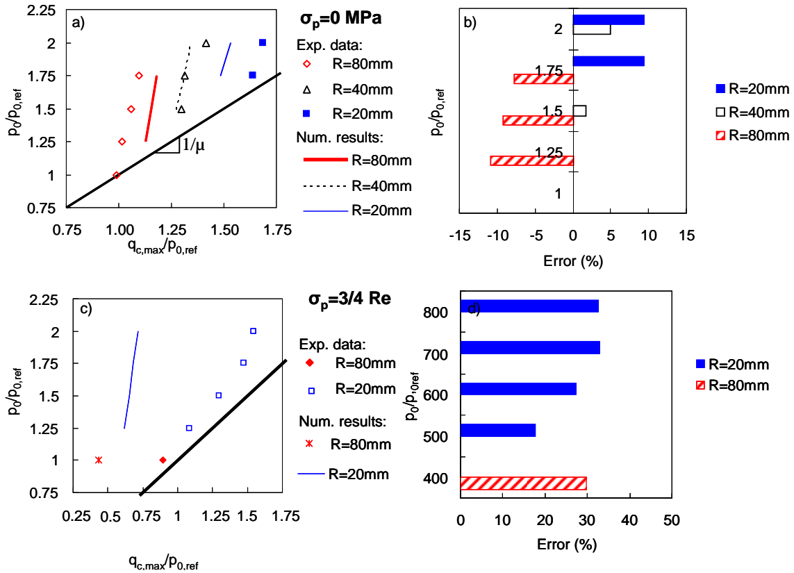
Figure IV-16 : comparaison entre la carte de fretting expérimentale et calculée par la méthode appliquée dans [Fouvry, 1996, 2004] et écarts entre les calculs et les résultats expérimentaux. a) et b) sans précontrainte, c) et d) avec précontrainte.
