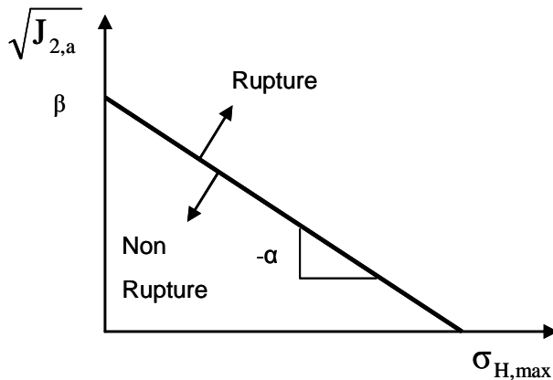
Figure II-4 : Diagramme représentant les domaines de rupture et non-rupture d'après le critère de Crossland
