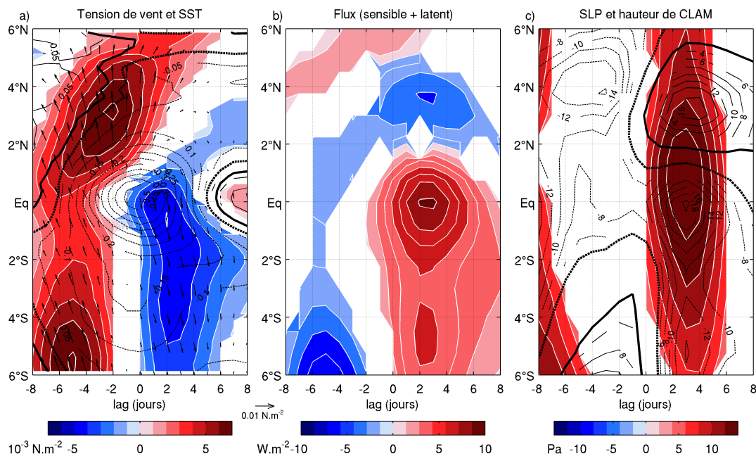
Figure 35 – Régressions linéaires sur le NCTI du lag -8 à +8 jours, de (a) la tension de vent QuikScat (couleurs, 10^{-3} \text{N.m}^{-2} ) et la SST TMI (contours, ^{\circ}\text{C} ), (b) la somme des flux de chaleur latente et sensible ( \text{W.m}^{-2} , négatif vers le haut), et (c) la SLP (couleurs, Pa) et la hauteur de CLAM (contours, m) ERA-Interim, moyennées entre 10°O et 6°E, entre avril et juillet 2000 à 2009. Les contours plus épais délimitent les zones significatives.
