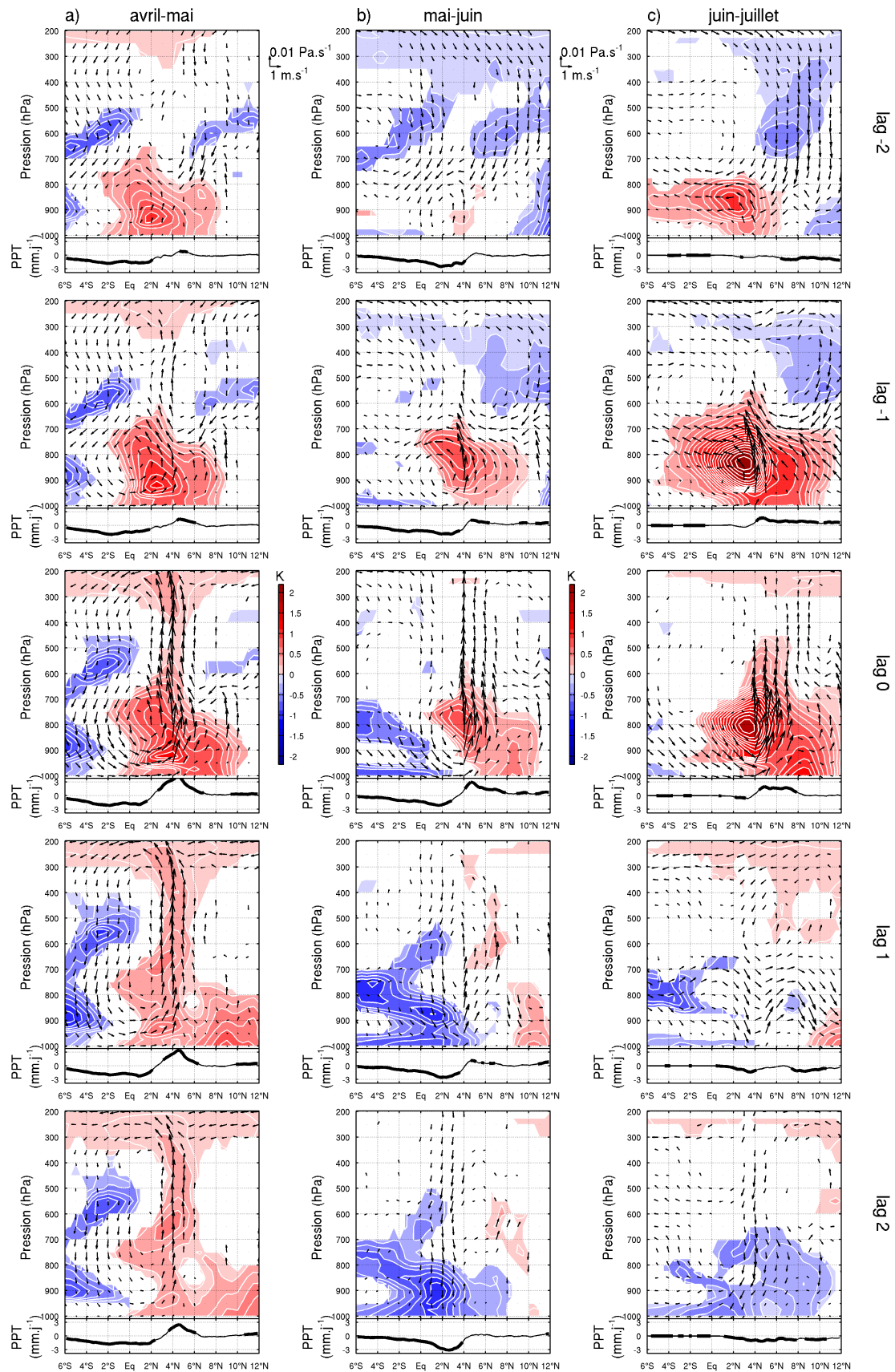
Figure 36 – Régressions linéaires sur \tau_\gamma -index avec lags de -2 à +2 jours, de \theta_e (couleurs, K) et du vent (flèches) CFSR ainsi que des précipitations TRMM (courbes), en (a) avril-mai, (b) mai-juin et (c) juin-juillet, entre 10-6°O. Seules les valeurs significatives à 10 % sont représentées.
