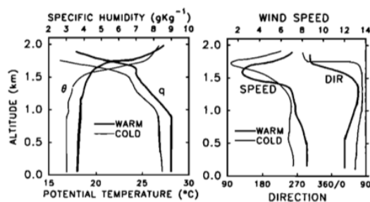
Figure 13 – Profils moyens de part et d'autre d'un front de SST dans l'Atlantique Nord - campagne FA-SINEX : (gauche) température potentielle ( ^{\circ}\text{C} ) et humidité spécifique ( \text{g.kg}^{-1} ); (droite) vitesse ( \text{m.s}^{-1} ) et direction ( ^{\circ} ) du vent. D'après Friehe et al. [1991].
