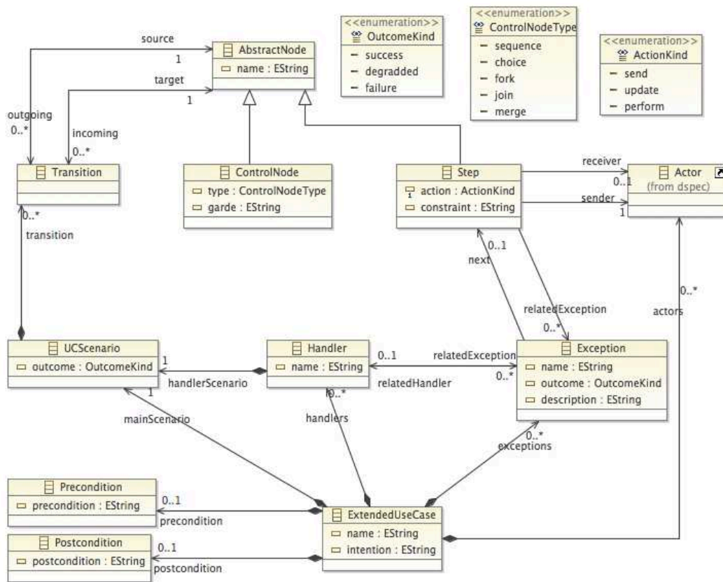
Figure 5.4 : Métamodèle des XUC
