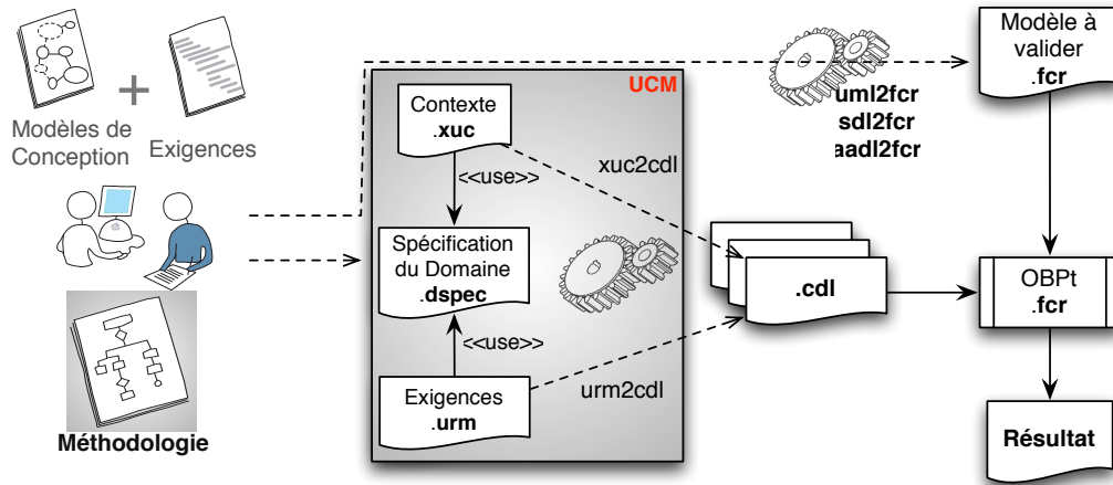
Figure 1.3 : Composant UCM pour la génération de modèles CDL
