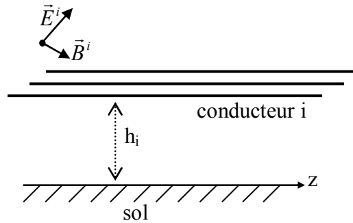
Figure III.4. Ligne aérienne illuminée par une onde électromagnétique.
