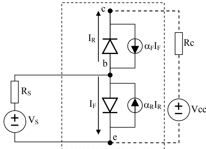
Figure II.16. Modèle de Ebers-Moll pour un transistor à jonction bipolaire.
