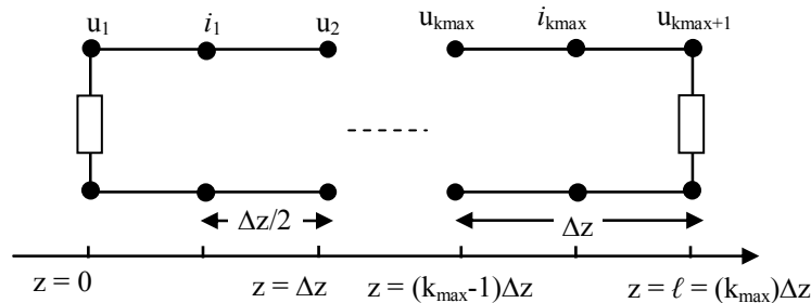
Figure III.5. Discrétisation des courants et tensions par FDTD sur une ligne.
