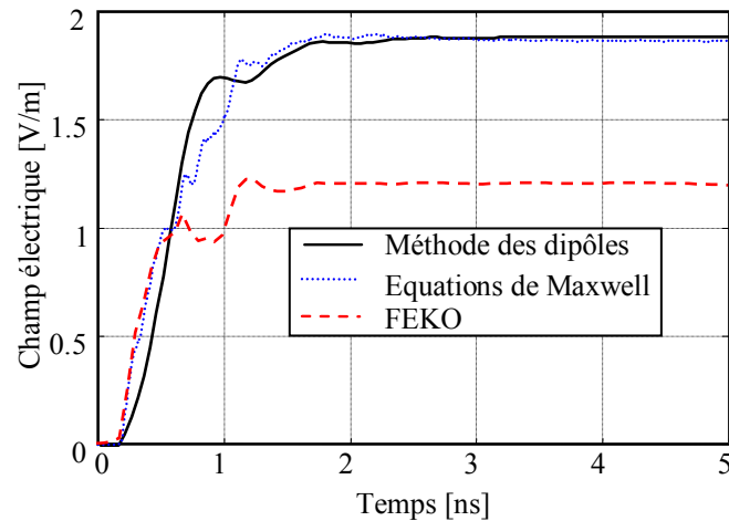
Figure IV.8. Champ électrique émis par le circuit sans plan de masse.
