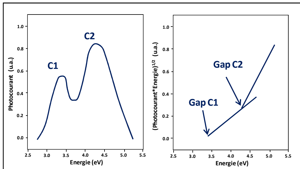
Figure II-12 : Allure typique d'une photocaractéristique en énergie composée de 2 contributions semi-conductrices obtenue lors de l'analyse par PEC d'un oxyde (à gauche), et transformée linéaire associée permettant d'obtenir la valeur de gap associée à chaque contribution (à droite) [209].
