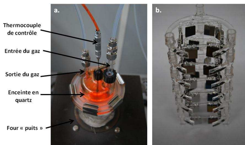
Figure II-9 : a. Photographie du dispositif des essais de longues durées ; b. photographie des nacelles en quartz supportant les échantillons.
