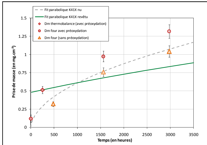
Figure VI-19 : Variation du gain de masse mesuré pour les échantillons d'alliage K41X revêtus d'un dépôt de \text{La}_2\text{O}_3 (avec ou sans préoxydation), exposés sous air sec à 800\text{ }^\circ\text{C} pendant 480, 1560 et 2976 heures. Le gain de masse final obtenu en thermobalance après 250 heures d'essai pour un échantillon revêtu (avec ou sans préoxydation) est également ajouté. Les fits paraboliques associés aux courbes thermogravimétriques obtenues en thermobalance avec et sans dépôts ont été ajoutés pour comparaison.
