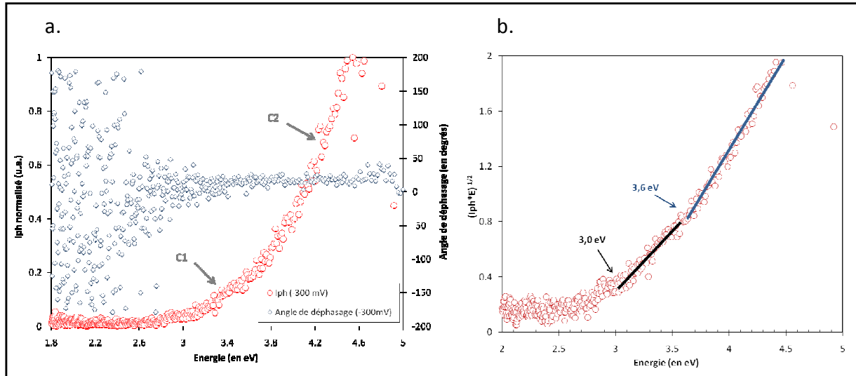
Figure IV-17 : a. Evolution du photocourant en fonction de l'énergie du rayonnement incident, pour un échantillon d'alliage K41X oxydé après 250 heures à 800 °C sous Ar-1\%H_2-9\%H_2O , polarisé à -300 mV. L'évolution de l'angle de déphasage est également indiquée b. Transformées linéaires de la photocaractéristique en énergie mettant en évidence les différentes transitions contribuant à l'intensité du photocourant.
