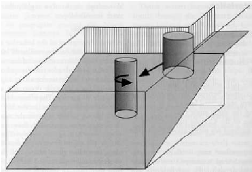
FIG. 1.2 – Étirement de colonnes de fluide (Lane-Serff, 2001).
