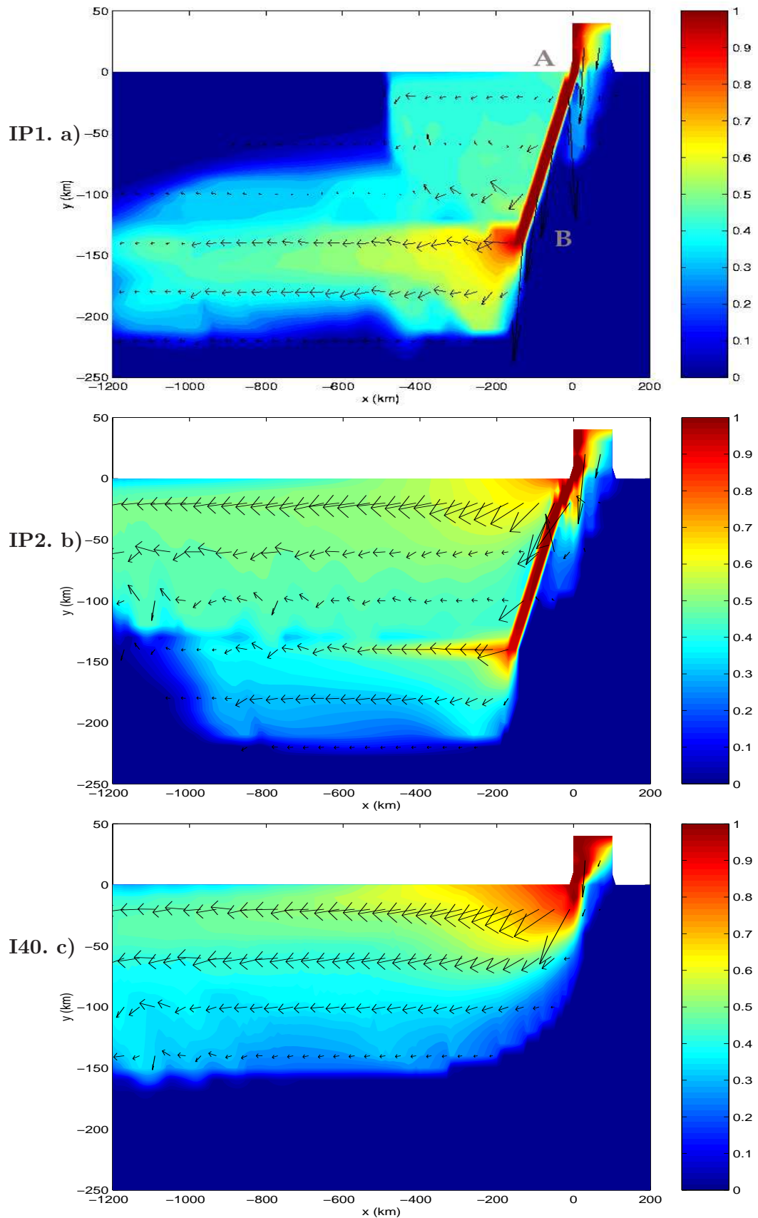
FIG. 6.10 – Concentration de traceur passif au-dessus de la topographie après 60 jours d'intégration et vecteurs vitesses pour les 3 profils topographiques de la configuration DOME montrés en figure 6.9,b dans des expériences avec BBL. Le profil dit P1 "falaise" est montré an a), le profil P2 en b), et le profil linéaire en c).
