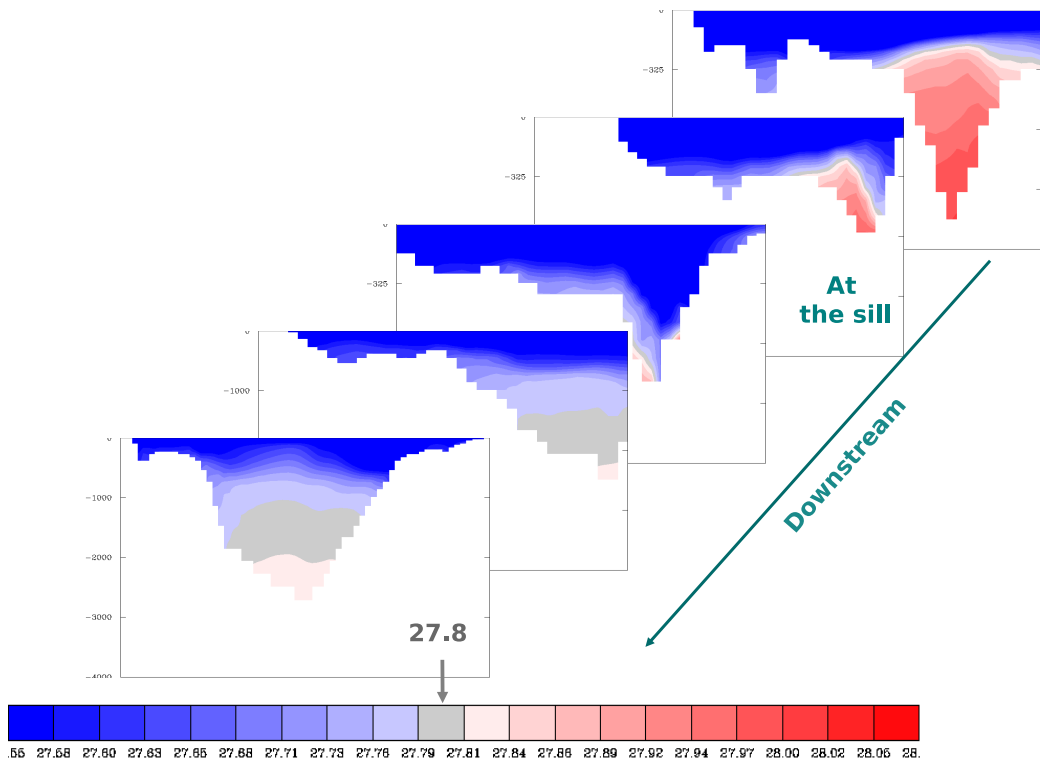
FIG. 3.7 – Evolution de la densité potentielle moyennée entre 1990-2000 à différentes sections (de haut en bas à 67^\circ N , 66.5^\circ N , 66^\circ N , 65^\circ N et 64^\circ N ) du Détroit du Danemark obtenue par la configuration ORCA025 (NEMO 11). On remarque que les eaux de fond, très denses en amont du seuil (à 67^\circ N ) perdent rapidement leur forte densité en aval.
