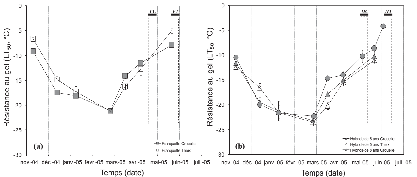
Figure II.3 : Variation au cours du temps de la résistance au gel des rameaux d’un an, pour 2 cultivars de noyer (‘Franquette’ (F) (a) et Hybride NG38 (H) (b) sur 2 sites expérimentaux (Crouelle (C) et Theix (T)). L’échantillonnage a été réalisé du 8 novembre 2004 au 24 mai 2005. Les barres d’erreur représentent l’erreur standard (n = 5). Les barres horizontales et les rectangles en pointillé indiquent les périodes de débourrement des arbres.
