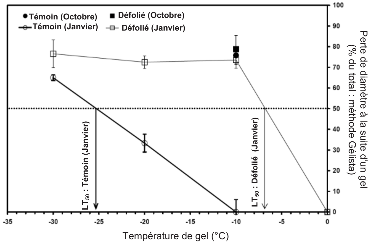
Figure I.4 : Estimation de la résistance au gel (LT 50 ) par la méthode Gélista™ pour deux traitements (témoin et défolié) et pour deux dates (Octobre et Janvier). La perte de diamètre, représentée par le pourcentage (du total) de perte de diamètre à la suite d'un cycle à la température de gel testée, est présentée. Pour chaque température testée, la moyenne et l'erreur standard sont indiquées (n=3).
