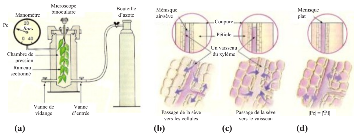
Figure m.13 : (a) Schéma d'une chambre de pression. (b), (c) et (d) Schéma explicatif du principe de la chambre de pression (extrait de Cruiziat et Tyree (1990)).
