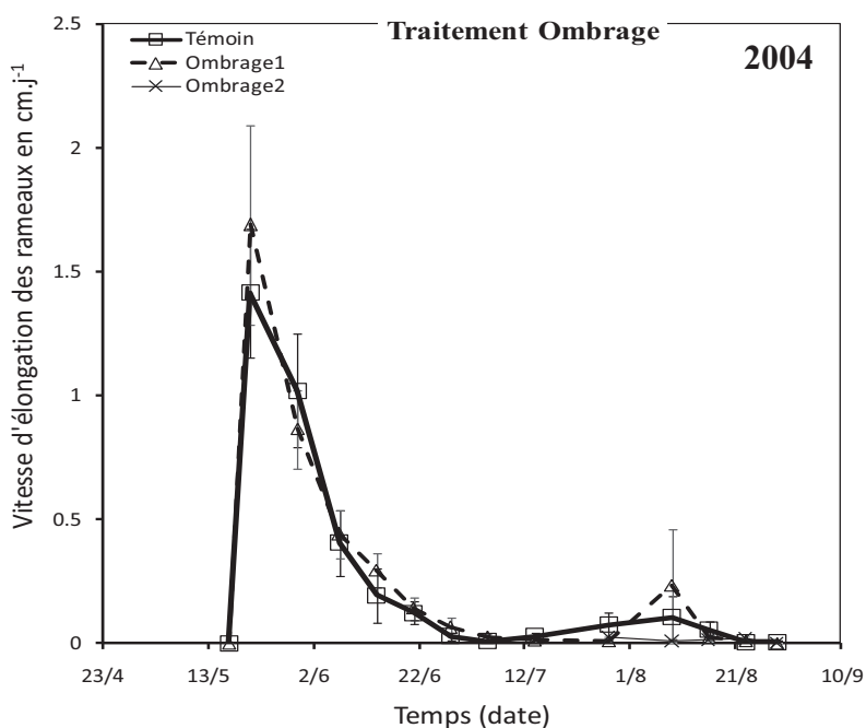
Figure III.21 : Evolution de la vitesse d’élongation des rameaux d’arbres subissant les traitements d’ombrage (moyenne ±SE ; n=6).
