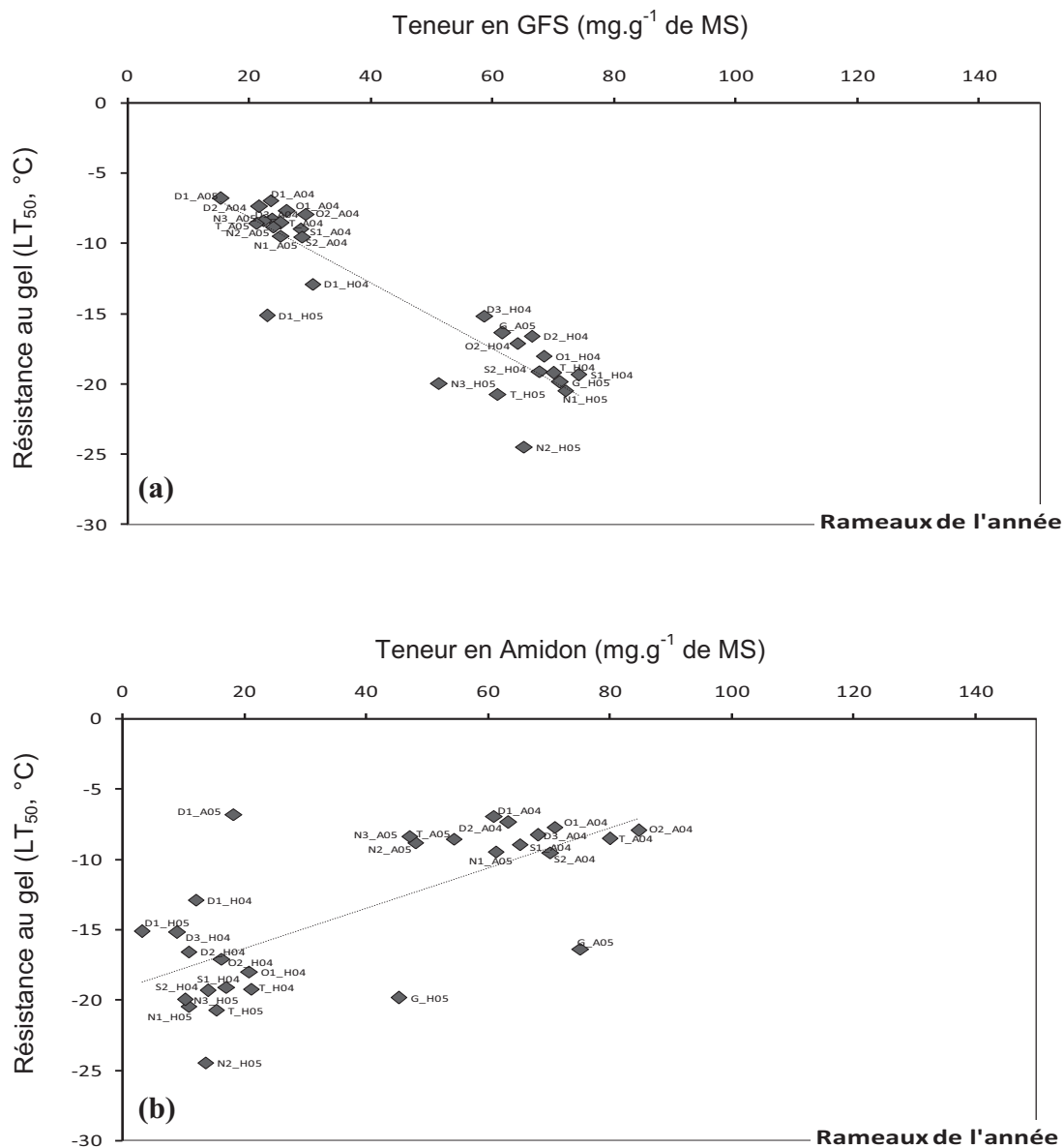
Figure III.B.6 : Régression linéaire entre la résistance au gel ( LT_{50} ) et les teneurs en sucres solubles (GFS) (a) ou en amidon (b) des rameaux de l'année de jeunes noyers en conteneur.
