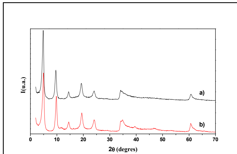
Fig. 10 : Diffractogrammes de la phase [Zn-Al-SPMA] synthétisée par échange avec [Zn-Al-Cl] : a) H'(A) ; b) H''(A)
