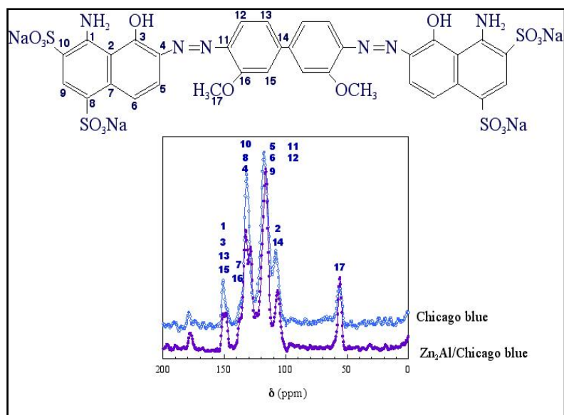
Fig. 17 : ^{13}\text{C} -CP-MAS RMN: de Chicago bleu et \text{Zn}_2\text{Al}/\text{Chicago}
