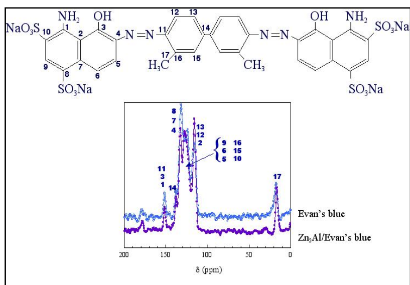
Fig. 18 : ^{13}\text{C} -CP-MAS RMN: de Evans bleu et \text{Zn}_2\text{Al}/\text{Evan}
