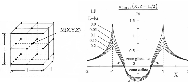
Figure I.17: Illustration de l'effet d'échelle introduit par Fouvry [Fouvry et al. (1998)]: les gradients de contraintes sont d'autant plus atténués que le volume de matière considéré est grand.
