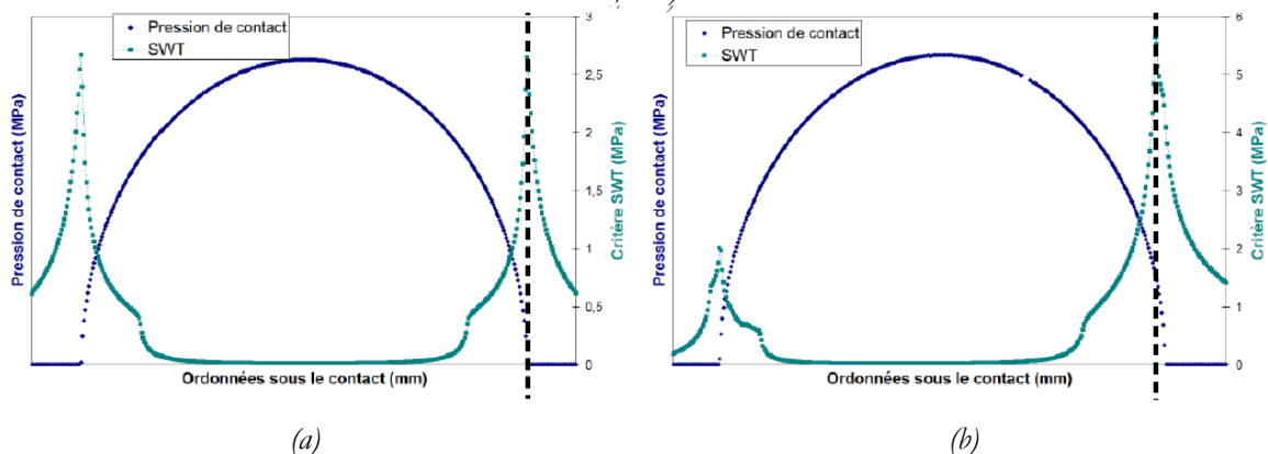
Figure V.7: Profils de pression sous le contact superposés au profil SWT, localisation du point de critère maximal dans le cas de l'essai (a) fretting simple ( Q = xxx N/mm) et (b) de l'essai fretting fatigue ( Q = xxx N/mm, \sigma = 350 MPa).
