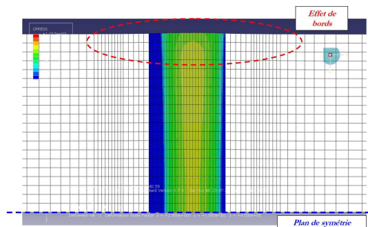
Figure xxix: Représentation des pressions de contact avec le modèle 3D: visualisation du plan de symétrie du modèle et de l'effet de bords.
