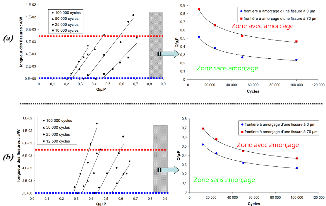
Figure IV.2: Détermination des condition d’amorçage des fissures pour la contact (a) cylindre/plan et (b) plan/plan : espace \{a/W, Q/\mu_t P\} et courbes de Whöler à amorçage en fretting correspondantes.
