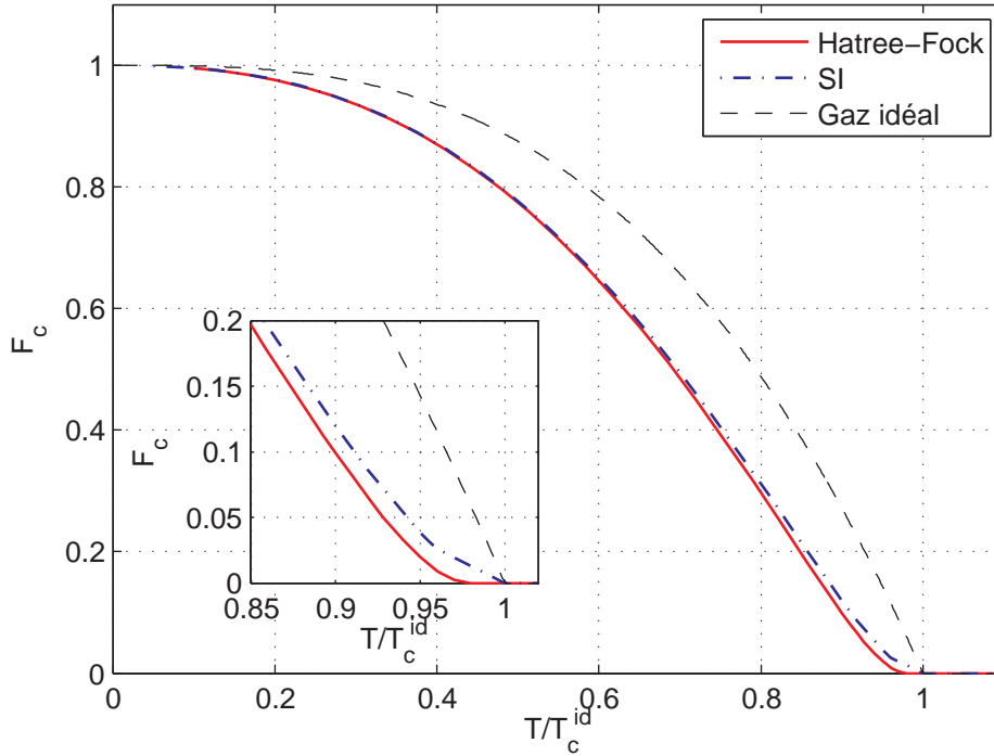
FIGURE 1.2 – Comparaison des fractions condensées pour un gaz sans interactions (ligne tiretée noire) et un gaz en interactions (ligne continue rouge : modèle Hartree–Fock complet, ligne tiretée bleue : modèle semi-idéal), pour N = 3300 atomes de sodium dans un piège de fréquence moyenne \bar{\omega} = 2\pi \times 1.1 kHz.
