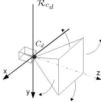
FIGURE 1.5: Modèle cinématique simplifié d'une caméra dynamique, [29]. Les axes de rotation en azimuth et en site, représentés par des flèches sur la figure, sont modélisés tels qu'ils soient alignés avec le centre optique.
