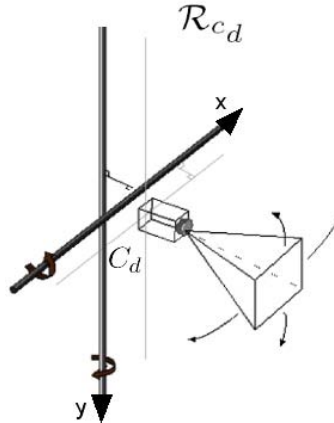
FIGURE 1.6: Modèle cinématique généralisé d'une caméra dynamique, [29]. Le mouvement en azimuth et en site, représentés par des flèches sur la figure, est modélisé comme des rotations autour d'axes de direction arbitraire dans l'espace.
