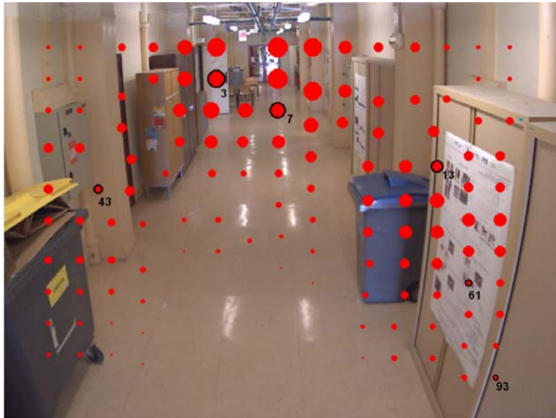
FIGURE 3.5: Quadrillage d'apprentissage lors du calibrage. Les points cerclés de noirs servent de base à la discussion sur la précision du calibrage. La taille des cercles représentent la densité de points SIFT extraits dans leurs voisinage.
