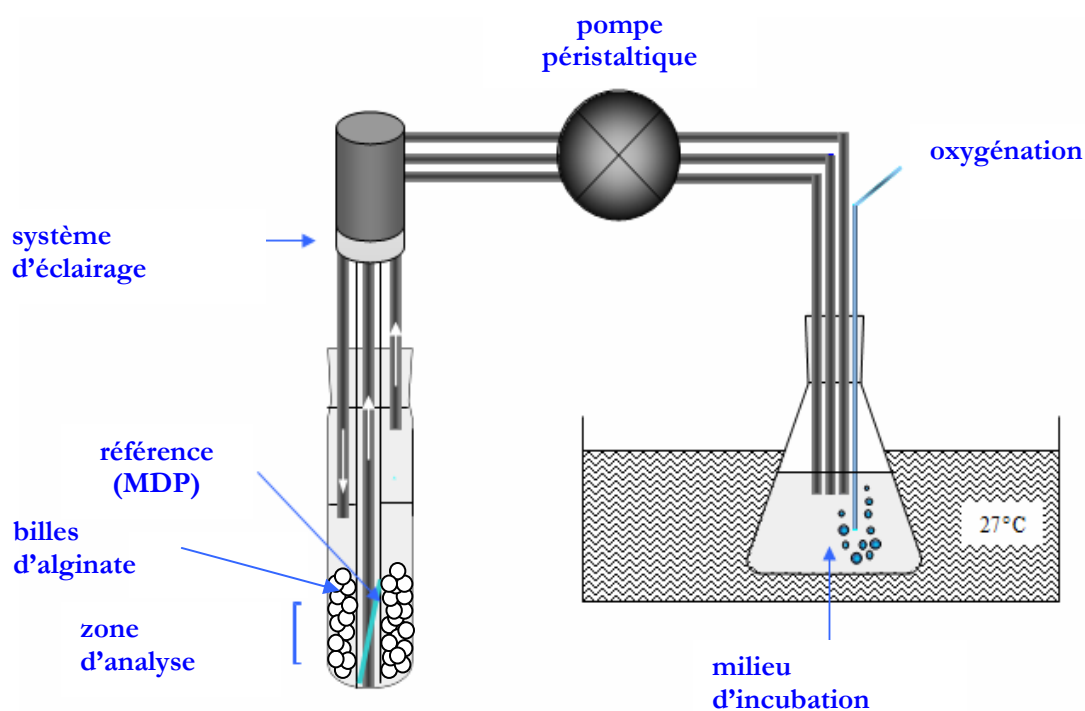
Figure 86 Schéma du système de perfusion mis en place pour réaliser la RMN ^{31}\text{P} in vivo (avec système d'éclairage pour les expériences réalisées au CEA de Grenoble- sans éclairage pour celles réalisées au SEESIB à Clermont-Ferrand)
