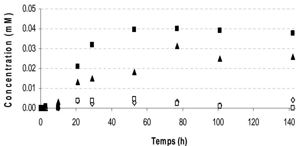
Figure 101 Evolution de la concentration en 6OHABT avec le temps lors de la biodégradation de l'ABT (0,5 mM). (△) cellules immobilisées + hv ; (▲) cellules immobilisées - hv ; (□) cellules libres + hv ; (■) cellules libres - hv
