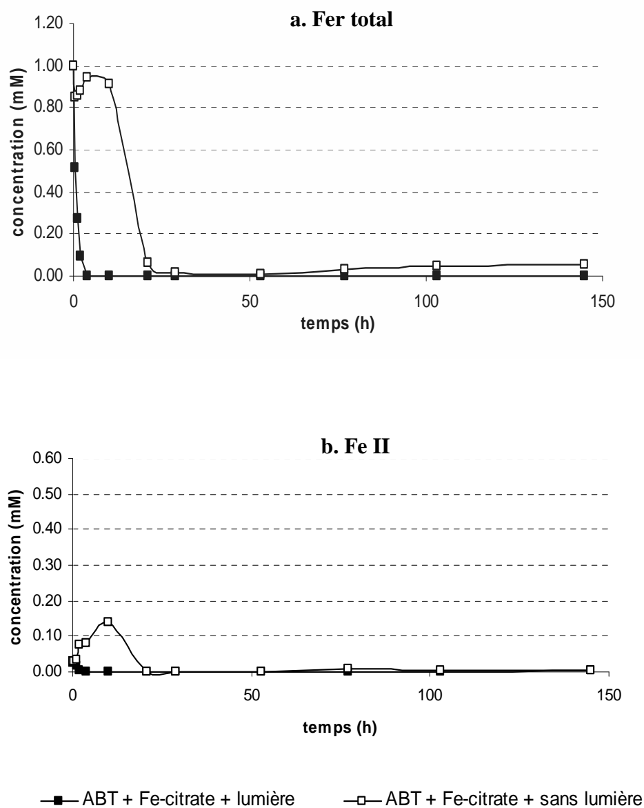
Figure 151 Evolutions des concentrations en fer total (a) et en Fe(II)(b) lors de la biodégradation d'ABT (0,5 mM) en présence du complexe Fe-citrate (1 mM), avec ou sans lumière
