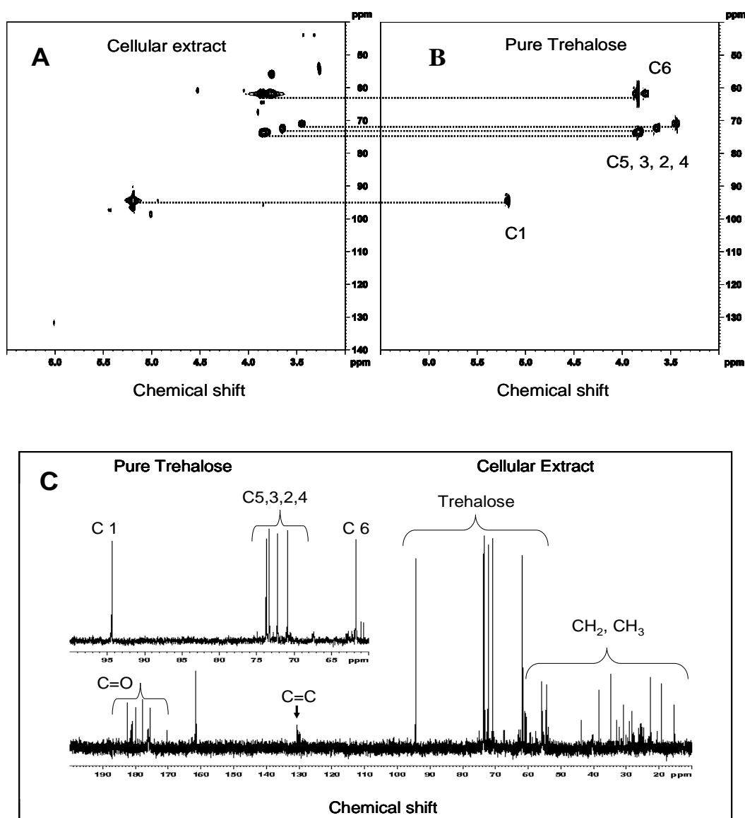
Figure 122 Spectres de RMN 2D HSQC ^1\text{H} - ^{13}\text{C} (A) des extraits cellulaires de Rhodococcus rhodochrous OBT18 obtenus après incubation avec du glucose marqué [ ^{13}\text{C} ] pendant 118 h ; (B) du tréhalose commercial pur ; (C), spectre de RMN 1D ^{13}\text{C} des extraits perchloriques de Rhodococcus rhodochrous OBT18 avant l'addition de glucose [ ^{13}\text{C} ], les signaux du tréhalose pur sont présentés en insert.
