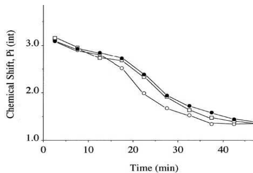
Figure 64 Evolution du déplacement chimique du signal du Pi avec le temps chez Escherichia coli , souche sensible. Cercles pleins, témoin ; cercles ouverts, cellules en présence de tellurite ; carrés ouverts, cellules en présence de sélénite. (Lohmeier-Vogel et al., 2004)
