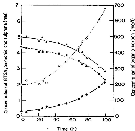
Figure 5 Concentration de différents éléments lors de la biodégradation du BTSO 3 par des boues activées (▲) BTSO 3 ; (●) ammonium; (○) sulfate; (■) carbone organique (d'après Mainprize et al., 1976)
