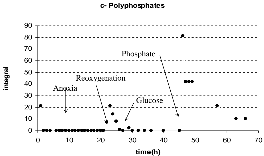
Figure 119 Evolutions de différents marqueurs de l'énergétique cellulaire de R. rhodochrous lorsqu'elle est soumise à différentes conditions. (a) évolution du déplacement chimique du Pi ; (b) évolution des valeurs des intégrales du \beta -ATP ; (c) évolution des valeurs des intégrales des polyphosphates
