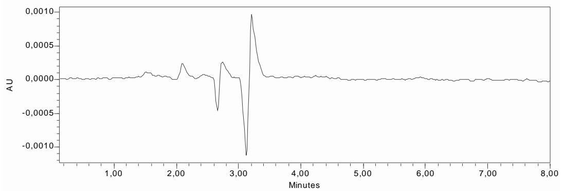
Figure 98 Chromatogramme après dépôt de 1 ml d'une solution de 6OH-ABT à 0,5 mM
