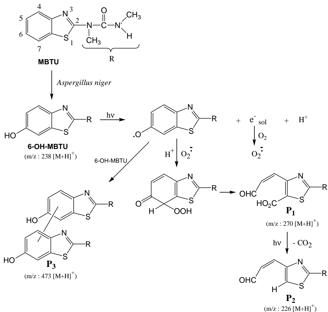
Figure 16 Dégradation du MBTU – proposition du mécanisme réactionnel mis en jeu
