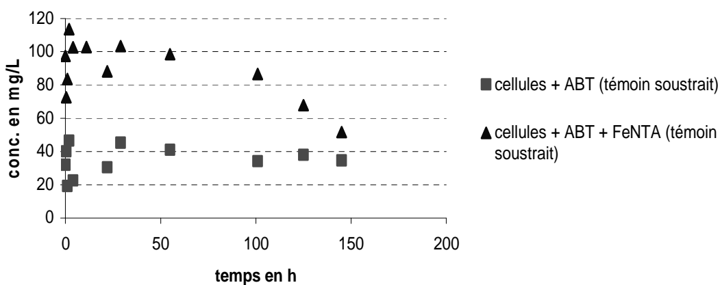
Figure 112 Evolution de la concentration en carbone organique total prenant en compte le témoin cellules lors des expériences (■) avec cellules + ABT (0,5 mM) et (▲) avec cellules + ABT (0,5 mM) + FeNTA (1 mM)
