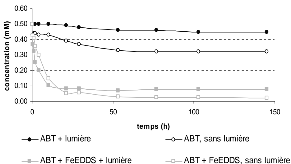
Figure 138 Dégradation de l'ABT (0,5 mM) par R. rhodochrous en présence ou en absence du complexe FeEDDS (1mM), avec ou sans lumière
