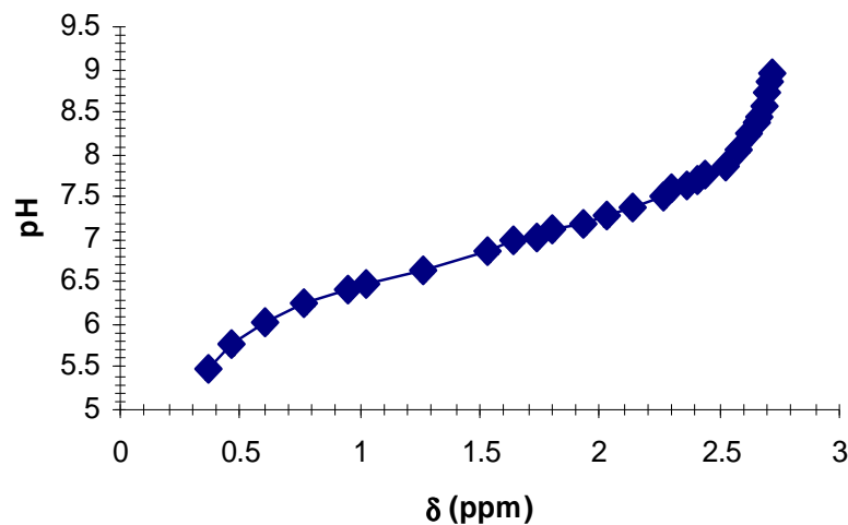
Figure 62 Variation du déplacement chimique du Pi en fonction du pH - Expérience réalisée avec Rhodococcus rhodochrous
