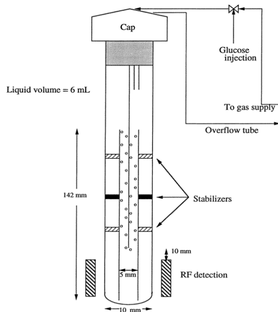
Figure 58 Système mis en place pour une étude RMN en condition aérobie (Grivet et Delort, 2008)
