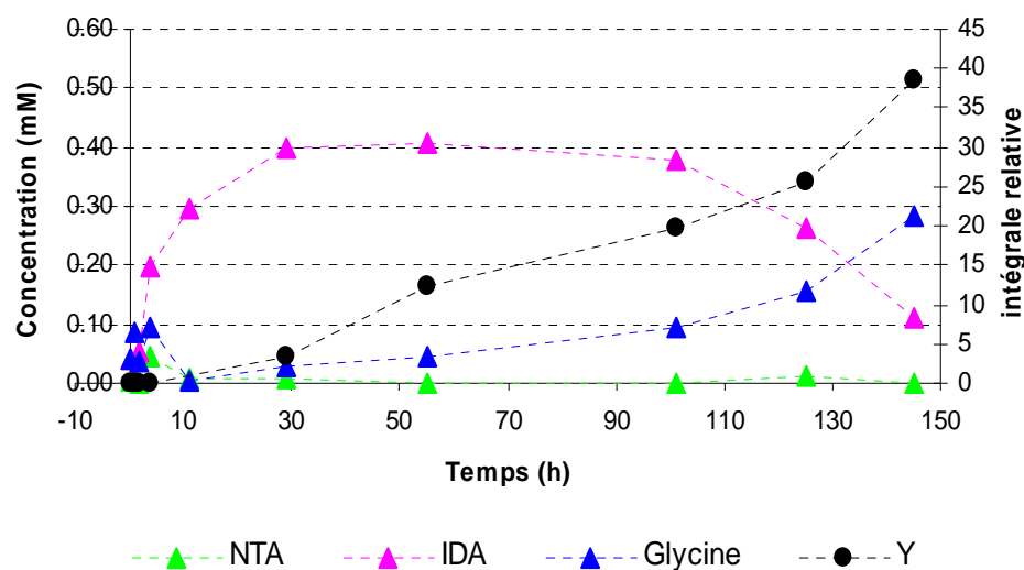
Figure 136 Evolutions des concentrations en NTA après décomplexation, IDA, glycine et de l'intégrale relative de Y d'après l'intégration de spectres RMN 1 H au cours de l'incubation de R. rhodochrous et de l'ABT (0,5 mM) avec le complexe FeNTA (1 mM) en absence de lumière
