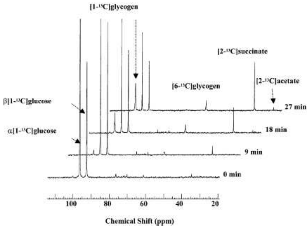
Figure 68 Spectres réalisés in vivo et mettant en évidence l'utilisation du [1- 13 C]glucose par des cellules en repos de F. succinogenes S85 (Matheron et al., 1997)
