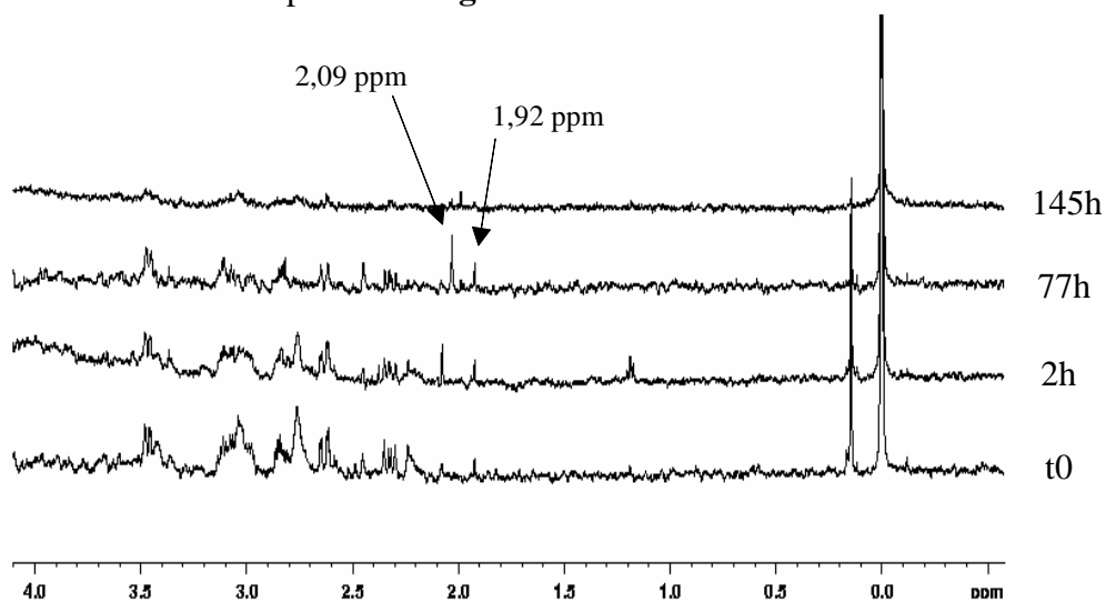
Figure 146 Spectres RMN 1 H montrant l'évolution du FeEDDS (1 mM) lors de la biodégradation de l'ABT à l'obscurité
