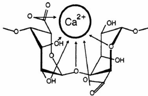
Figure 54 Coordination d'un cation Ca^{2+} avec deux unités d'acides gulonique
