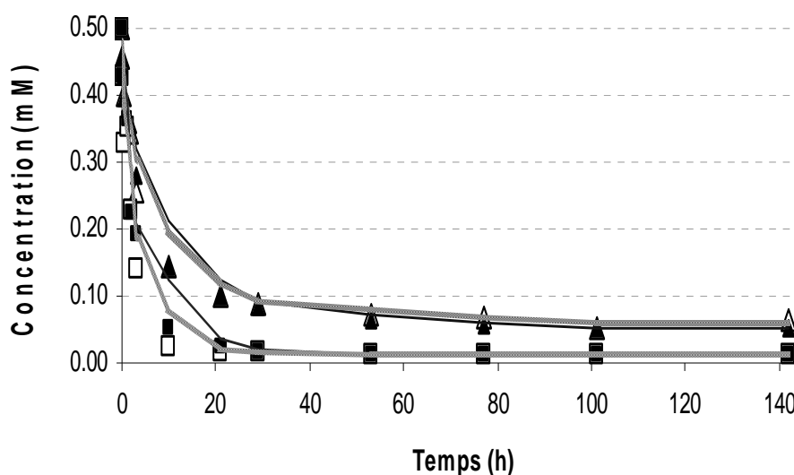
Figure 105 Evolution de la concentration en ABT avec le temps lors de la photobiodégradation de l'ABT (0,5 mM) en présence de FeNTA (1 mM). (Δ) cellules immobilisées + hv ; (▲) cellules immobilisées - hv ; (□) cellules libres + hv ; (■) cellules libres - hv Rq : les valeurs sont brutes et ne prennent pas en considération l'adsorption sur l'alginate
