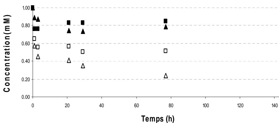
Figure 104 Evolution de la concentration en fer total avec le temps lors de la photodégradation de l'ABT (0,5 mM). (△) billes d'alginate + hv ; (▲) billes d'alginate - hv ; (□) solution + hv ; (■) solution - hv
