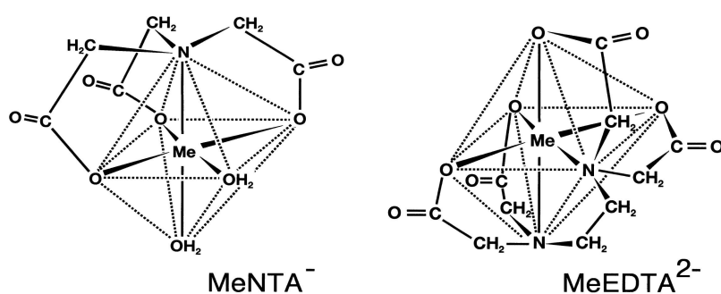
Figure 29 Structures des complexes Métal-NTA et Métal-EDTA
