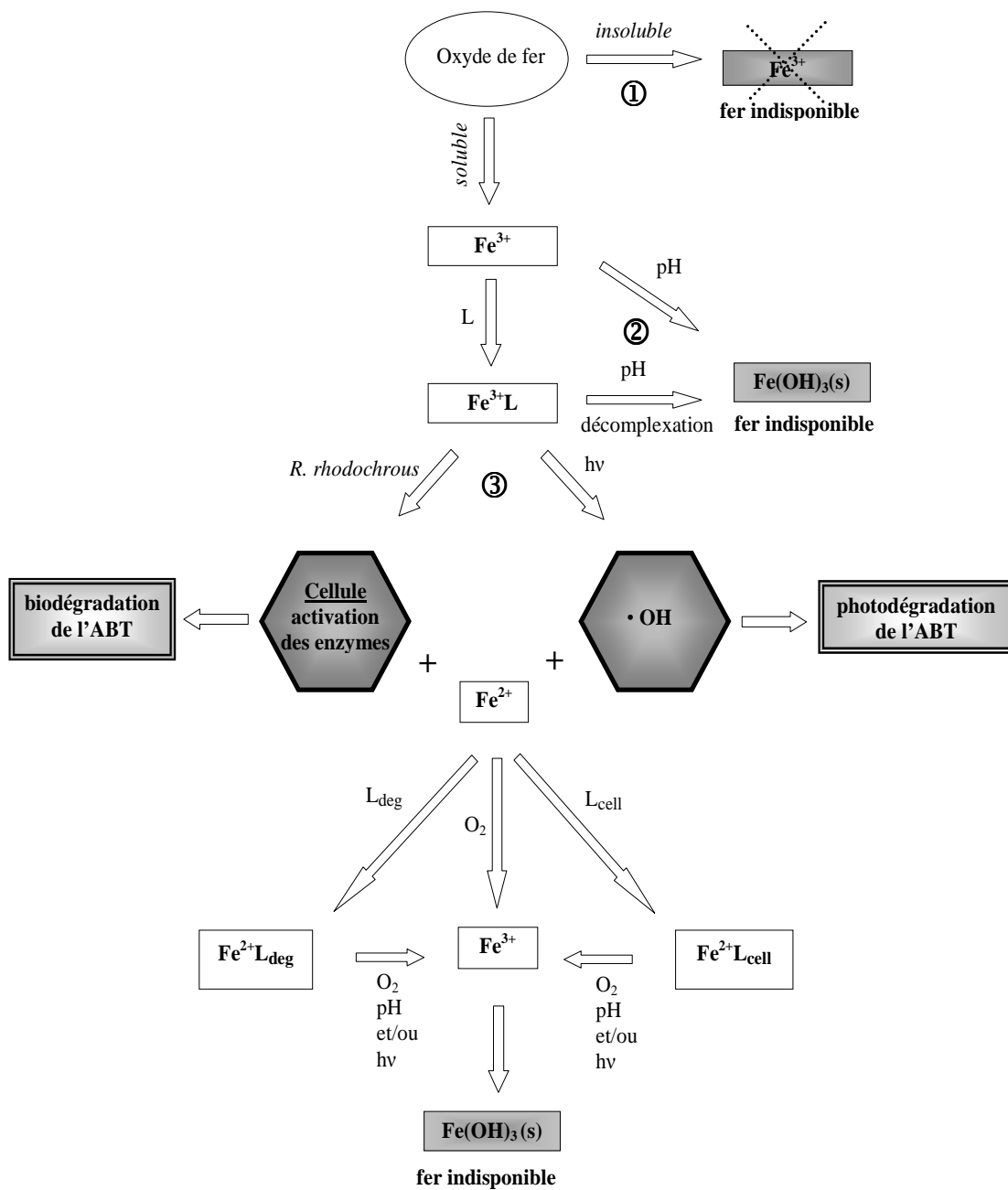
Figure 158 Schéma montrant l'utilisation et le devenir du fer ( L : ligand présent dans le milieu aqueux ; L_{\text{deg}} : ligand issu de la dégradation photochimique ou microbiologique de L ; L_{\text{cell}} : ligand produit par la cellule)
