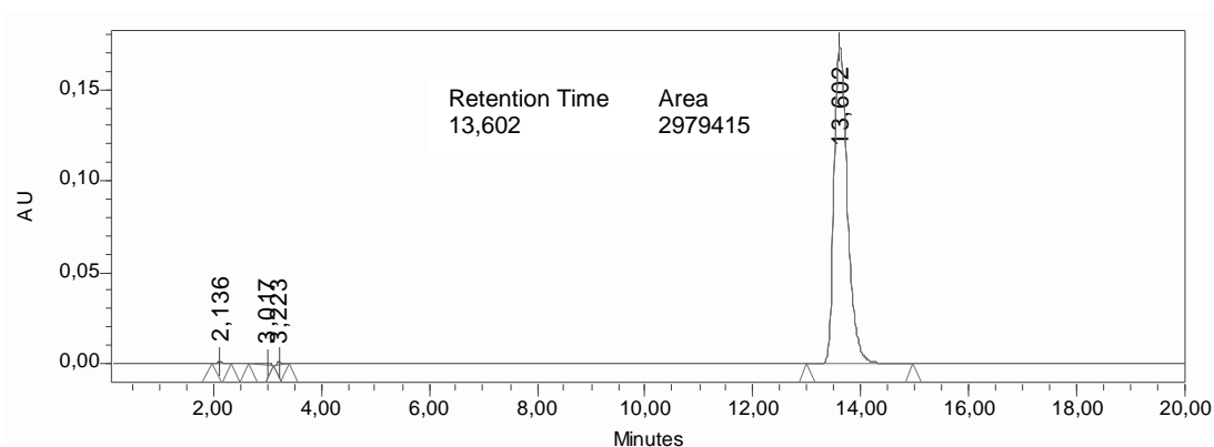
Figure 94 Chromatogramme d'une solution mère d'ABT à 0,5 mM avant SPE
