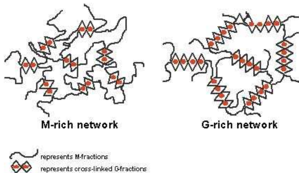
Figure 55 Mécanisme de gélification de l'alginate (site www.genialab.de )
