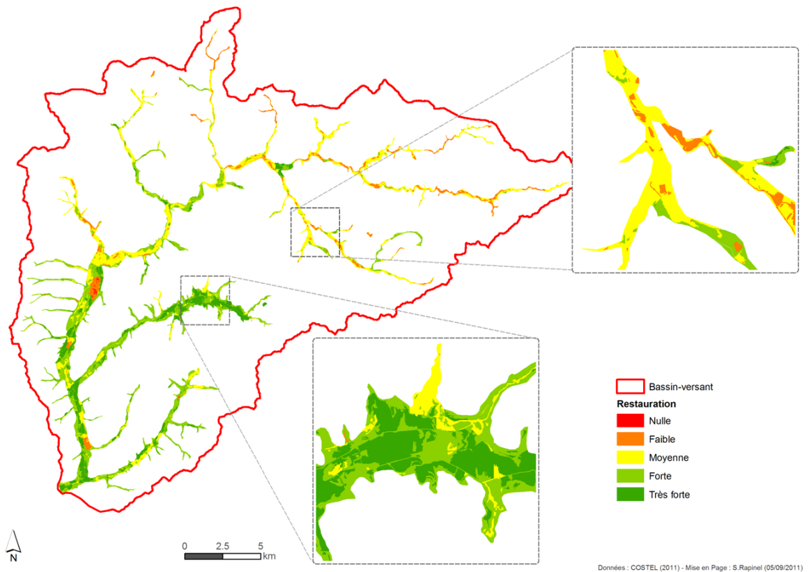
Figure 8.14 – Cartes de vulnérabilité (haut) et de priorité de restauration (bas) pour la fonction dénitrification
