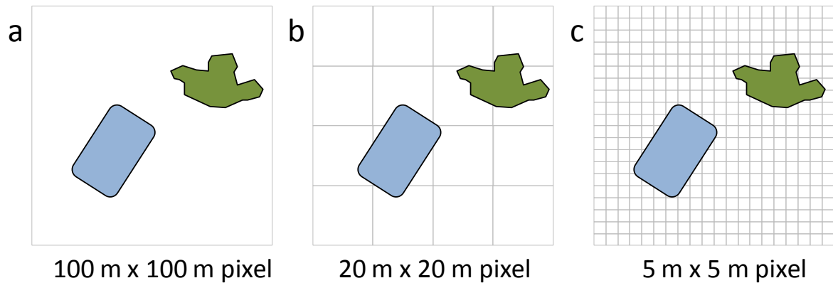
Figure 2.2 – Relations entre les objets et la résolution spatiale : (a) faible résolution : les pixels sont significativement plus grands que les objets, approche par démixage appropriée. (b) résolution moyenne : les pixels et les objets sont de la même taille, approche par pixel appropriée. (c) haute résolution : les pixels sont plus petits que les objets, approche basée-objet appropriée (adapté de Blaschke, 2010).
